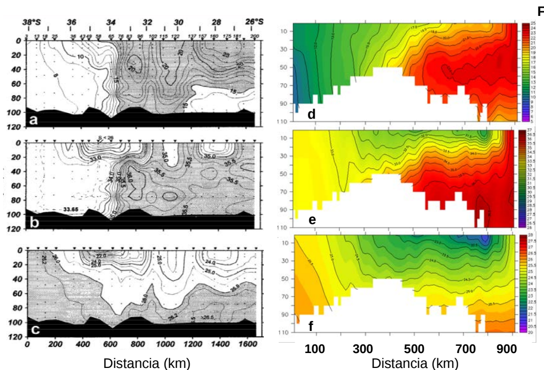
figura 32: Cortes a lo largo de las transectas sinóptico de junio en Piola et al (2000): temperatura (a), salinidad (b), densidad (c); y para el mes de junio en ROMS: temperatura (d), salinidad (e) y densidad (f).
