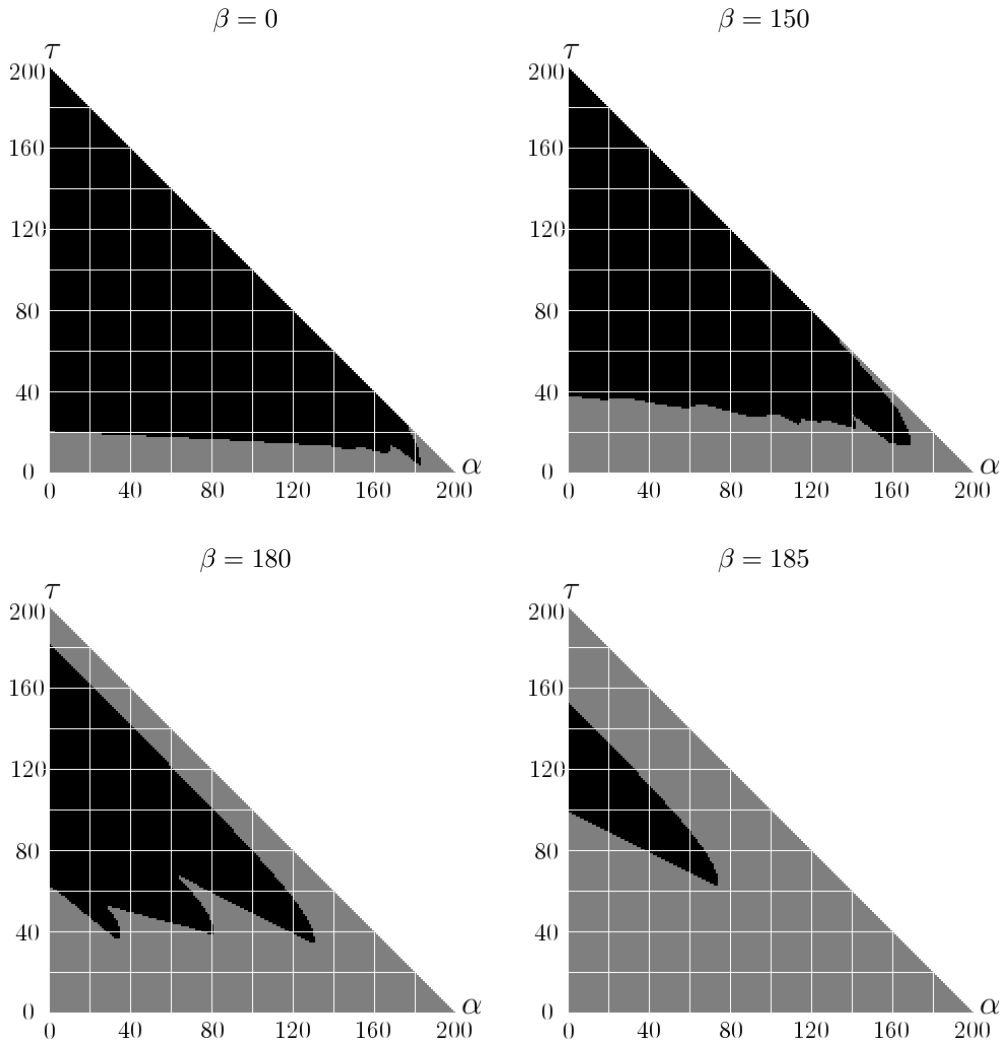
Figura 4.2: Parte de la estrategia óptima, para puntaje del contrincante = 0,150,180 y 185. En la zona gris se debe tirar y en la zona negra parar
