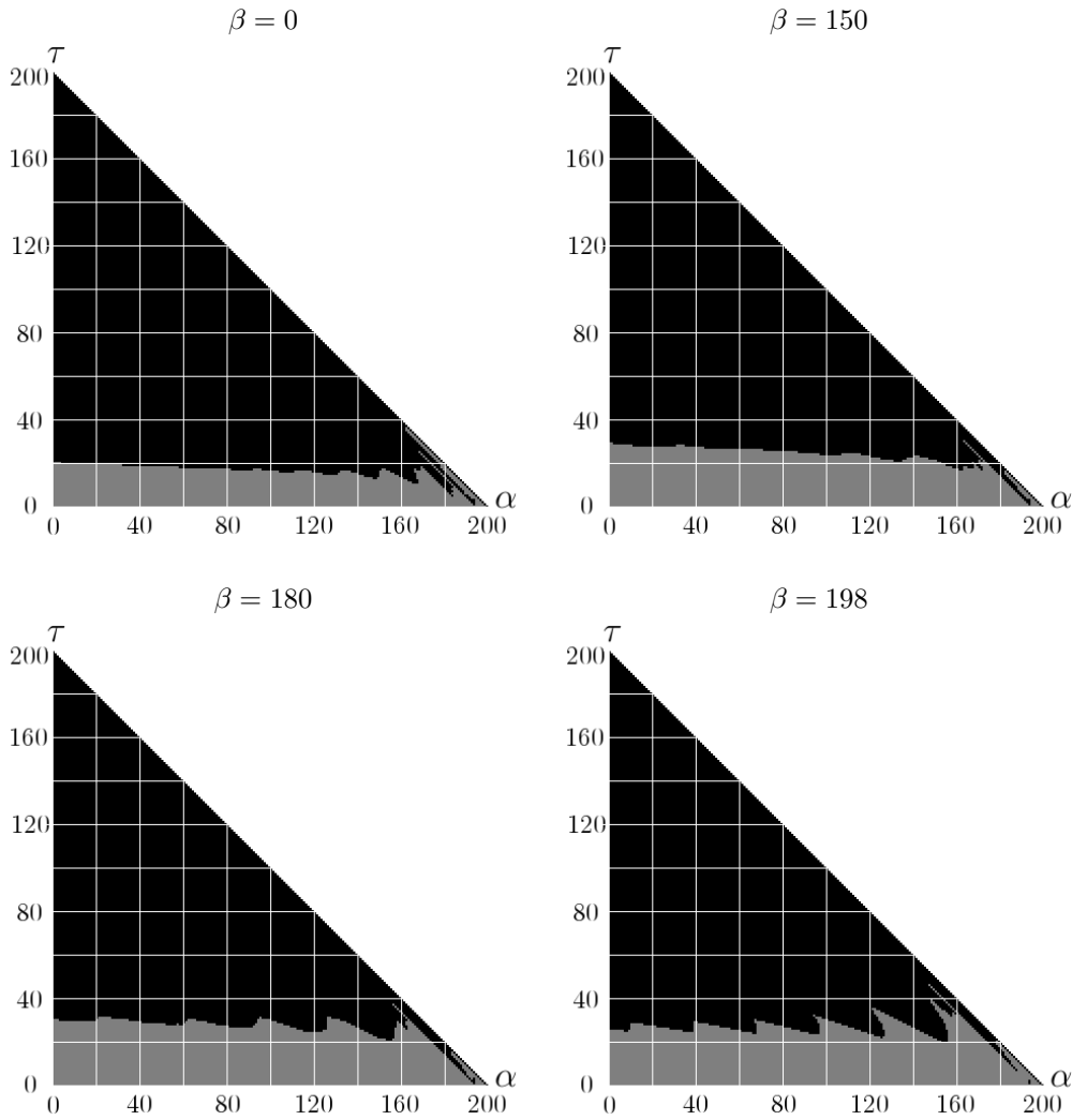
Figura 4.3: Parte de la estrategia óptima para el modelo con rebote, para puntaje del contrincante = 0,150,180 y 198. En la zona gris se debe tirar y en la zona negra parar
