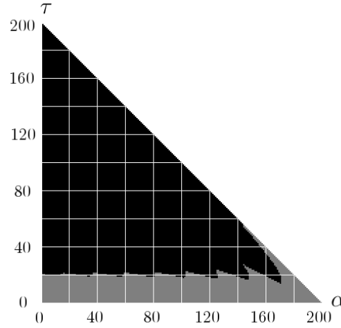
Figura 4.1: Estrategia solitaria que minimiza el valor esperado de la cantidad de turnos. En la zona gris se debe tirar , mientras que en la zona negra se debe parar
