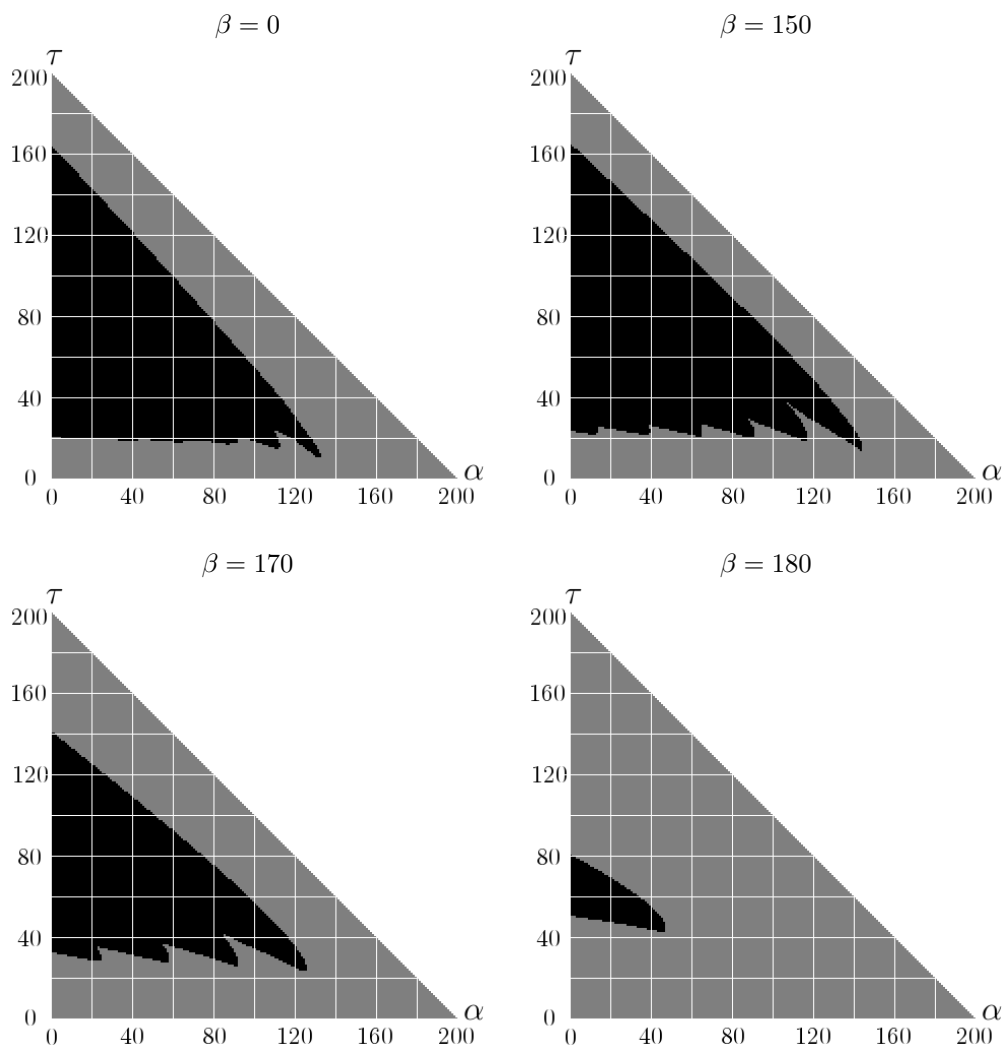
Figura 4.4: Parte de la estrategia óptima cuando se quiere maximizar la diferencia de puntaje, para puntaje del contrincante = 0,150,170 y 180. En la zona gris se debe tirar y en la zona negra parar
