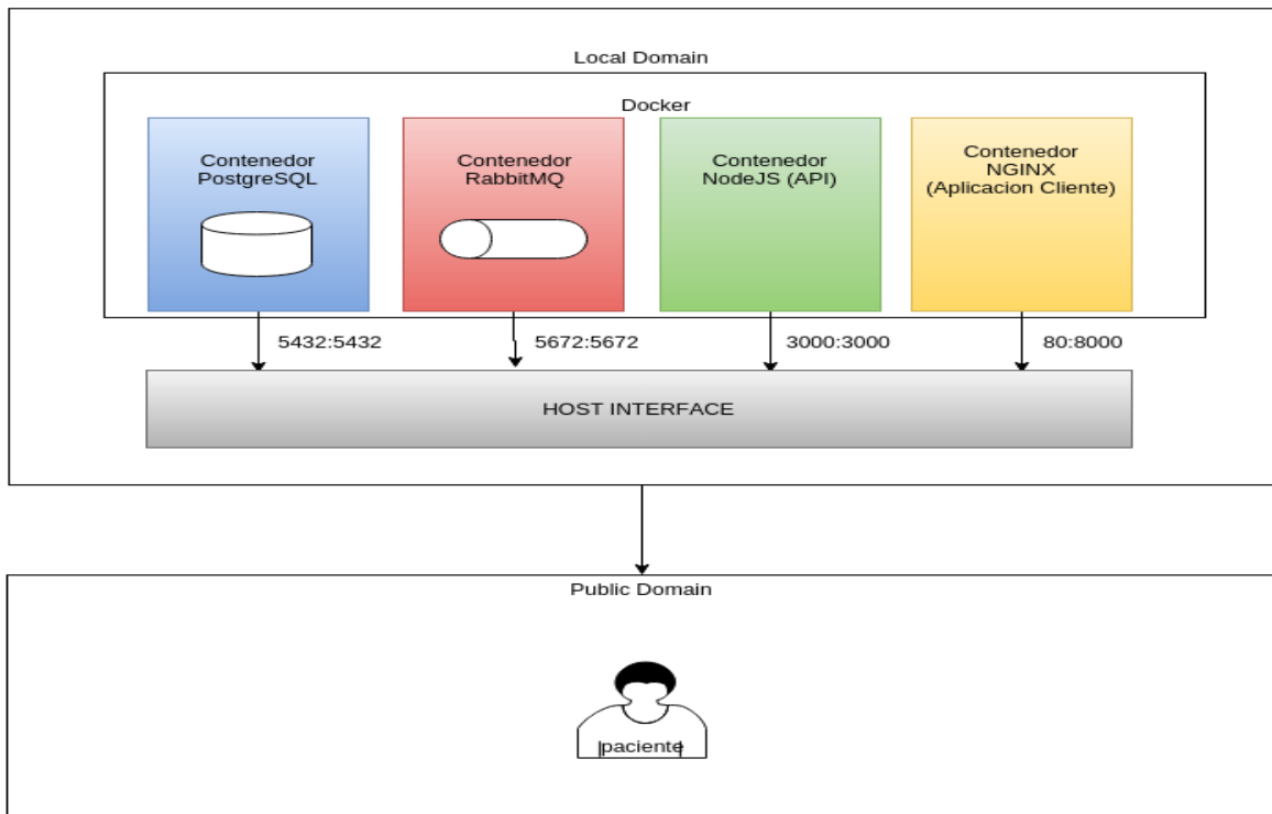
Figura AA2 – Docker orquestador principal de servicios brindados por SAREM
