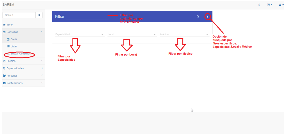
Figura 12 – Filtros para Búsqueda de Consultas.
