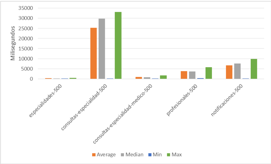
Figura P4 – Contexto Local: 1000 Peticiones, Nivel de concurrencia 500.
