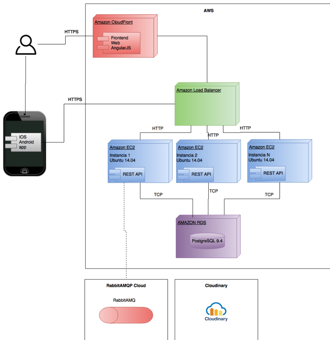
Figura A6 – Diagrama de Despliegue.
