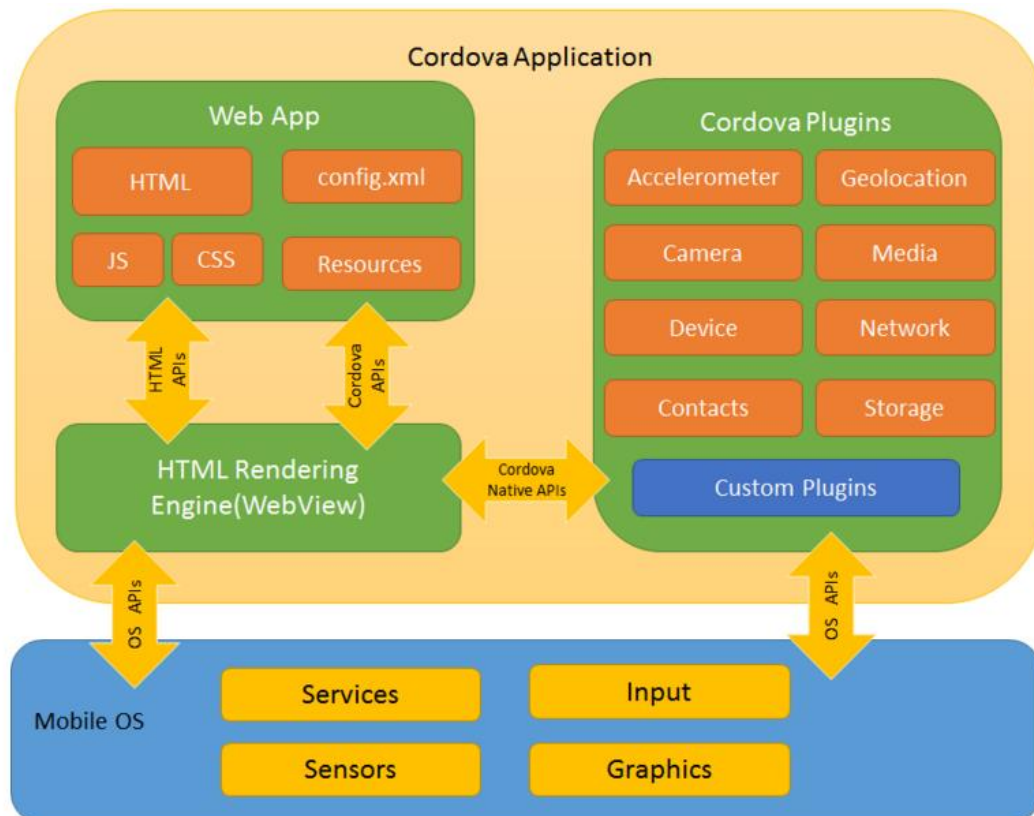
Figura A4 – Arquitectura Apache Cordova.
