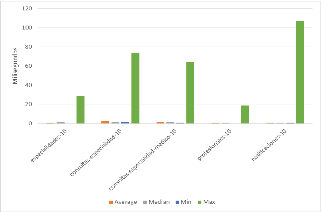
Figura P6 – Contexto Local-NGINX: 1000 Peticiones, Nivel de concurrencia 10.
