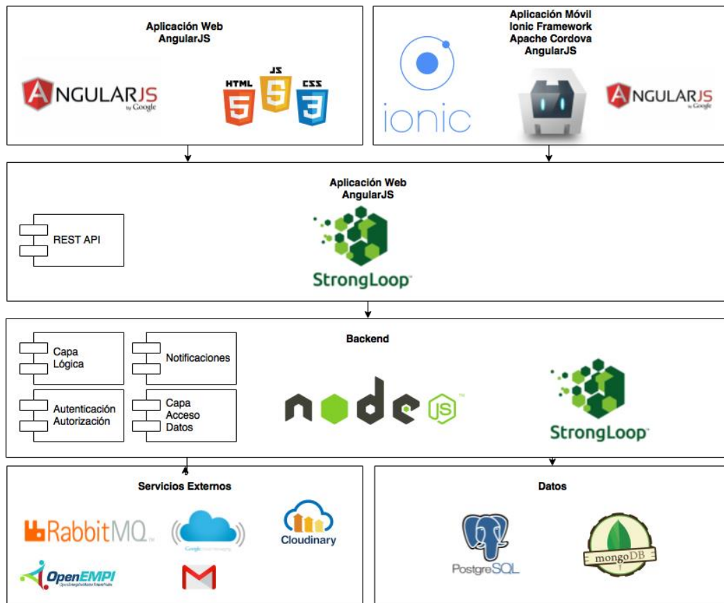
Figura A3 – Enfoque Top-Down de los componentes de SAREM.
