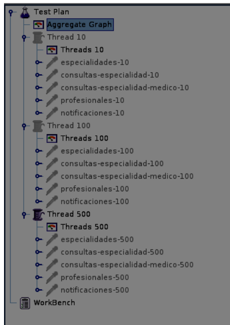
Figura P1 – Captura de cómo se define el conjunto de pruebas de stress para lograr el entorno de configuración.
