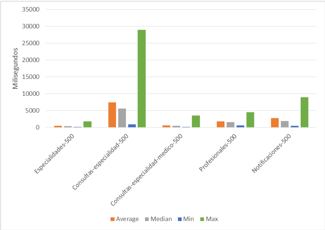
Figura P11 – Contexto Remoto: 1000 Peticiones, Nivel de concurrencia 500.
