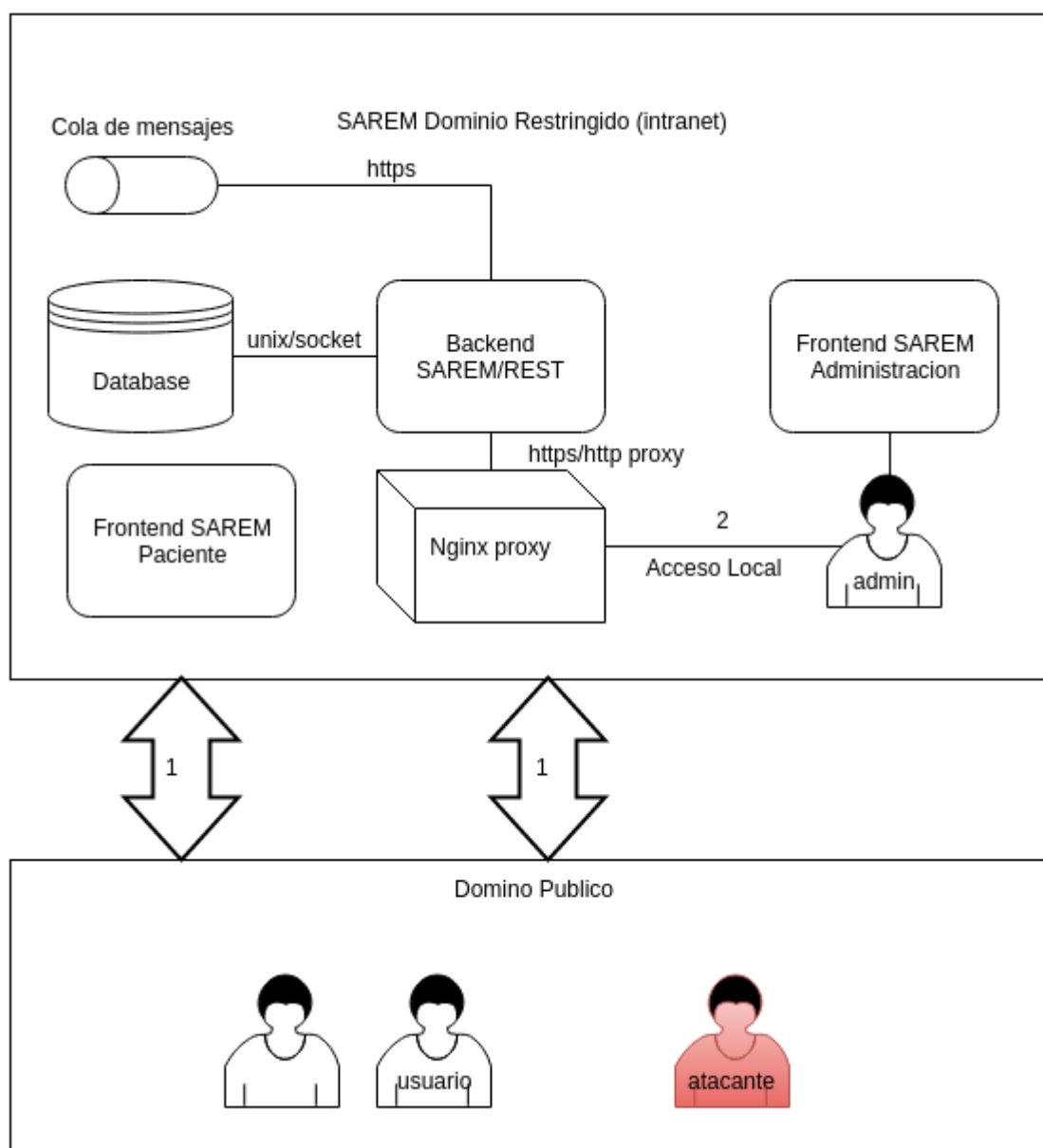
Figura AA1 – Dominios Restringidos
