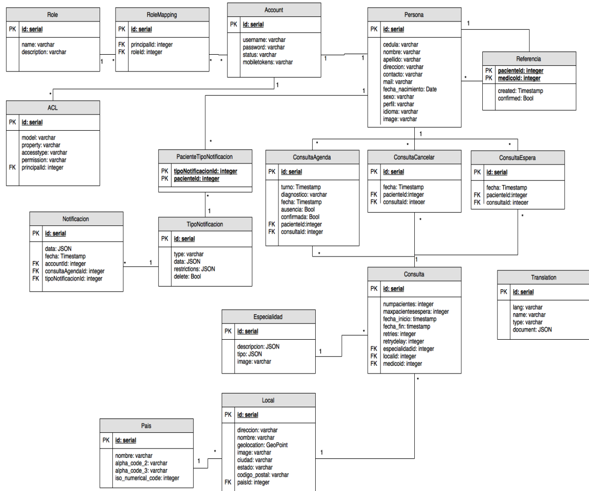
Figura A5 – Modelo de Datos.
