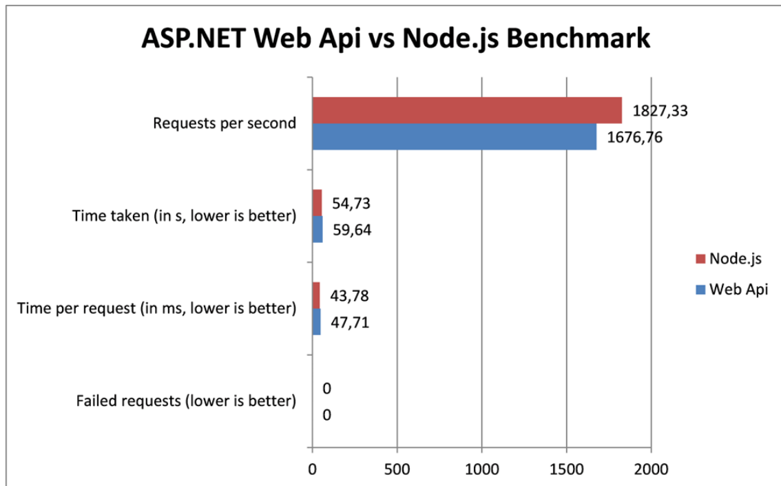
Figura I3 – ASP.NET Web API y Node.js para leer de forma asíncrona el cuerpo de una petición POST.
