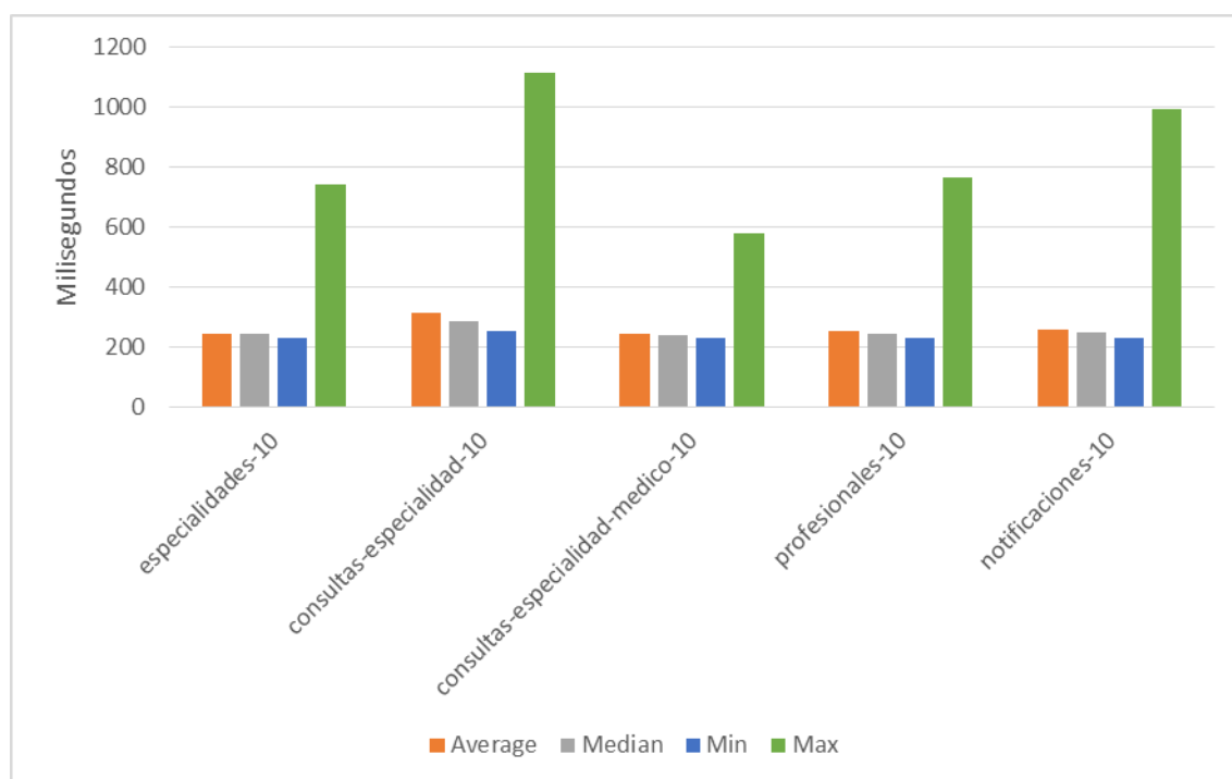
Figura P9 – Contexto Remoto: 1000 Peticiones, Nivel de concurrencia 10.
