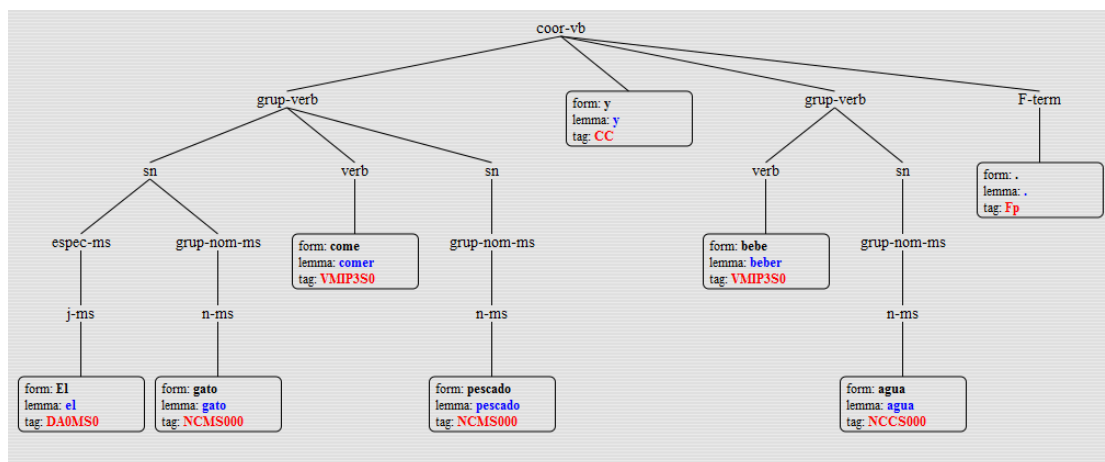
FIGURA A.6: Árbol de parsing de una oración
