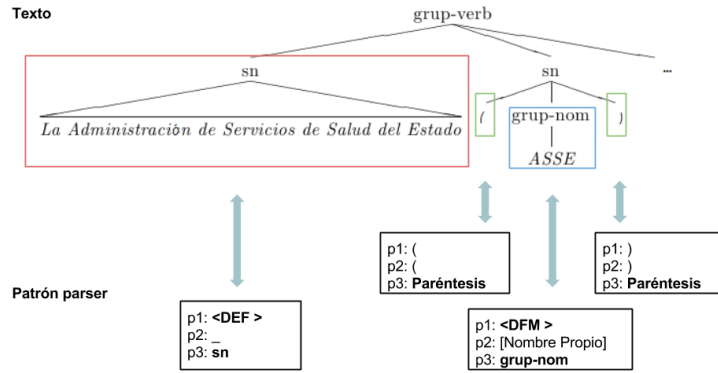
FIGURA 4.9: Correspondencia entre el texto y el patrón parser
