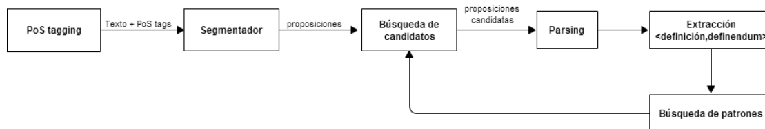
FIGURA 4.1: Diseño del módulo de extracción
