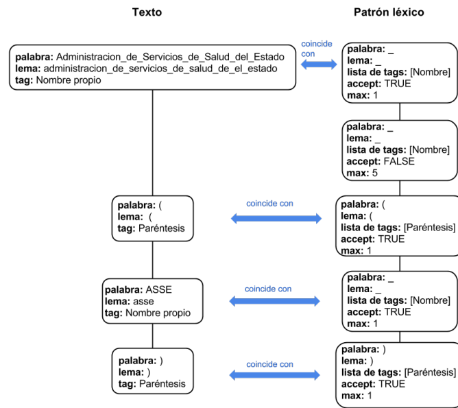
FIGURA 4.8: Correspondencia entre el texto y el patrón léxico
