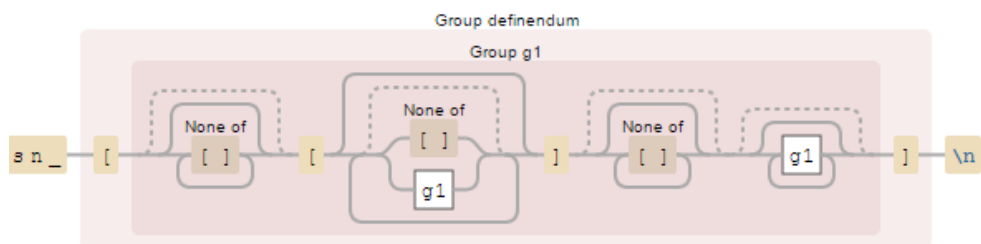
FIGURA B.1: PCRE: Representación gráfica del grupo definendum
