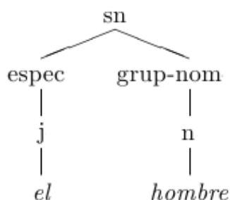
FIGURA B.2: PCRE: Árbol de parsing de “ El hombre ”
