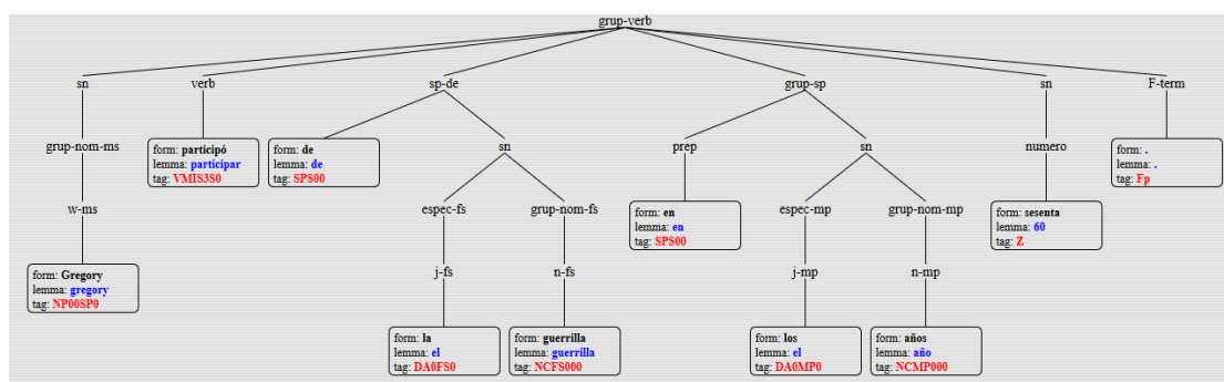
FIGURA 6.4: Ejemplo de parsing incorrecto
