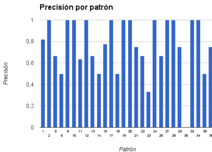
FIGURA 7.2: Corpus 180: Precisión por patrón mejorada
