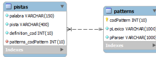
FIGURA 6.2: Esquema de la base de datos.
