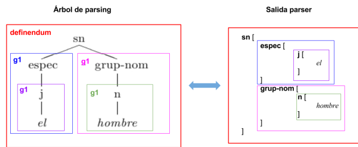
FIGURA B.3: PCRE: Correspondencia entre el árbol y la salida del parser
