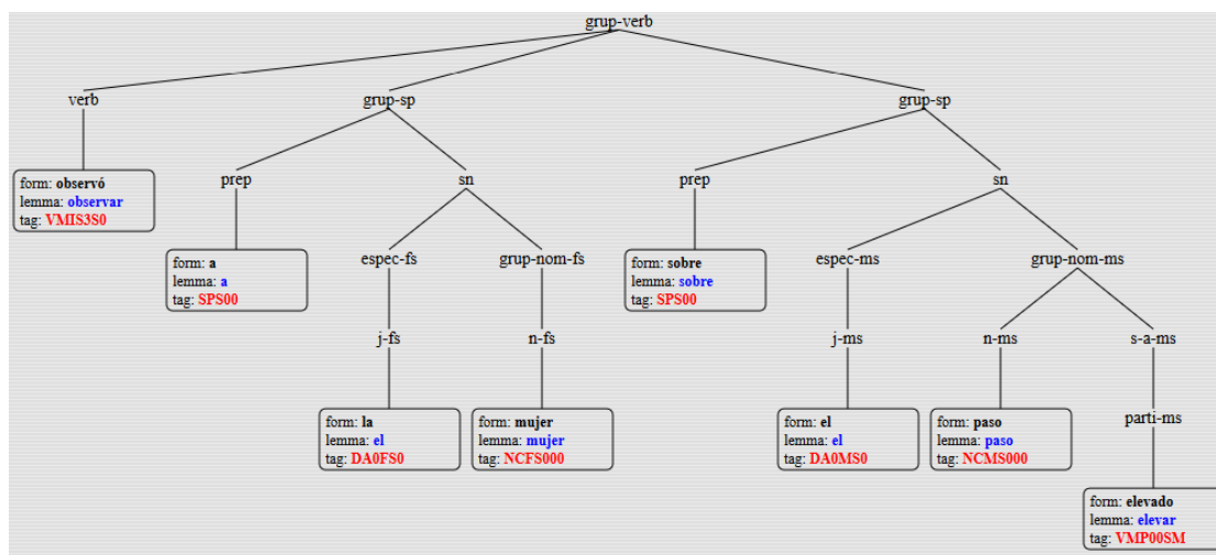
FIGURA 6.3: Ejemplo de parsing incorrecto
