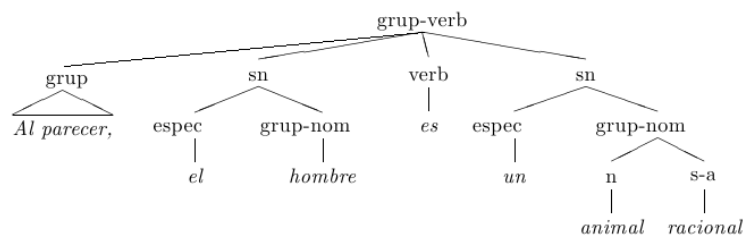
FIGURA 4.6: Árbol de parsing completo: “El hombre es un animal racional”
