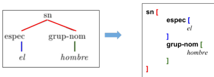
FIGURA 4.7: Ejemplo de salida del parser
