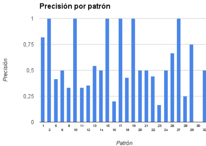
FIGURA 7.1: Corpus 180: Precisión por patrón inicial
