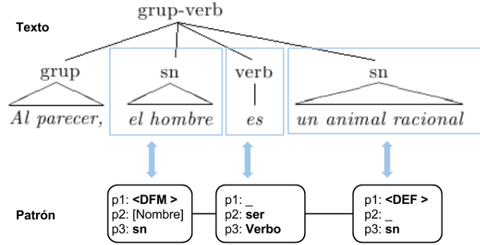
FIGURA 4.4: Correspondencia entre el texto y el patrón parser .
