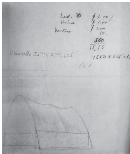
Boceto con bóvedas autoportantes de Dieste y algún arquitecto colaborador, 1954. Archivo de la Parroquia del Sagrado Corazón de Jesús, Atlántida.
