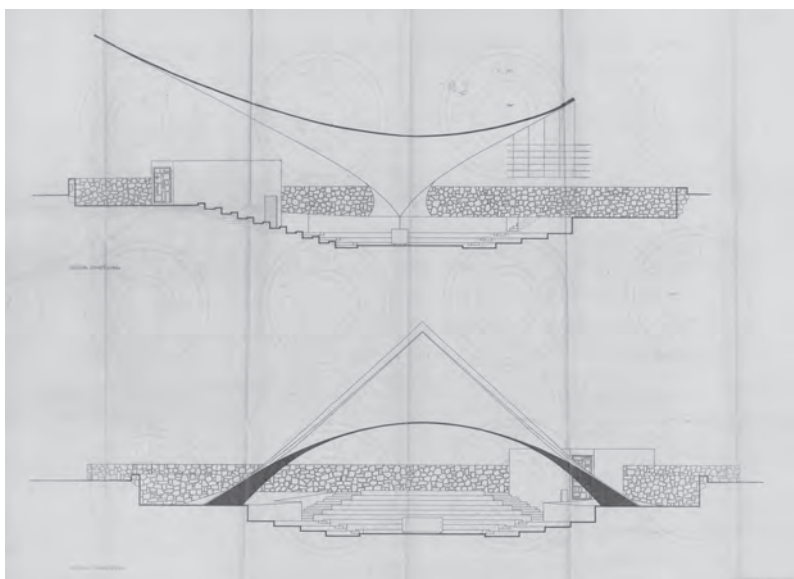
Nuestra Señora del Mar, Port Salou, 1961. Planta y cortes. COAC. Arxiu Històric d'Arquitectura de Barcelona. Fondo Bonet.
