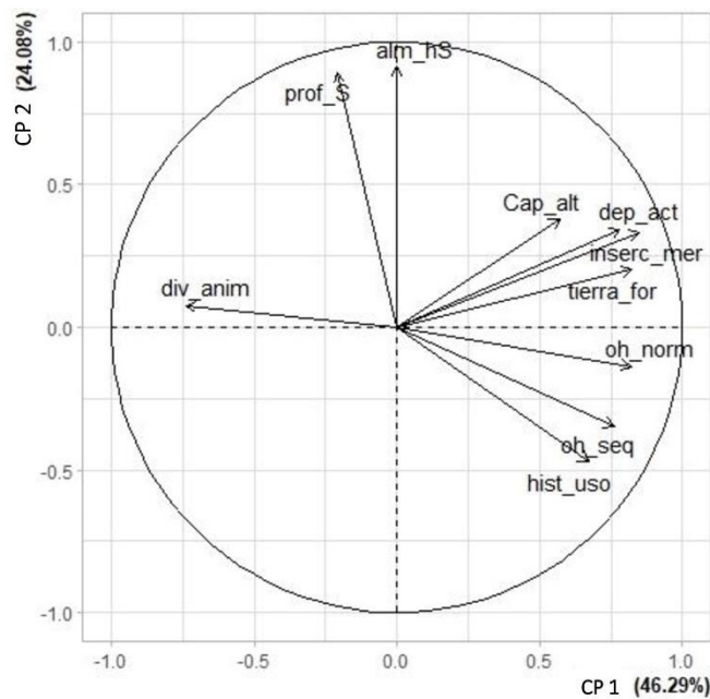
Figura 3.5 Relación entre las variables explicativas de la vulnerabilidad a la sequía y los dos primeros Componentes Principales. Almacenamiento de agua en el suelo: alm_hS; profundidad del suelo: prof_$; inserción en el mercado: inserc_mer; dependencia económica: dep_act; disponibilidad de tierra para producción vegetal: tierra_for; disponibilidad hídrica sin sequía: oh_norm; disponibilidad hídrica durante sequías: oh_seq; diversidad de especies animales: div_anim; intensidad de usos del suelo previos: hist_uso; capacidad de reducir daño de las sequías: Cap_alt.
