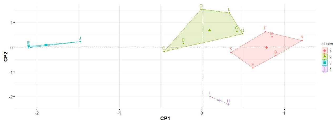
Figura 3.8 Grupos de productores/as según di/similitud de valores de Componentes Principales.
