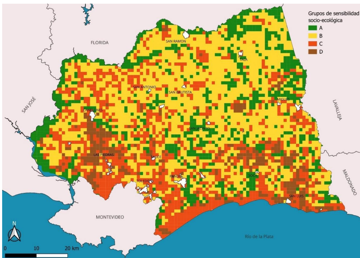
Figura 2.5 Agrupamiento de celdas según niveles de sensibilidad socio-ecológica durante las sequías registradas entre enero de 2015 y mayo de 2022.
