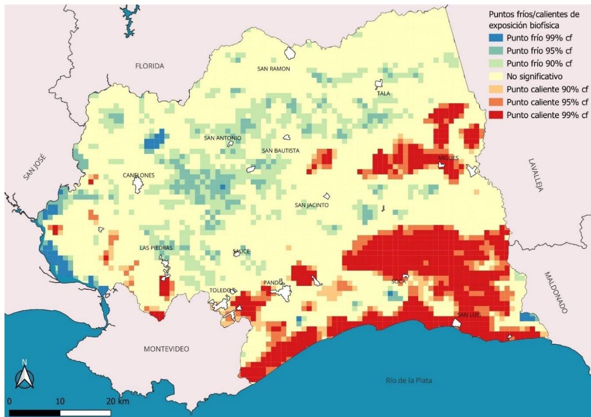
Figura 2.3 Puntos calientes/fríos de exposición biofísica a la sequía en Canelones con confianza (cf) estadística.
