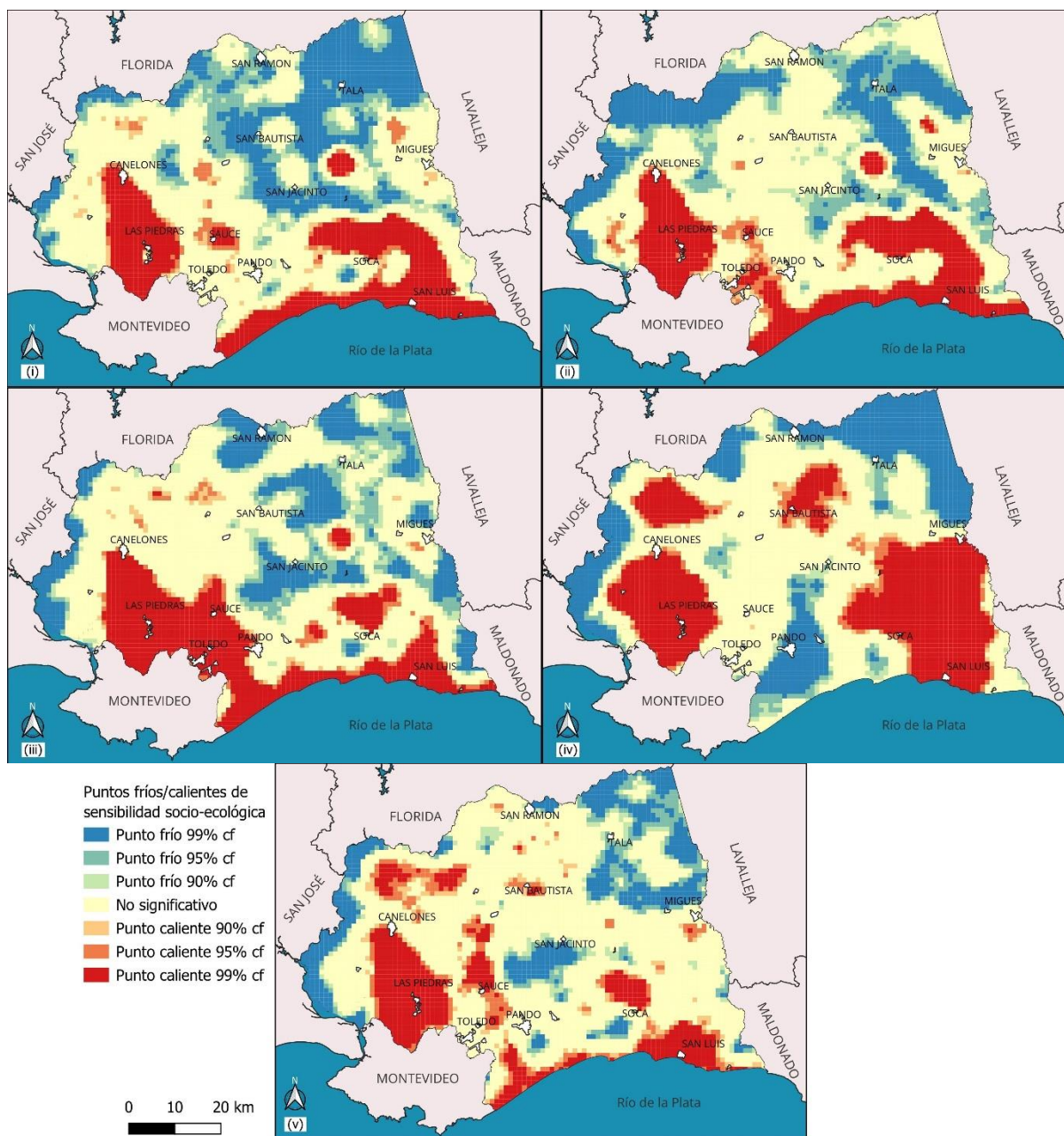
Figura 2.4 Puntos calientes/fríos de sensibilidad socio-ecológica a la sequía en Canelones con confianza estadística (cf) durante los cinco eventos de sequía (i-v) registrados entre enero de 2015 y mayo de 2022. Evento (i): de abril a julio de 2015; Evento (ii) en setiembre de 2015; evento (iii) de febrero a mayo de 2020; evento (iv) de noviembre a diciembre de 2020; evento (v) en octubre de 2021.
