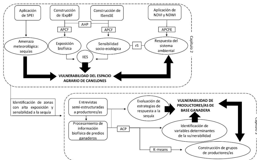
Figura 1.1 Estrategia general de investigación. SPEI: Standarized Precipitation Evapotranspiration Index, IexpBF: Índice de Exposición Biofísica, Índice de Sensibilidad Socio-Ecológica: ISensSE, Índice Integrado de Exposición y Sensibilidad: IIES, Normalized Difference Vegetation Index: NDVI, Normalized Difference Water Index: NDWI, Análisis Jerárquico Ponderado: AHP, Análisis de Puntos Calientes/Fríos: APCF, Análisis de Puntos Calientes/Fríos Emergentes: APCFE, correlación de Spearman: rS, Análisis de Componentes Principales: ACP y análisis clúster método K-means: K-means.
