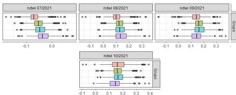
Figura 2.20 Diagrama de cajas del NDWI por grupos de sensibilidad socio-ecológica para los tres meses previos (arriba) y durante el evento (abajo) de sequía (v). En color rosado: Grupo A; en verde: Grupo B; en celeste: Grupo C; y en violeta: Grupo D.
