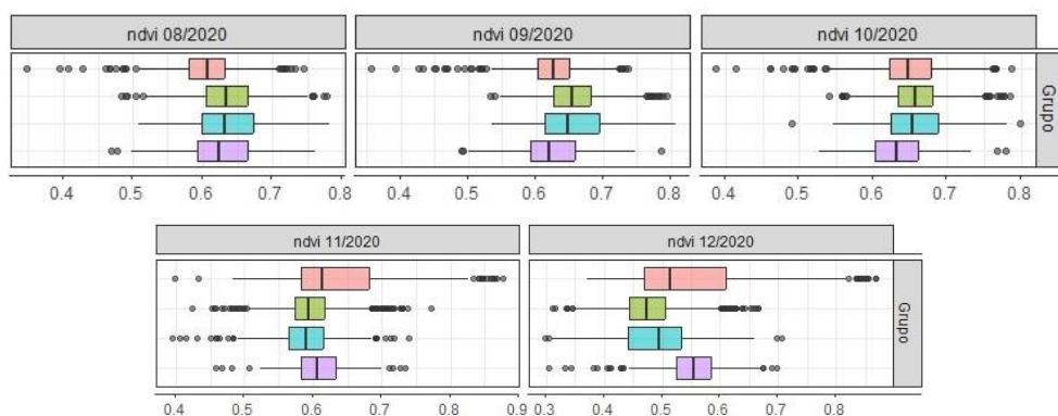
Figura 2.17 Diagrama de cajas del NDVI por grupos de sensibilidad socio-ecológica para los tres meses previos (arriba) y durante el evento (abajo) de sequía (iv). En color rosado: Grupo A; en verde: Grupo B; en celeste: Grupo C; y en violeta: Grupo D.
