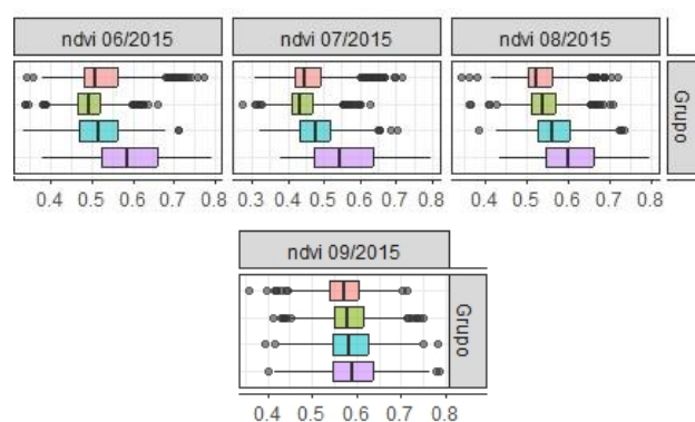
Figura 2.13 Diagrama de cajas del NDVI por grupos de sensibilidad socio-ecológica para los tres meses previos (arriba) y durante el evento (abajo) de sequía (ii). En color rosado: Grupo A; en verde: Grupo B; en celeste: Grupo C; y en violeta: Grupo D.
