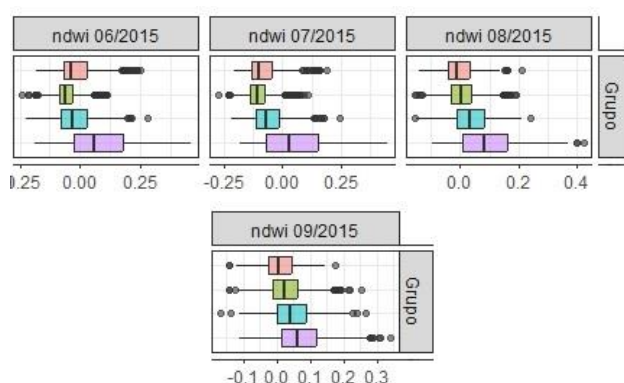
Figura 2.14 Diagrama de cajas del NDWI por grupos de sensibilidad socio-ecológica para los tres meses previos (arriba) y durante el evento (abajo) de sequía (ii). En color rosado: Grupo A; en verde: Grupo B; en celeste: Grupo C; y en violeta: Grupo D.
