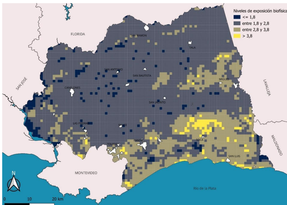
Figura 2.1 Distribución espacial de la exposición biofísica a las sequías en Canelones.
