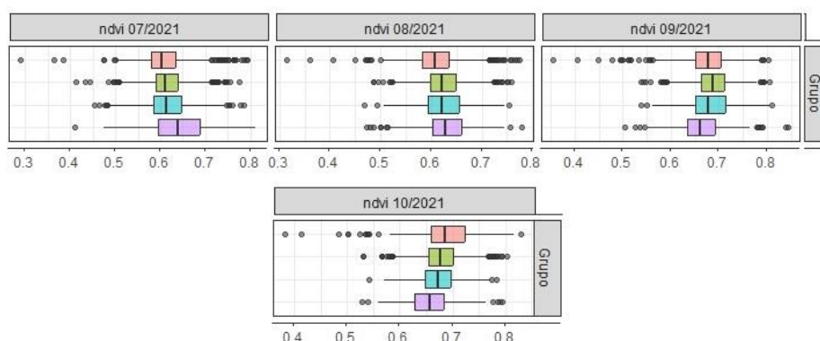
Figura 2.19 Diagrama de cajas del NDVI por grupos de sensibilidad socio-ecológica para los tres meses previos (arriba) y durante el evento (abajo) de sequía (v). En color rosado: Grupo A; en verde: Grupo B; en celeste: Grupo C; y en violeta: Grupo D.
