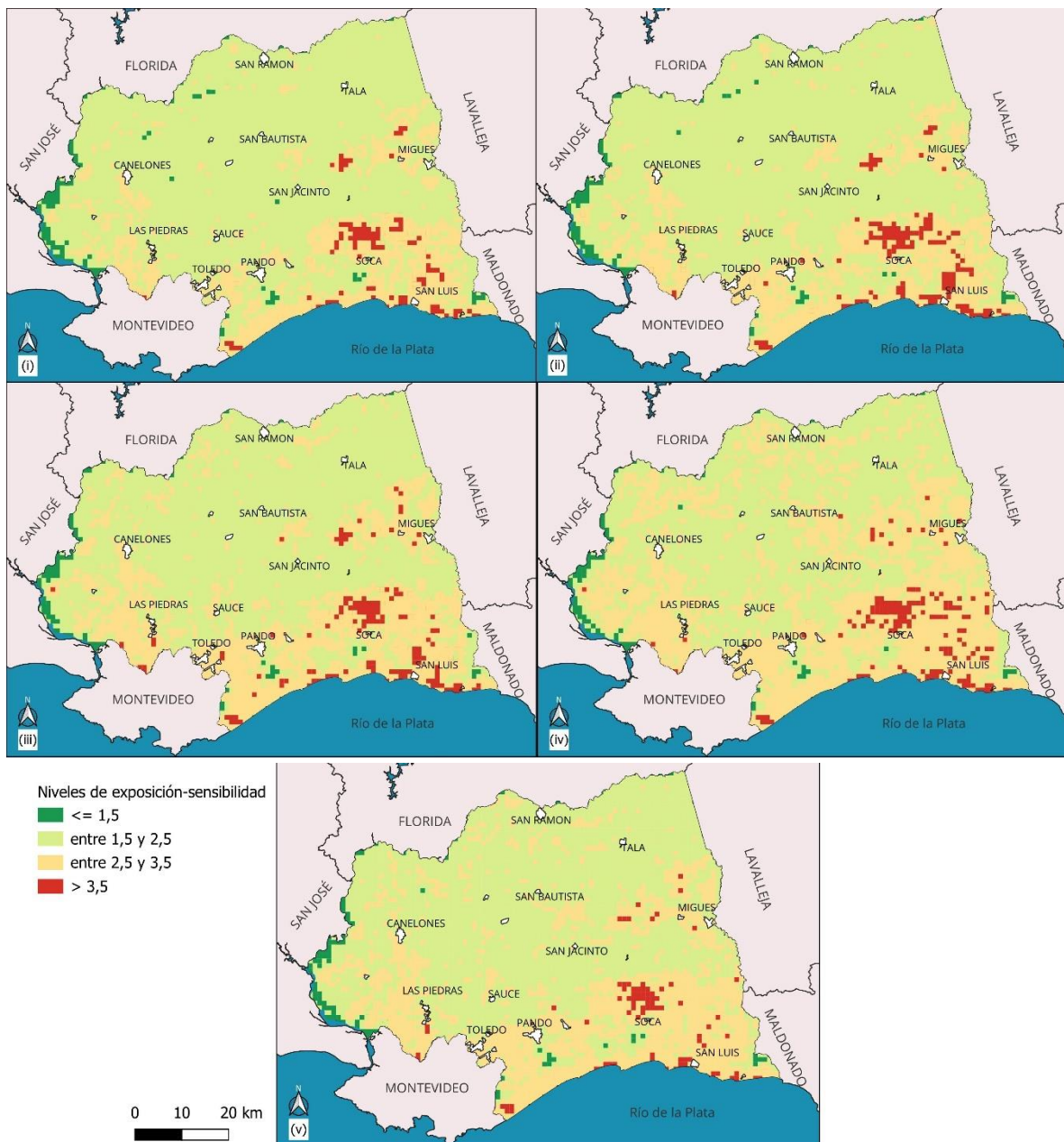
Figura 2.7 Distribución de niveles del índice de exposición-sensibilidad a la sequía durante los cinco eventos de sequía registrados entre enero de 2015 y mayo de 2022. Evento (i): de abril a julio de 2015; Evento (ii) en septiembre de 2015; evento (iii) de febrero a mayo de 2020; evento (iv) de noviembre a diciembre de 2020; evento (v) en octubre de 2021.
