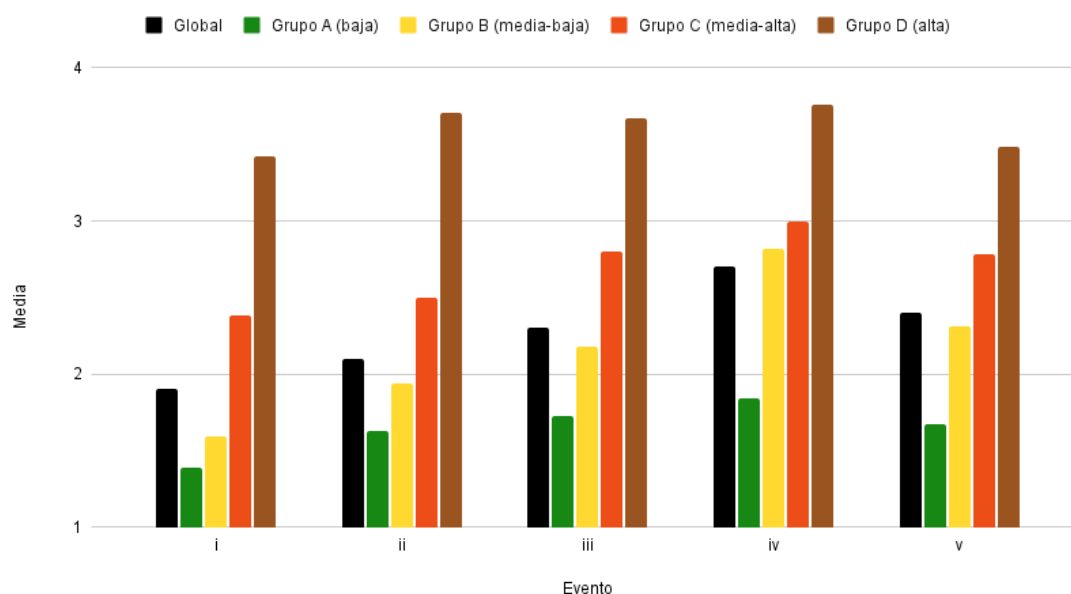
Figura 2.6 Evolución de valores medios de sensibilidad socio-ecológica a la sequía por grupos de sensibilidad para los cinco eventos de sequía registrados entre enero de 2015 y mayo de 2022. Evento (i): de abril a julio de 2015; Evento (ii) en setiembre de 2015; evento (iii) de febrero a mayo de 2020; evento (iv) de noviembre a diciembre de 2020; evento (v) en octubre de 2021.
