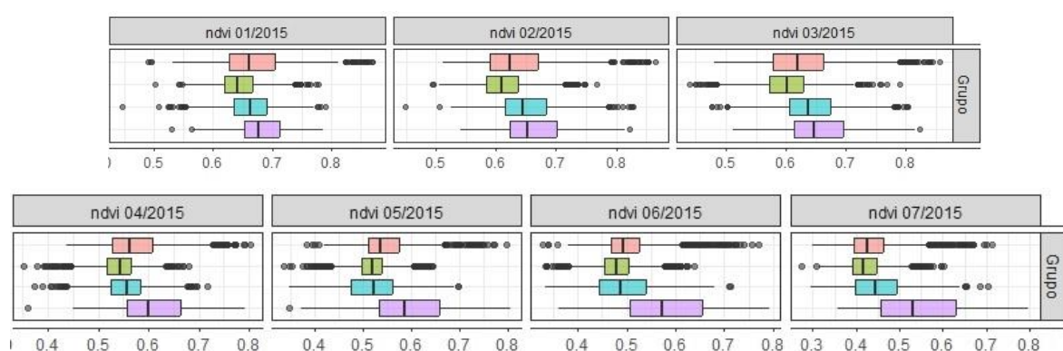
Figura 2.11 Diagrama de cajas del NDVI por grupos de sensibilidad socio-ecológica para los tres meses previos (arriba) y durante el evento (abajo) de sequía (i). En color rosado: Grupo A; en verde: Grupo B; en celeste: Grupo C; y en violeta: Grupo D.
