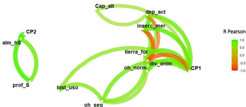
Figura 3.6 Red de correlación Pearson entre las variables explicativas de la vulnerabilidad y los dos primeros Componentes Principales. Almacenamiento de agua en el suelo: alm_hS; profundidad del suelo: prof_S; inserción en el mercado: inserc_mer; dependencia económica: dep_act; disponibilidad de tierra para producción vegetal: tierra_for; disponibilidad hídrica sin sequías: oh_norm; disponibilidad hídrica durante sequías: oh_seq; diversidad de especies animales: div_anim; intensidad de usos del suelo previos: hist_uso; capacidad de reducir daño de las sequías: Cap_alt.
