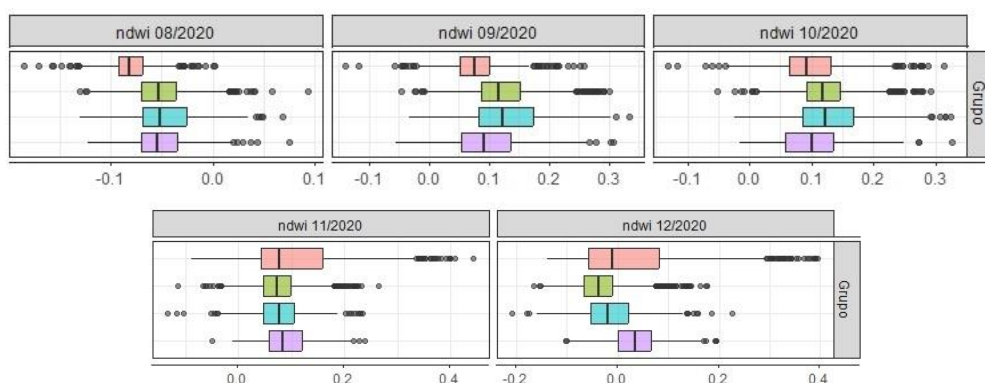
Figura 2.18 Diagrama de cajas del NDWI por grupos de sensibilidad socio-ecológica para los tres meses previos (arriba) y durante el evento (abajo) de sequía (iv). En color rosado: Grupo A; en verde: Grupo B; en celeste: Grupo C; y en violeta: Grupo D.
