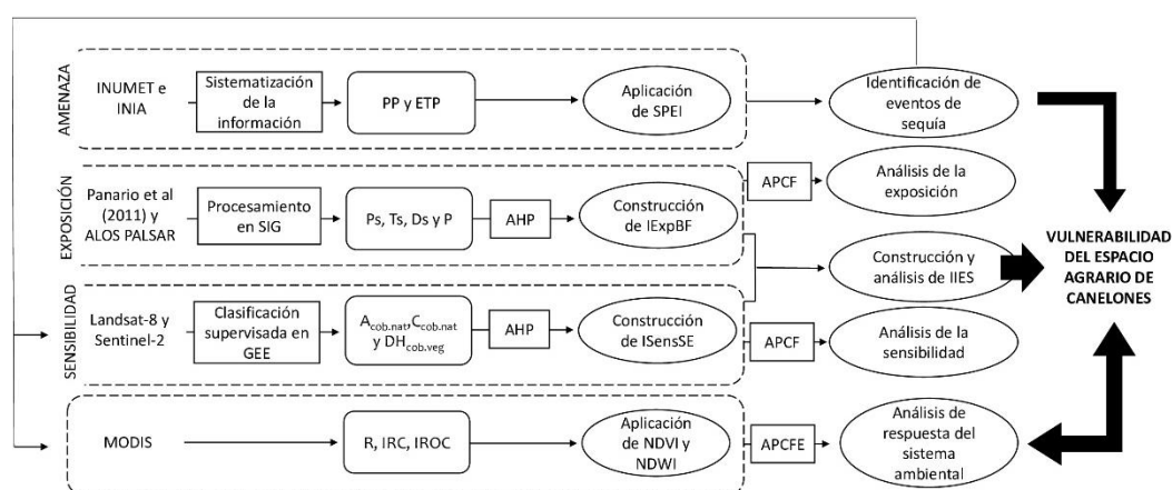
Figura 2.1 Estrategia de investigación del capítulo II. Precipitación: PP, evapotranspiración potencial: ETP, Standardized Precipitation Evapotranspiration Index (SPEI), profundidad del suelo: Ps, textura del suelo: Ts y drenaje del suelo: Ds, pendiente del terreno: P, Análisis Jerárquico Ponderado: AHP, Índice de Exposición Biofísica: IExpBF, Análisis de Puntos Calientes/Fríos: APCF, área ocupada por vegetación natural: Acob.nat, conectividad de la cobertura vegetal natural: Ccob.nat, demanda hídrica de la vegetación: DHcob.veg, Índice de Sensibilidad Socio-Ecológica: ISensSE, Índice Integrado de Exposición y Sensibilidad: IIES, reflectancia de las bandas espectrales del Rojo: R, Infrarrojo Cercano: IRC e Infrarrojo de Onda Corta: IROC, Normalized Difference Vegetation Index: NDVI, Normalized Difference Water Index: NDWI, Análisis de Puntos Calientes/Fríos Emergentes (PCFE).
