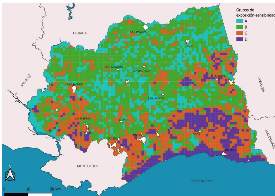
Figura 2.9 Agrupamiento de celdas de 1x1km según similitud en valores del IIES.
