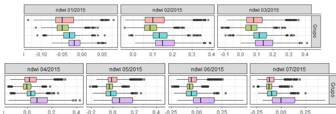
Figura 2.12 Diagrama de cajas del NDWI por grupos de sensibilidad socio-ecológica para los tres meses previos (arriba) y durante el evento (abajo) de sequía (i). En color rosado: Grupo A; en verde: Grupo B; en celeste: Grupo C; y en violeta: Grupo D.
