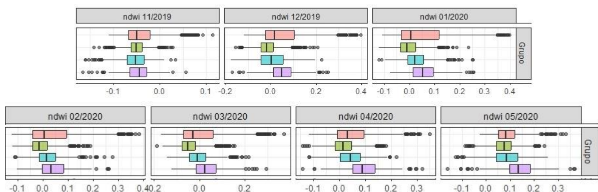
Figura 2.16 Diagrama de cajas del NDWI por grupos de sensibilidad socio-ecológica para los tres meses previos (arriba) y durante el evento (abajo) de sequía (iii). En color rosado: Grupo A; en verde: Grupo B; en celeste: Grupo C; y en violeta: Grupo D.
