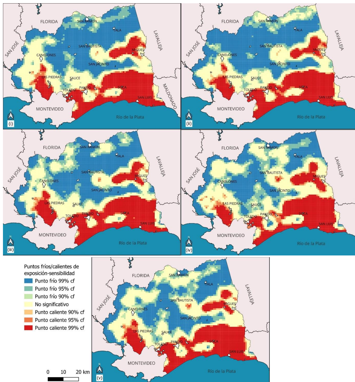
Figura 2.8 Puntos calientes/fríos del IIES en Canelones con confianza (cf) estadística durante los cinco eventos de sequía registrados entre enero de 2015 y mayo de 2022. Evento (i): de abril a julio de 2015; Evento (ii) en setiembre de 2015; evento (iii) de febrero a mayo de 2020; evento (iv) de noviembre a diciembre de 2020; evento (v) en octubre de 2021.
