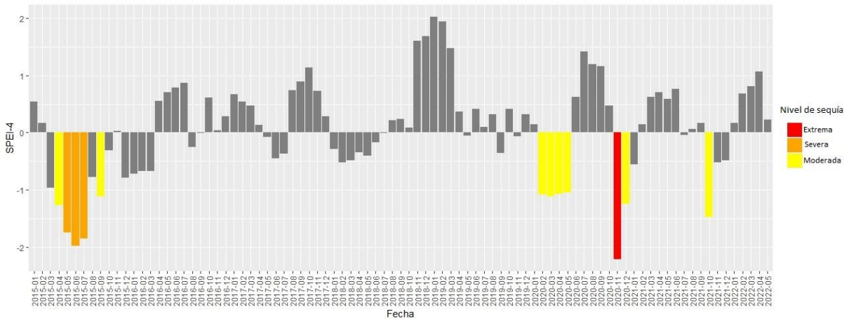
Figura 2.1 Evolución mensual de SPEI-4 meses en Canelones entre enero de 2015 y mayo de 2022.
