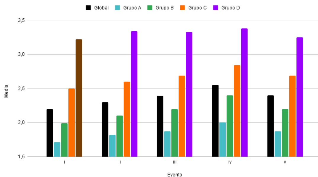
Figura 2.10 Evolución de valores medios del IIES por grupos de exposición-sensibilidad a la sequía. Evento (i): de abril a julio de 2015; Evento (ii) en setiembre de 2015; evento (iii) de febrero a mayo de 2020; evento (iv) de noviembre a diciembre de 2020; evento (v) en octubre de 2021.
