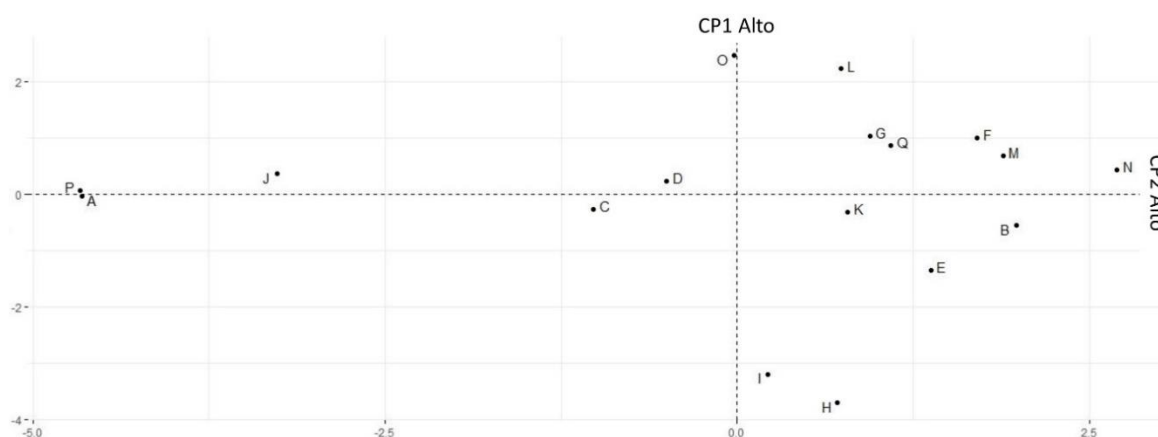
Figura 3.7 Posición de los/as productores/as (indicados con letras) de base ganadera respecto a los valores de los Componentes Principales 1 y 2. El cuadrante inferior del eje vertical y el izquierdo del eje horizontal se vinculan a una alta vulnerabilidad biofísica y económico-productiva, respectivamente.
