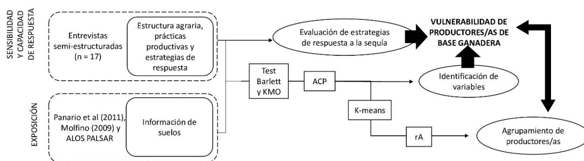
Figura 3.3 Estrategia de investigación del capítulo III. Criterio Kaiser-Meyer-Olkin: KMO, Análisis de Componentes Principales: ACP, análisis clúster método K-means: K-means, test ANOSIM: rA.
