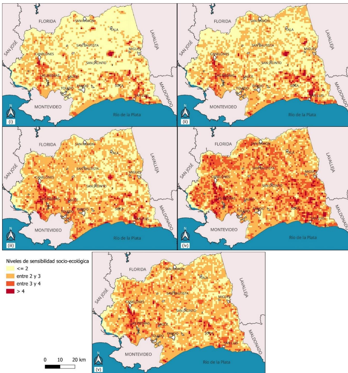
Figura 2.2 Distribución espacial de los niveles de sensibilidad socio-ecológica a la sequía en Canelones para cada uno de los cinco eventos de sequía identificados entre enero de 2015 y mayo de 2022. Evento (i): de abril a julio de 2015; Evento (ii) en setiembre de 2015; evento (iii) de febrero a mayo de 2020; evento (iv) de noviembre a diciembre de 2020; evento (v) en octubre de 2021.
