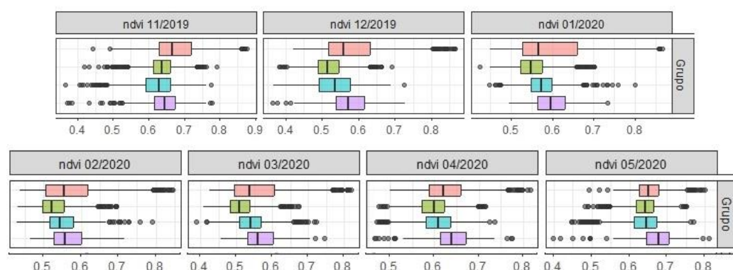
Figura 2.15 Diagrama de cajas del NDVI por grupos de sensibilidad socio-ecológica para los tres meses previos (arriba) y durante el evento (abajo) de sequía (iii). En color rosado: Grupo A; en verde: Grupo B; en celeste: Grupo C; y en violeta: Grupo D.
