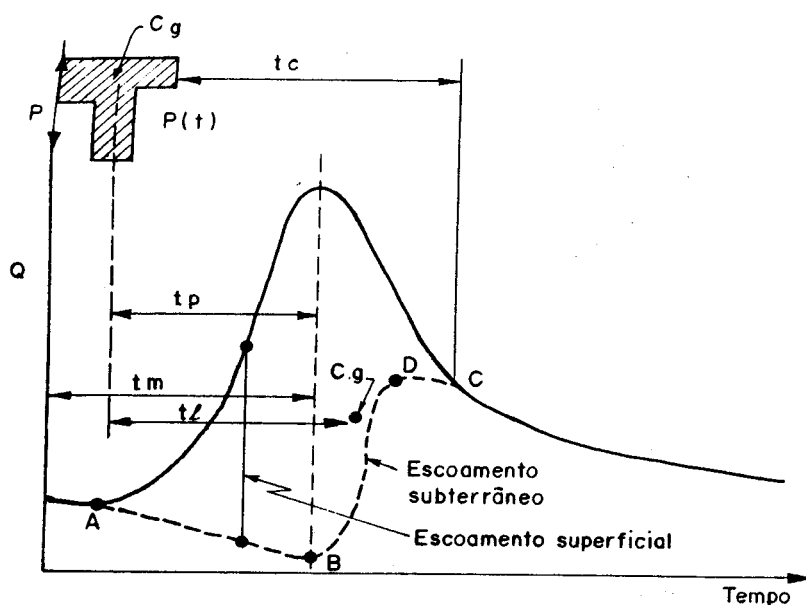
Figura 3.- Hidrograma tipo, tomada de Tucci (1993)
