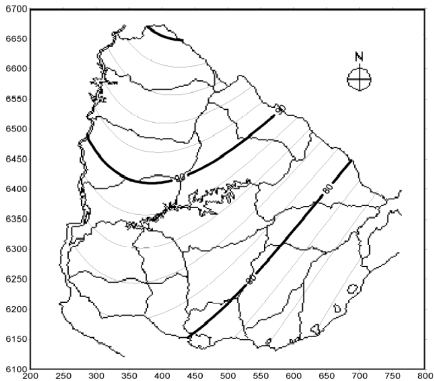
Figura 4.-Isoyetas de lluvias extremas en el Uruguay. Precipitación de 3 horas de Duración y 10 años de Período de Retorno. Fuente: Genta et al. (1998)
