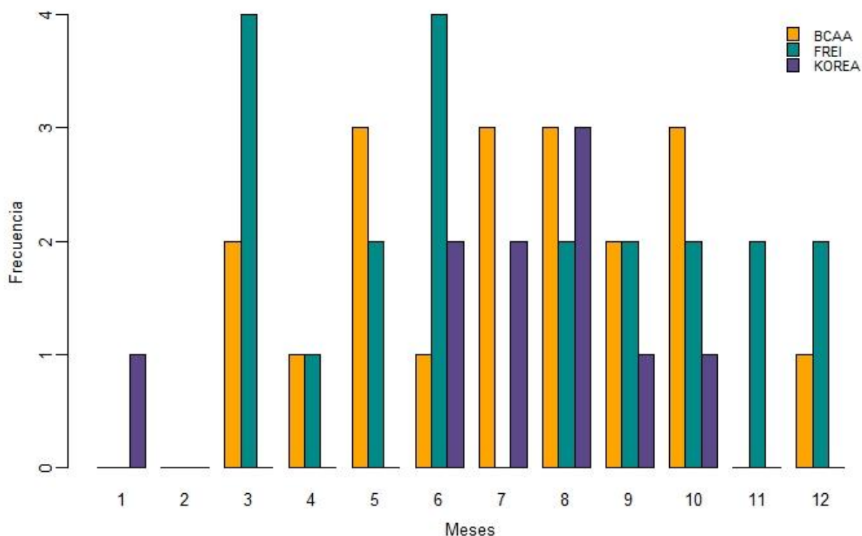
Figura 55. Distribución mensual de los ECE para las 3 estaciones (BCAA, FREI y KOREA).
