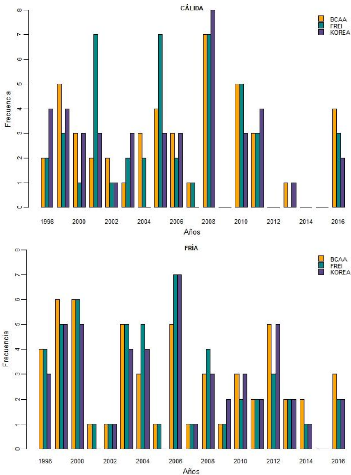
Figura 52. Distribución anual de los EC para la época cálida (superior) y fría (inferior), para las 3 estaciones: BCAA (naranja), FREI (verde) y KOREA (violeta).
