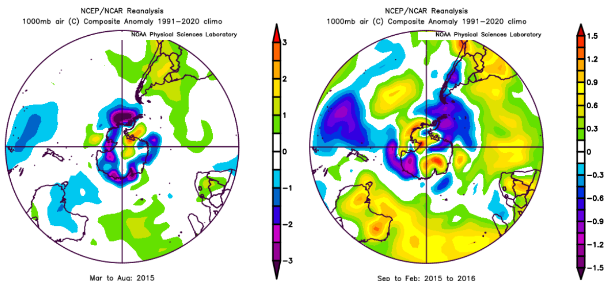
Figura 48. Anomalía anual de temperatura para el año 2015 (superior) para la región 40-90°S. Anomalía de temperatura para la estación fría Mar-Ago (izquierda) y cálida Set-Feb (derecha). Fuente: Physical Sciences Laboratory, NOAA.
