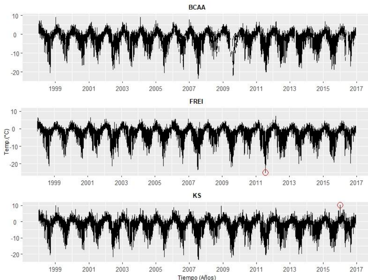
Figura 15. Variabilidad anual de la temperatura del aire en las tres estaciones: BCAA (arriba), FREI (centro) y KS (abajo). Los círculos rojos señalan el mínimo y máximo absoluto de temperatura.
