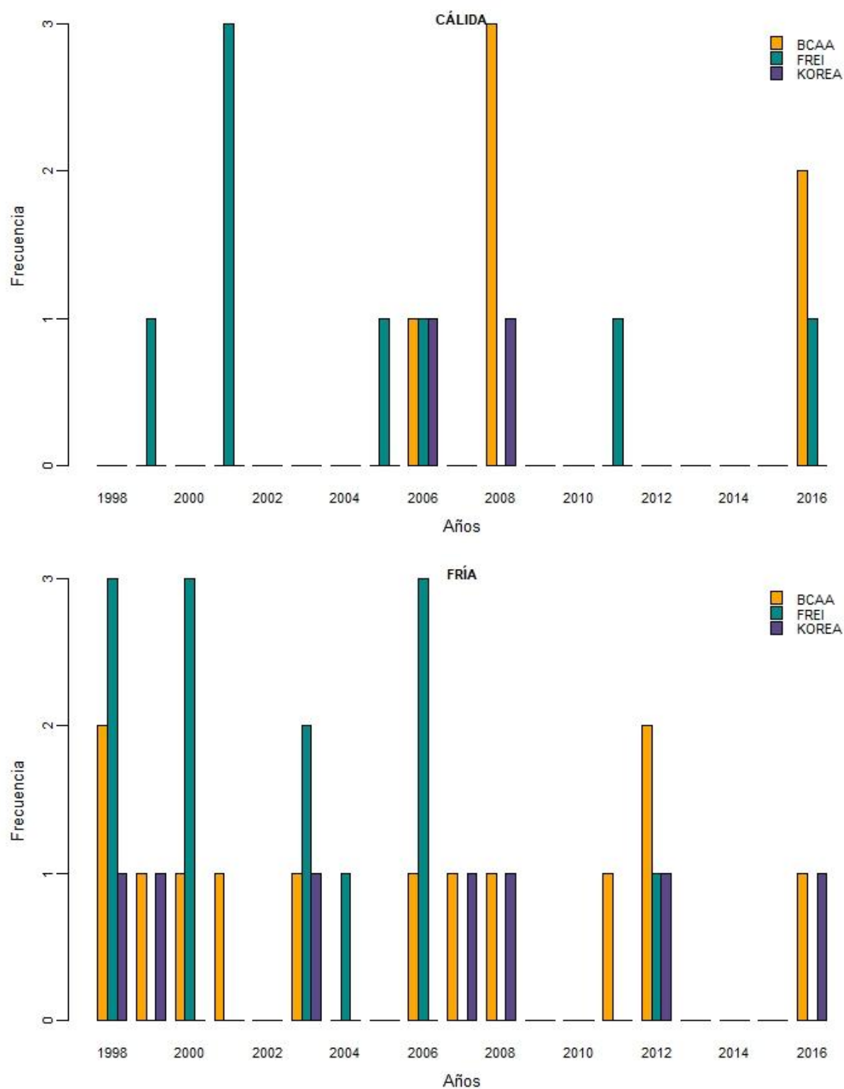
Figura 57. Distribución anual de los ECE en la época cálida (superior) y fría (inferior), para las 3 estaciones: BCAA (naranja), FREI (verde) y KOREA (violeta).
