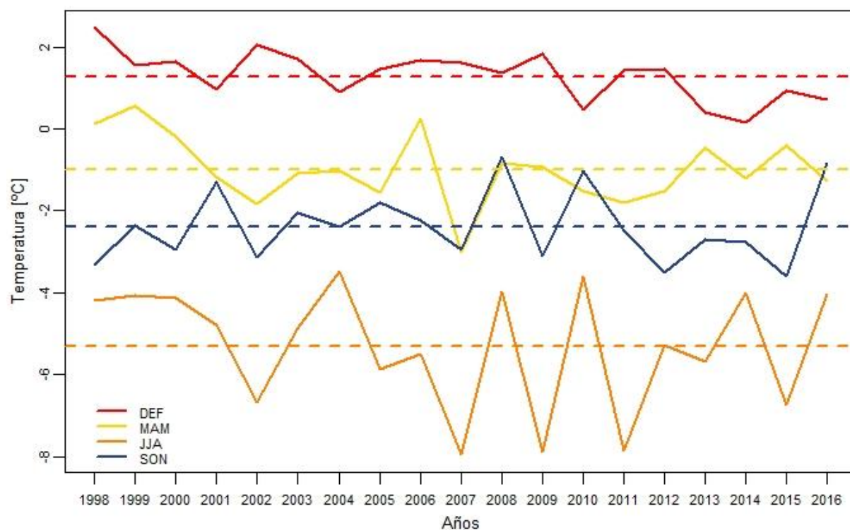
Figura 42. Temperatura media anual para cada una de las estaciones: verano (DEF, rojo), otoño (MAM, amarillo), invierno (JJA, naranja) y primavera (SON, azul). Las líneas punteadas corresponden a la media climatológica de cada estación.
