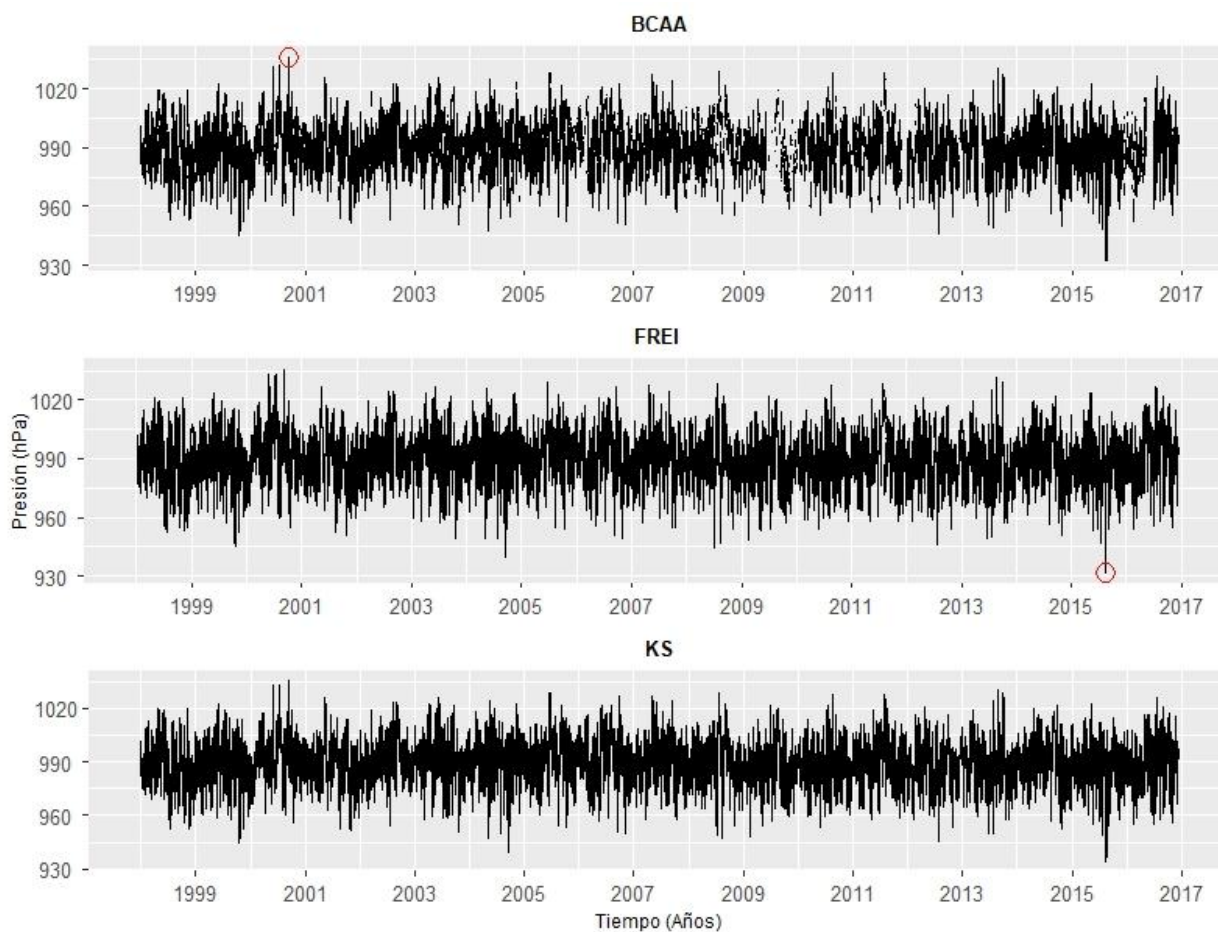
Figura 16. Variabilidad anual de la presión atmosférica en las tres estaciones: BCAA (arriba), FREI (centro) y KS (abajo). Los círculos rojos señalan el mínimo y máximo absoluto de presión.
