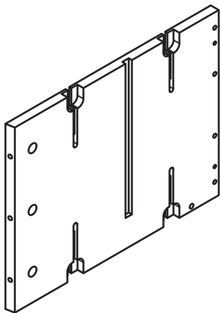
Vista Isométrica
