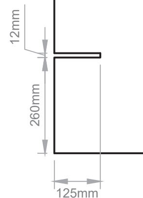
Vista Posterior
