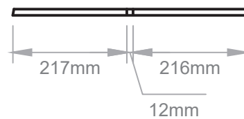
Vista Superior
