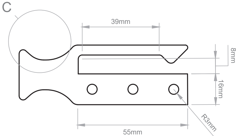
Vista Posterior
