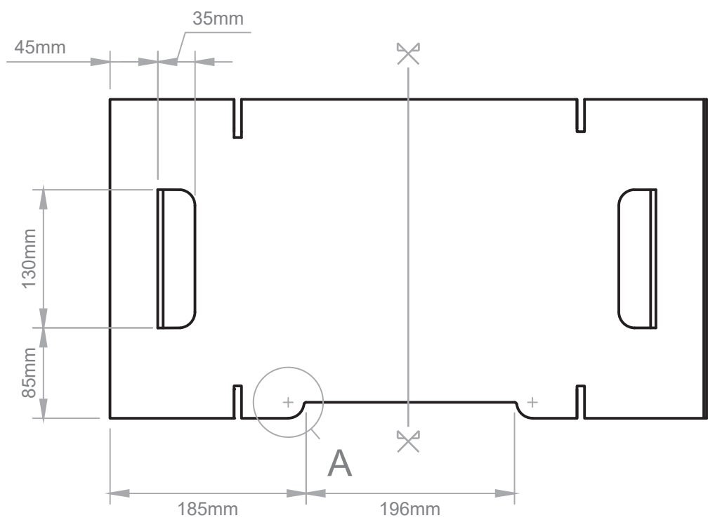
Vista Posterior
