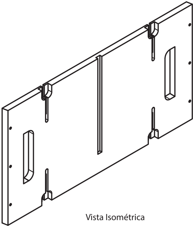
Vista Isométrica
