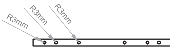
Vista Inferior
