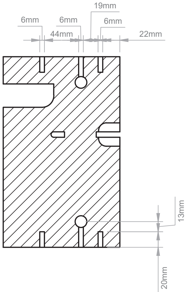
A-A (1:3)
