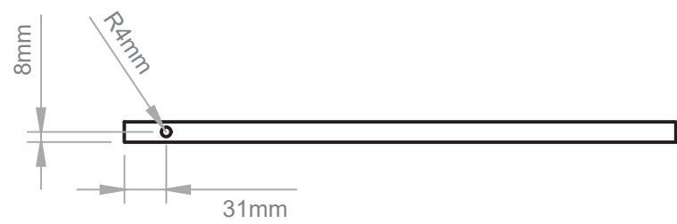
Vista Superior
