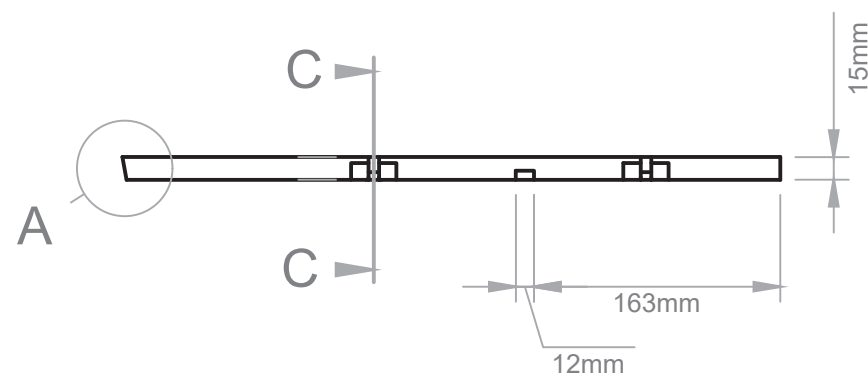
Vista Superior
