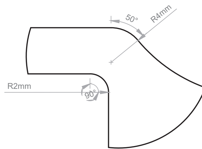
B (4:1)
