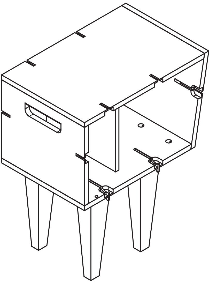
Vista Isométrica
