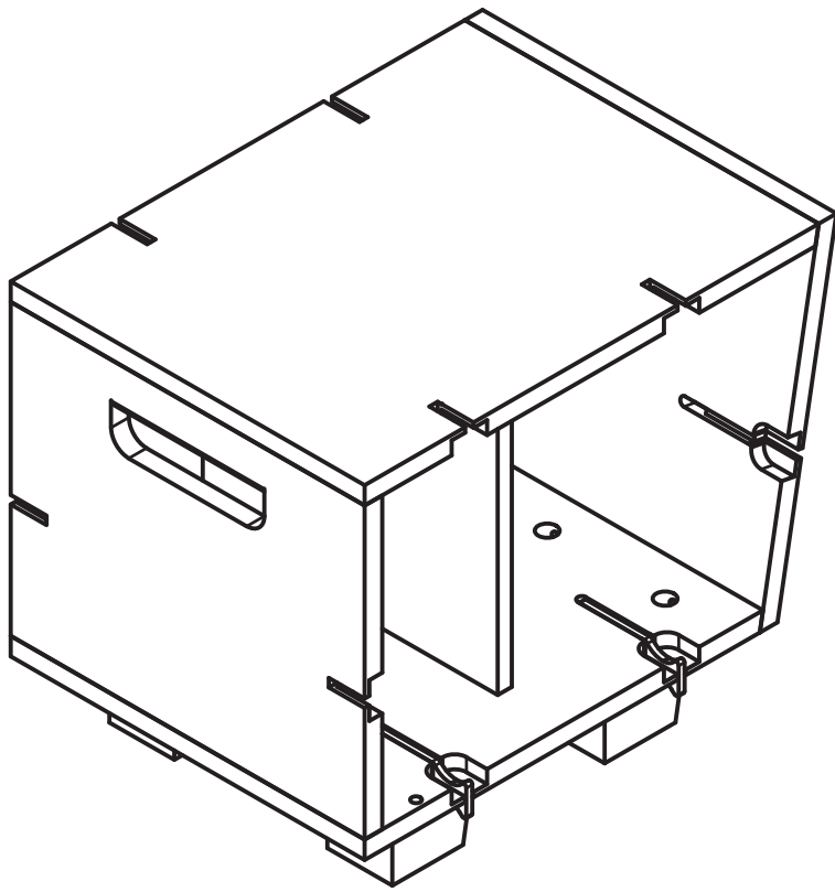
Vista Isométrica
