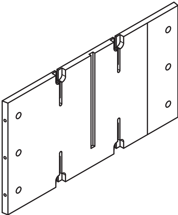
Vista Isométrica
