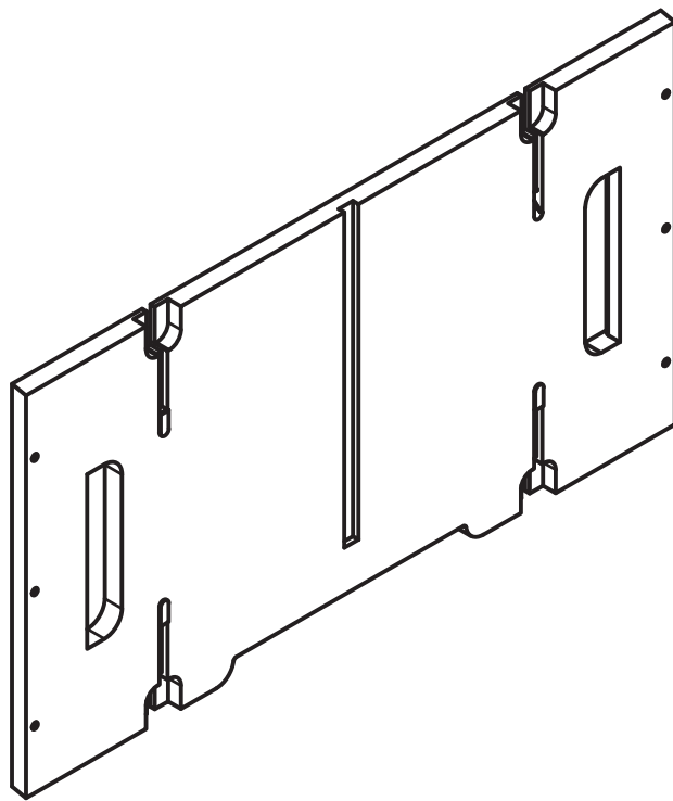
Vista Isométrica
