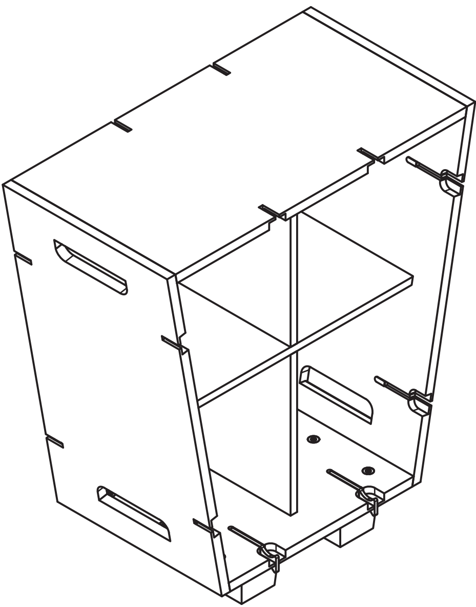
Vista Isométrica
