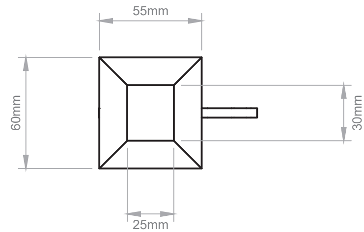
Vista Inferior
