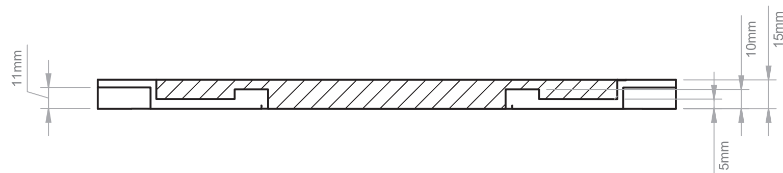
C-C (1:2)
