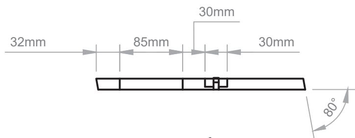
Vista Inferior
