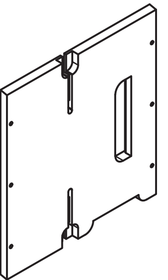
Vista Isométrica
