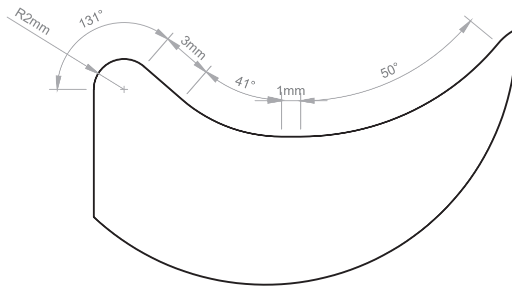
C (4:1)
