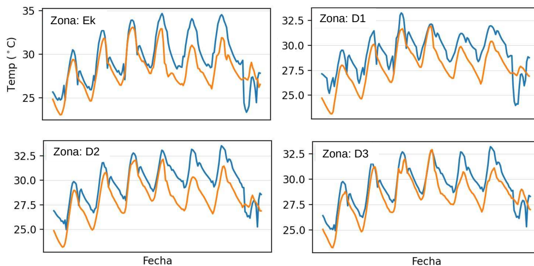
Figura 2: Temperaturas medidas y simuladas para las diferentes zonas térmicas de la vivienda tradicional para el periodo de verano. Azul: Mediciones; Amarillo: Simulaciones.
