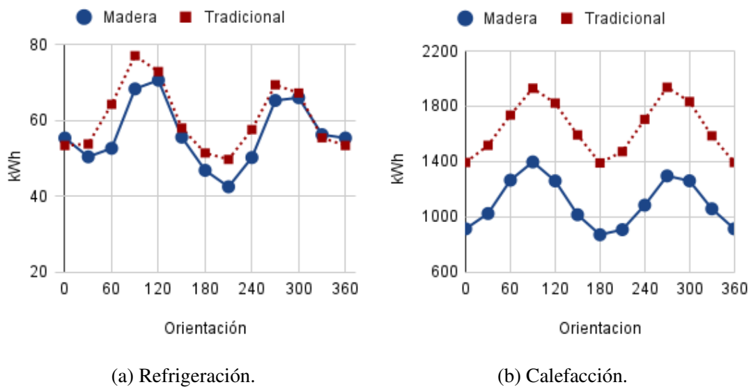
Figura 5: Requerimiento anual de energía para acondicionamiento térmico para ambas viviendas en función de la orientación de la fachada principal.
