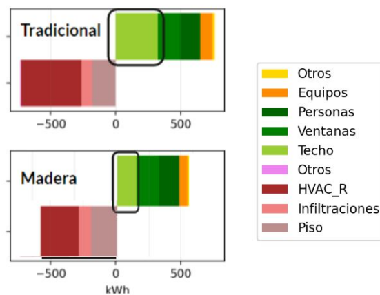
Figura 6: Aporte de energía para el mes de Enero para ambos casos para orientación 0^\circ
