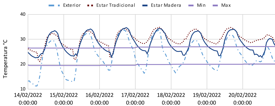
Figura 8: Temperatura durante una semana de invierno en la zona Ek para ambas viviendas.
