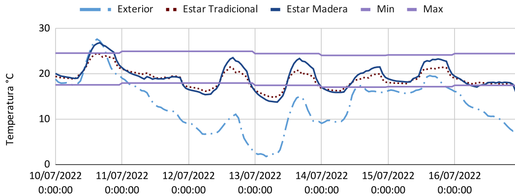
Figura 7: Temperatura durante una semana de verano en la zona Ek para ambas viviendas.
