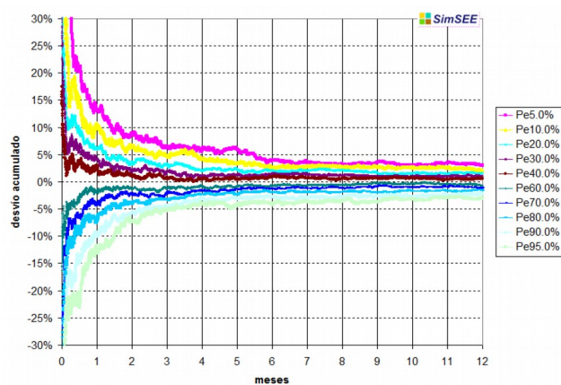
Fig. 2: Desvío de la generación Eólica acumulada para diferentes cortes de probabilidad.
