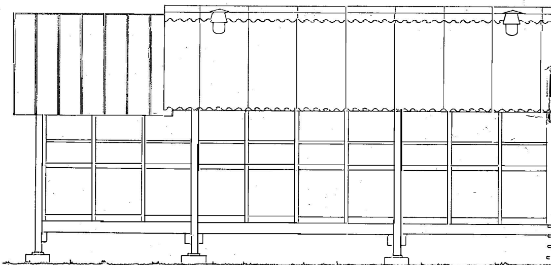
FACHADA NORTE
