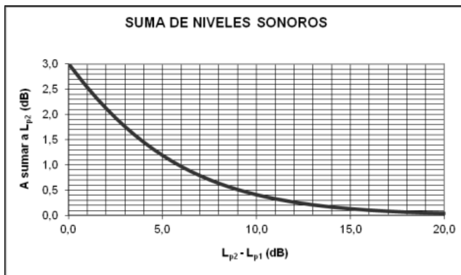
Figura 2-1. Ábaco para suma de niveles sonoros
