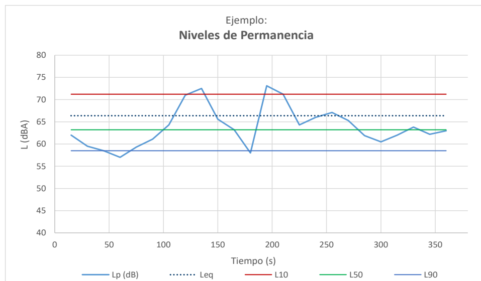
Figura 3-2. Niveles de permanencia
