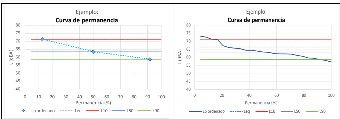
Figura 3-3. Curva de permanencia de niveles de presión sonora (izq. 3 puntos; der. 24 puntos)
