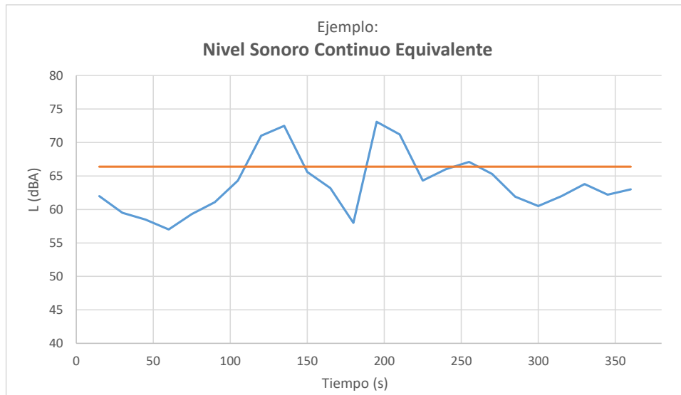
Figura 3-1. Nivel sonoro continuo equivalente
