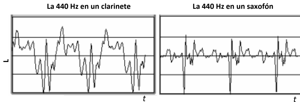
Figura 1-1: Gráfico L(t) de un sonido de 440 Hz emitido por un clarinete (izq.) y un saxofón (der.) (tomado de Jordà Puig, 1997) Nótese que, aun tratándose de sonidos de la misma frecuencia, la forma de la onda y la evolución de la intensidad sonora en el tiempo tienen comportamientos diferentes
