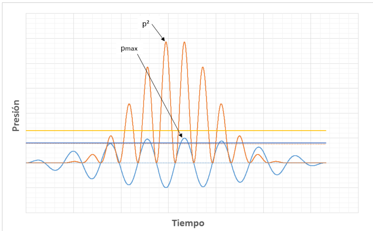
Figura 1-2. Representación de la presión eficaz: en el gráfico se observa p(t) (celeste); p^2(t) (naranja); media de p^2(t) (recta amarilla) y raíz cuadrada de la media de p^2(t) (recta azul).
