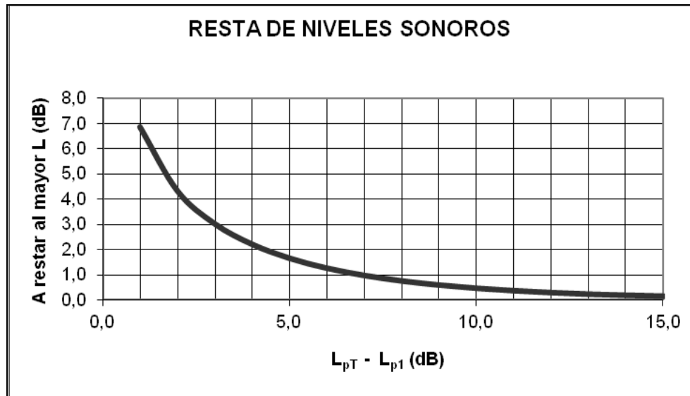
Figura 2-2. Ábaco para restar niveles sonoros
