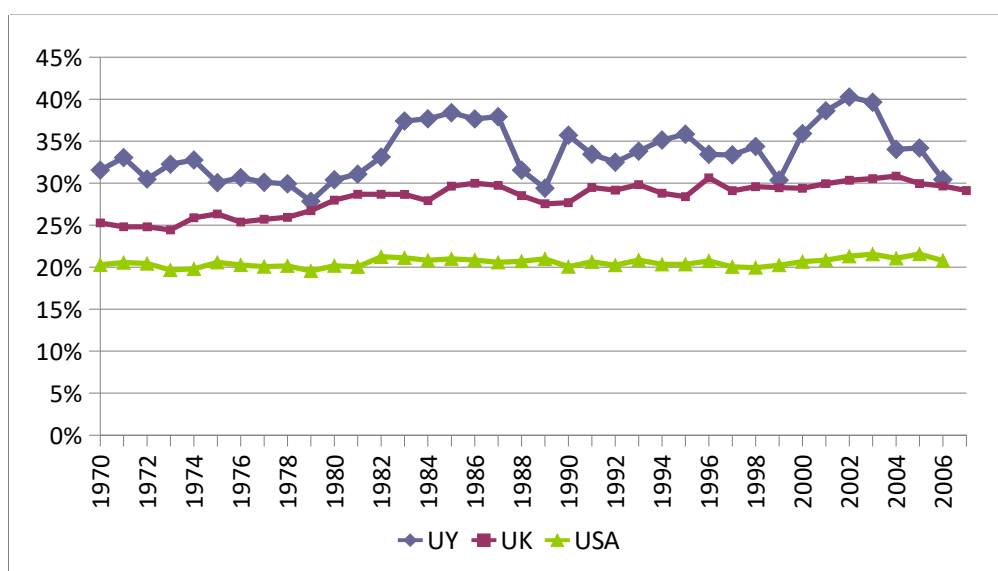
Gráfico 4. URUGUAY, USA Y REINO UNIDO. Participación del Consumo Residencial en el Total de Energía Final (%)
