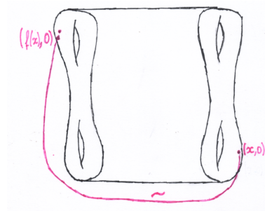
Figura 5.5: Ejemplo de Mapping torus
