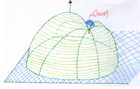
Figura 4.4: Caso n = 3
