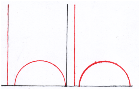
Figura 2.3: Geodésicas del Semi-Plano
