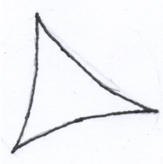
Figura 3.1: Triángulo Hiperbólico
