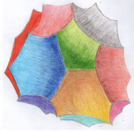
Figura 5.2: Poliedro hiperbólico de dimensión 3
