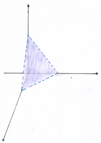
Figura 4.5: Conjunto \Delta^2
