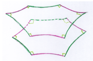
Figura 6.2: Pegado de Hexágonos para formar P
