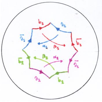
Figura 5.3: Octógono Hiperbólico
