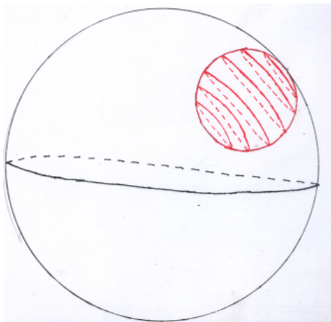
Figura 3.4: Horoesfera en el modelo de la Bola
