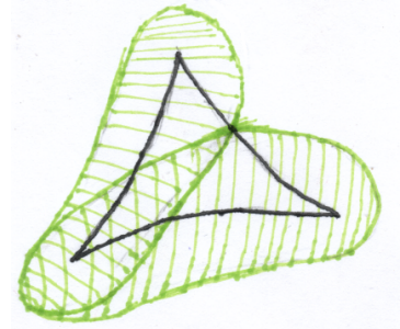
Figura 3.2: \delta -entornos
