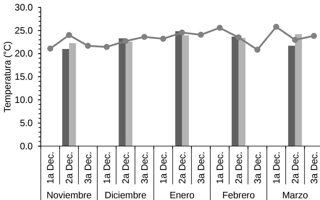
1a Dec: Primera decada. 2a Dec: Segunda decada . 3a Dec: Tercera decada. Columna gris oscura: Temperatura promedio mensual del periodo 2002-2020. Columna gris clara: Temperatura promedio mensual del periodo 2019-2020. Línea gris: Temperatura decádica del periodo 2019-2020. Figura 4. Temperaturas (°C) promedio mensuales y decádicas durante la zafra 2019-2020 ocurridas en la EEMAC (Paysandú) y valores promedio mensuales de la serie histórica 2002-2020.
