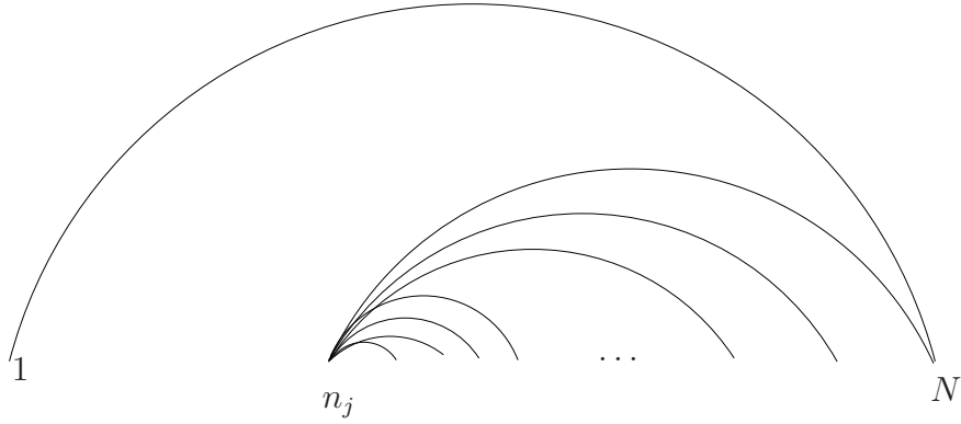
Figura 5.1: Tiempo Hiperbólico
