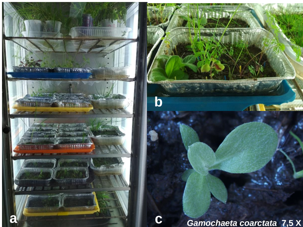
Figura 6. a. Seguimiento del experimento en cámara germinadora. b. Bandeja con las diferentes especies germinando. c. Gamochaeta coarctata , una de las especies que presentó mayor densidad.
