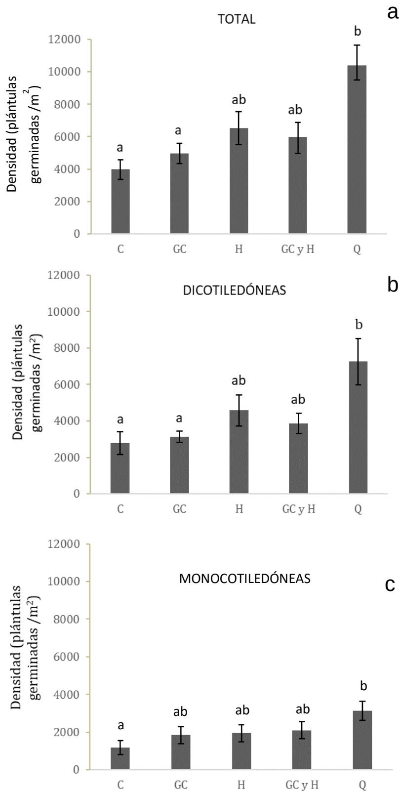
Figura 7. Densidad de plántulas germinadas \pm 1EE del banco de semillas de un pastizal del Paisaje Protegido Quebrada de los Cuervos, sujeto a cinco tratamientos: control (C), golpe de calor (GC), humo (H), golpe de calor y humo (GCyH) y quema in situ (Q) Las letras distintas indican diferencias significativas entre los tratamientos con p < 0,05 .
