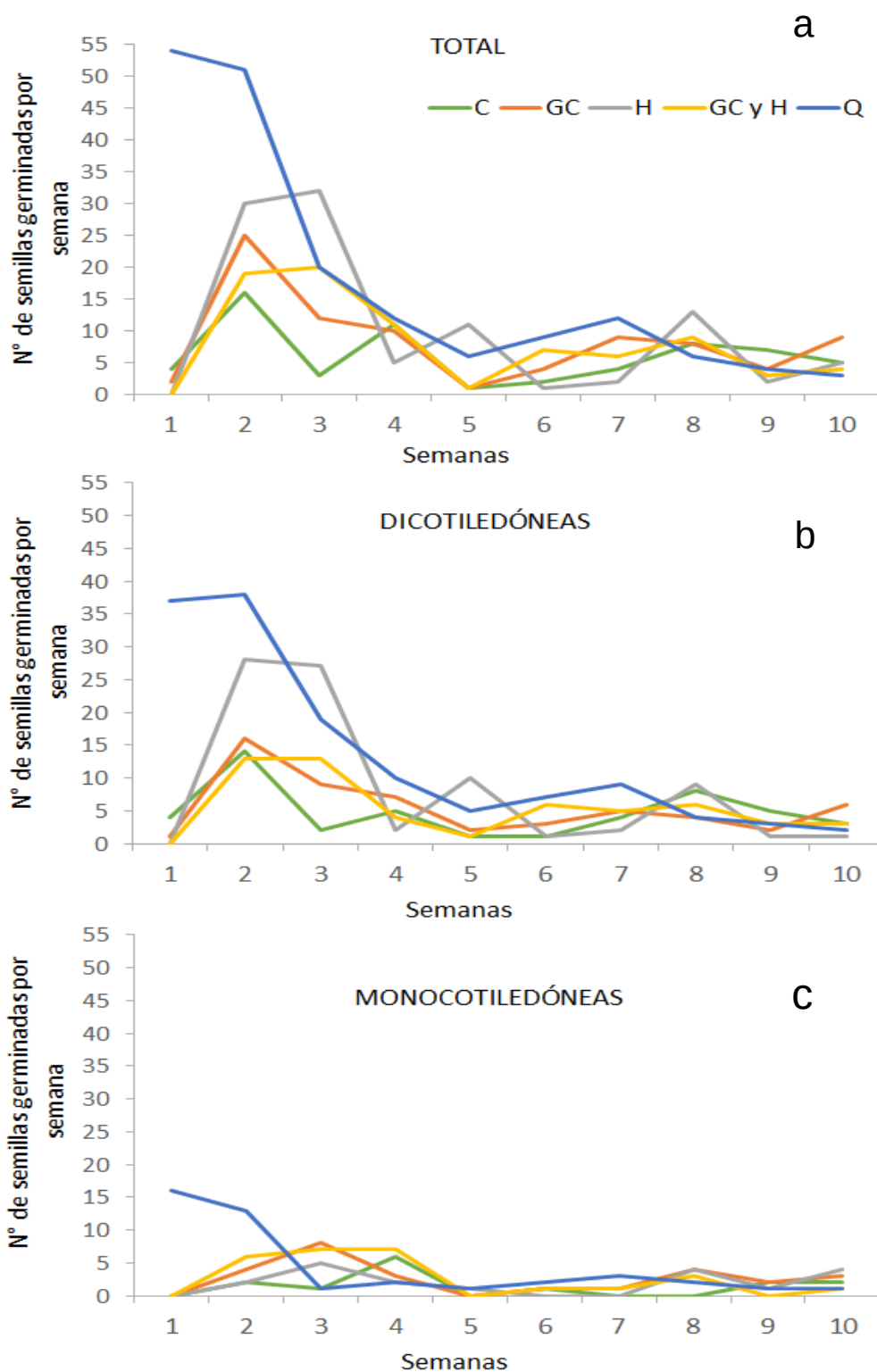
Figura 9. Especies germinadas semanalmente a partir del banco de semillas de un pastizal del Paisaje Protegido Quebrada de los Cuervos, sujeto a cinco tratamientos: control (C), golpe de calor (GC), humo (H), golpe de calor y humo (GCyH) y quema in situ (Q). Sólo se muestran las primeras 10 semanas, de las 20 que duró el experimento.
