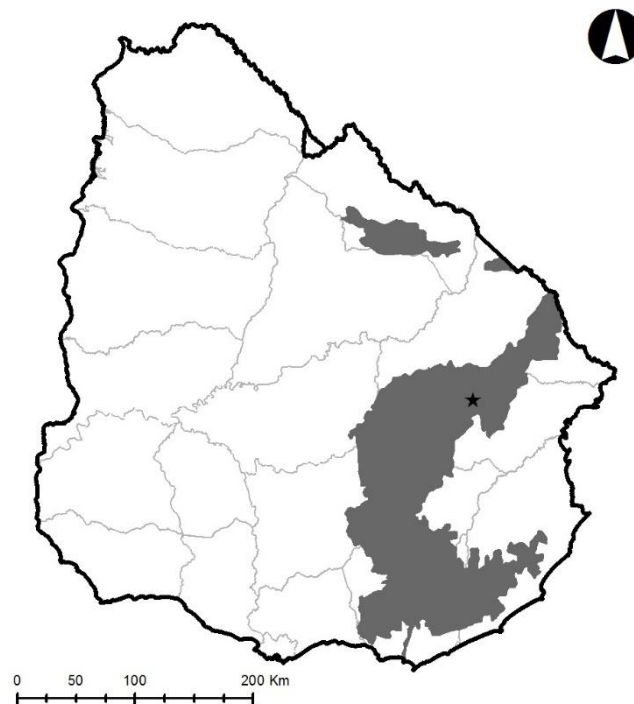
Figura 2. Mapa de Uruguay en el que se muestra en gris la región geomorfológica Sierras del Este.★: zona de estudio, Paisaje Protegido Quebrada de los Cuervos en el Departamento de Treinta y Tres, Uruguay.
