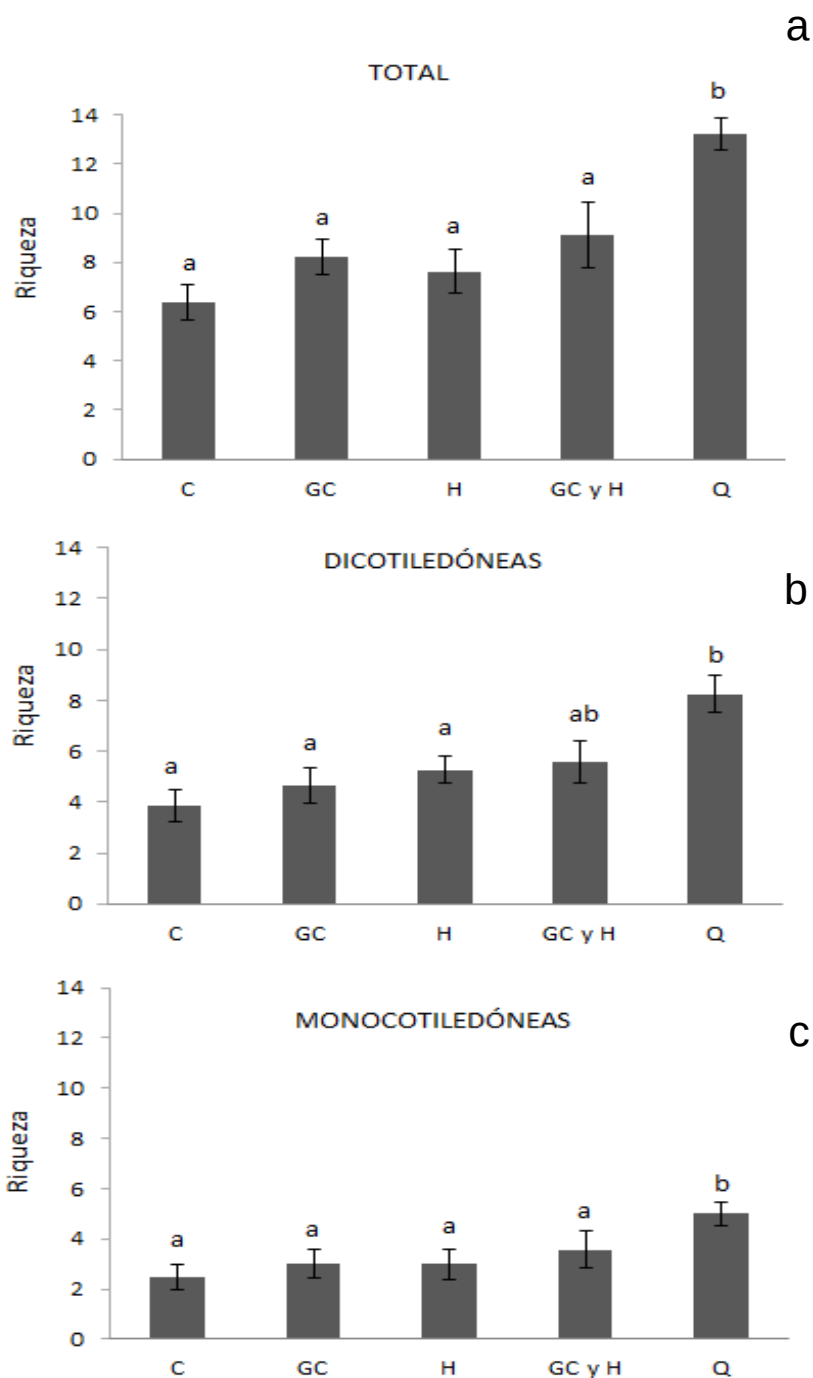
Figura 8. Riqueza de especies germinadas \pm 1EE del banco de semillas de un pastizal del Paisaje Protegido Quebrada de los Cuervos, sujeto a cinco tratamientos: control (C), golpe de calor (GC), humo (H), golpe de calor y humo (GCyH) y quema in situ (Q). Las letras distintas indican diferencias significativas entre los tratamientos con p < 0,05 .
