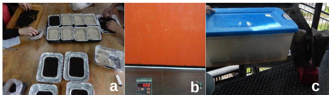
Figura 5. Montaje y aplicación de tratamientos. a. Colocación de suelo disgregado en bandejas. b. Golpe de calor en estufa de secado. c. Aplicación de humo con ahumador de apicultor.
