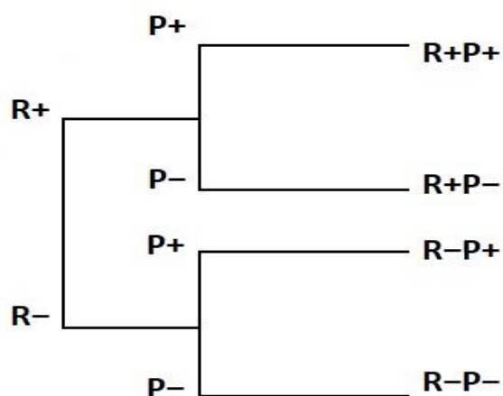
Figura 1. Clasificación de las cuatro respuestas básicas al fuego según Pausas et al. (2004). R+ : rebrotadoras, R- : no rebrotadoras, P+ : propágulos persistentes, P- : propágulos no persistentes. Las dos dicotomías son: en primer lugar, si las plantas persisten después del incendio por rebrote y, en segundo lugar, si las plantas persisten después del incendio por germinación. Los cuatro grupos son: R+P+ (especies facultativas), R+P- (rebrotadoras obligadas; las semillas no resisten el fuego y el reclutamiento es por rebrote durante el período entre incendios), R-P+ (germinadoras obligadas; estas solo persisten por semillas; por lo tanto, están especializadas en el reclutamiento posterior al incendio) y R-P- (especies que no persisten después del incendio).
