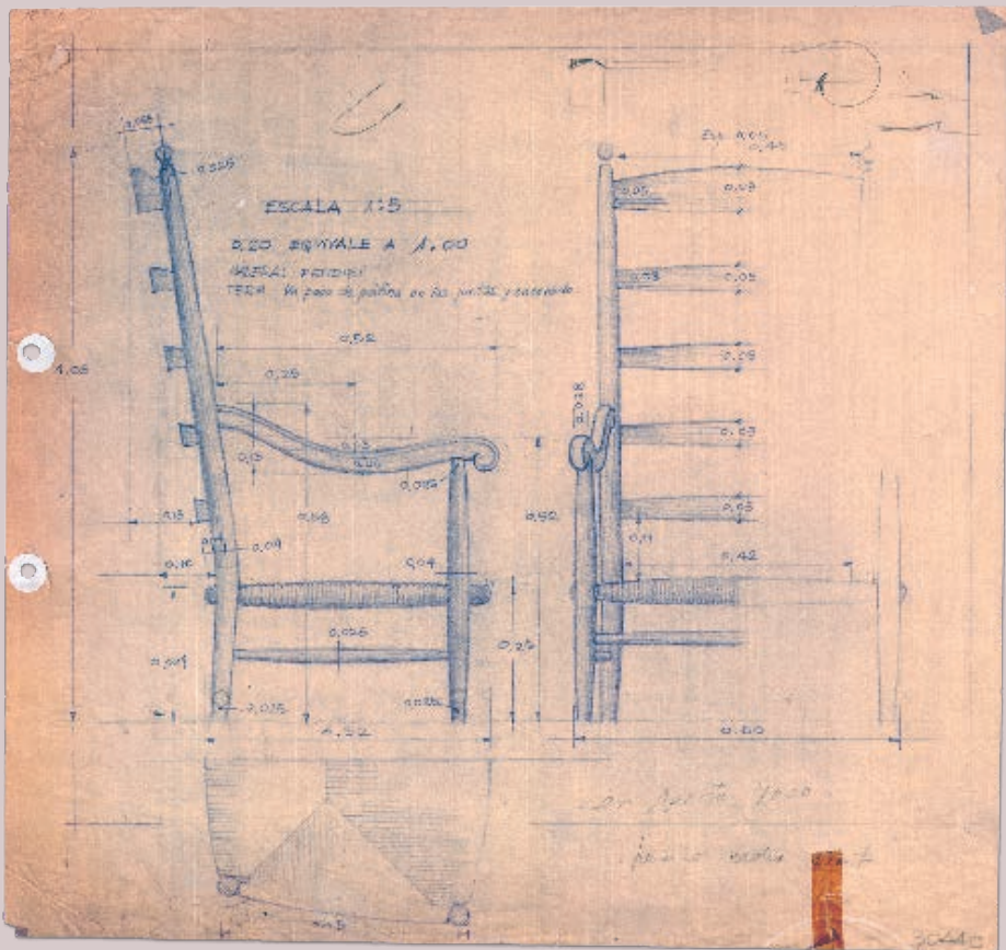
FIGURA 16. PLANTILLA PARA LA FABRICACIÓN DE UNA SILLA. LÁPIZ SOBRE PAPEL.
