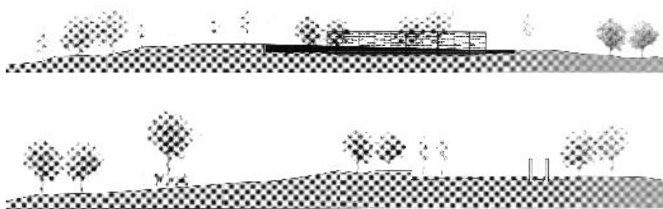
FIGURA 12. MEMORIAL EN RECORDACIÓN DE LOS DETENIDOS DESAPARECIDOS. KOHEN, OTERO, SAGRADINI, DODERA, LÓPEZ DE HARO, FRONTINI. CORTES.
