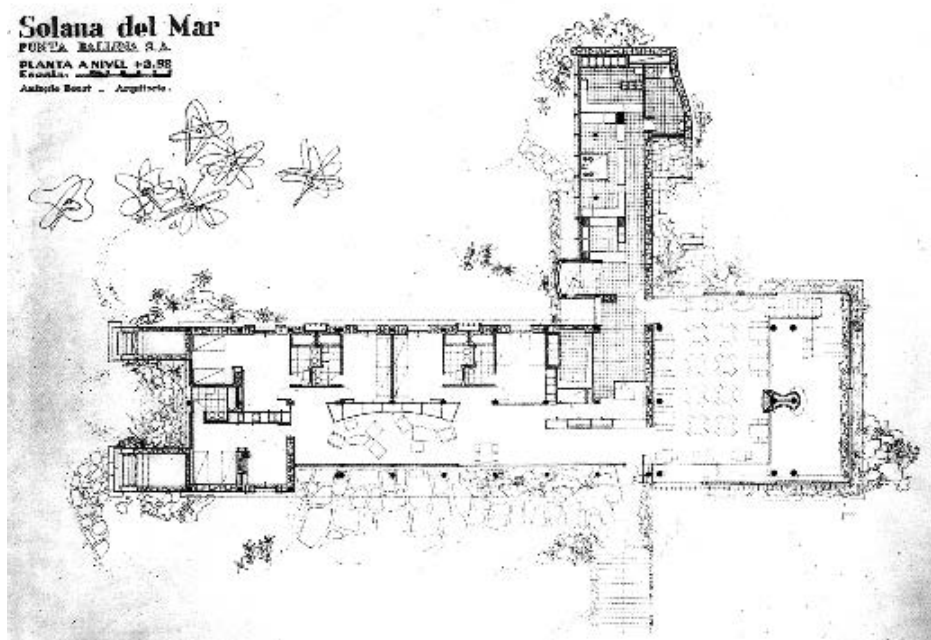
FIGURA 1. SOLANA DEL MAR (BONET, 1946). PLANTA ALTA: COMEDOR, GALERÍA Y DORMITORIOS.
