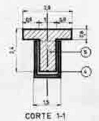
CORTE 1-1
