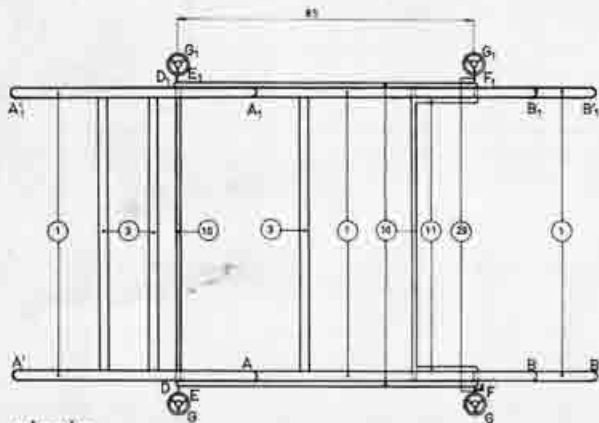
planta ESC-1/10
