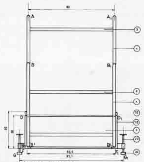
alzado frontal ESC-1/10
