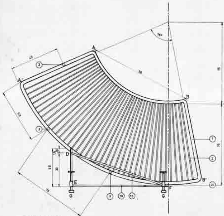
alzado lateral ESC-1/10
