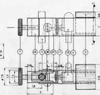
detalle fijación pieza nº 4 ESC-1/1 CANTIDAD: 24
