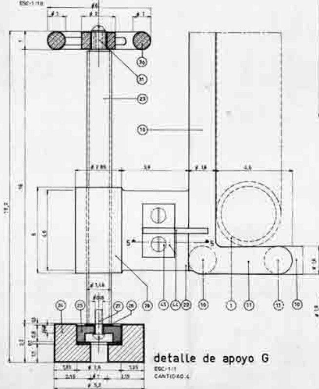
planta ESC-1/10
