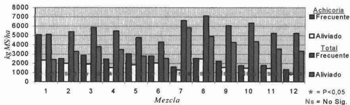
Figura 9. Producción de achicoria y total de cada mezcla durante la primavera.
