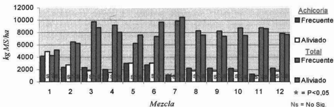
Figura 10. Producción de achicoria y total de cada mezcla durante el verano.
