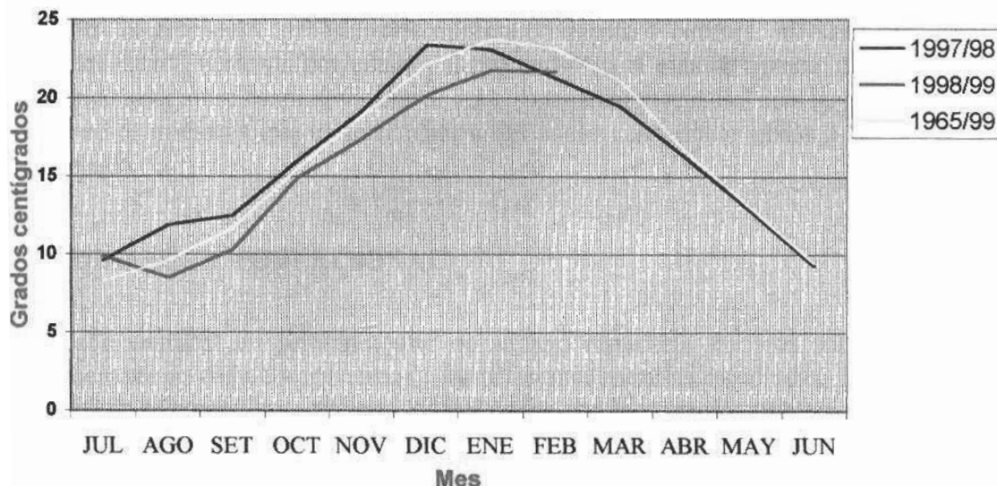
Figura 7. Temperatura media del suelo cubierto a 5 cm 1997/98, 1998/99 y 1965/99.
