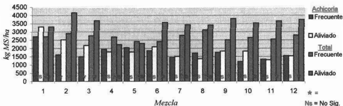
Figura 12. Producción de achicoria y total de cada mezcla durante el invierno.
