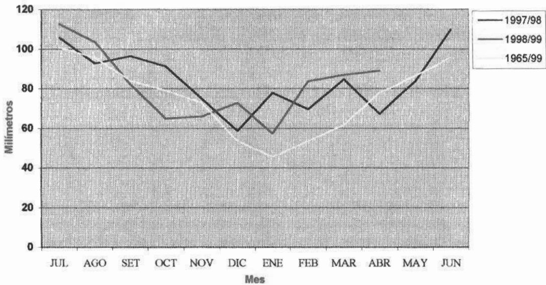
Figura 5. Agua disponible 1997/98, 1998/99 y 1965/99.
