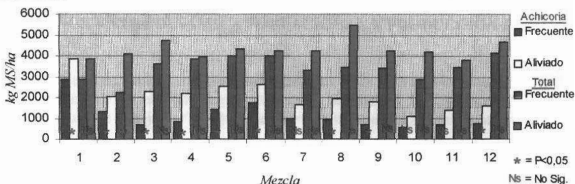
Figura 13. Producción de achicoria y total de cada mezcla durante la primavera 2.
