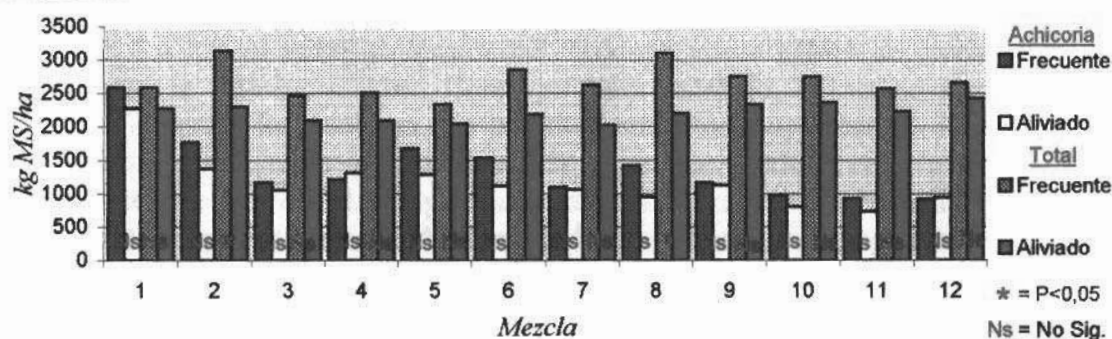
Figura 11. Producción de achicoria y total de cada mezcla durante el otoño.
