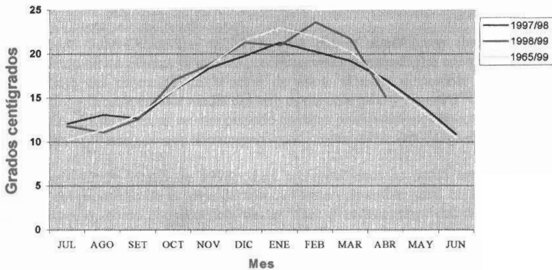
Figura 6. Temperatura media del aire 1997/98, 1998/99 y 1965/99.
