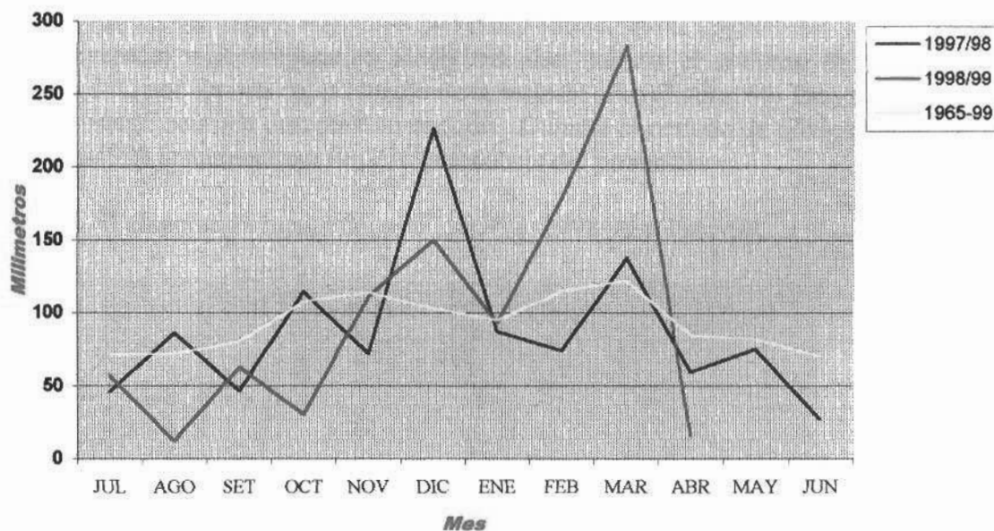
Figura 4. Precipitaciones mensuales 1997/98, 1998/99 y 1965/99.
