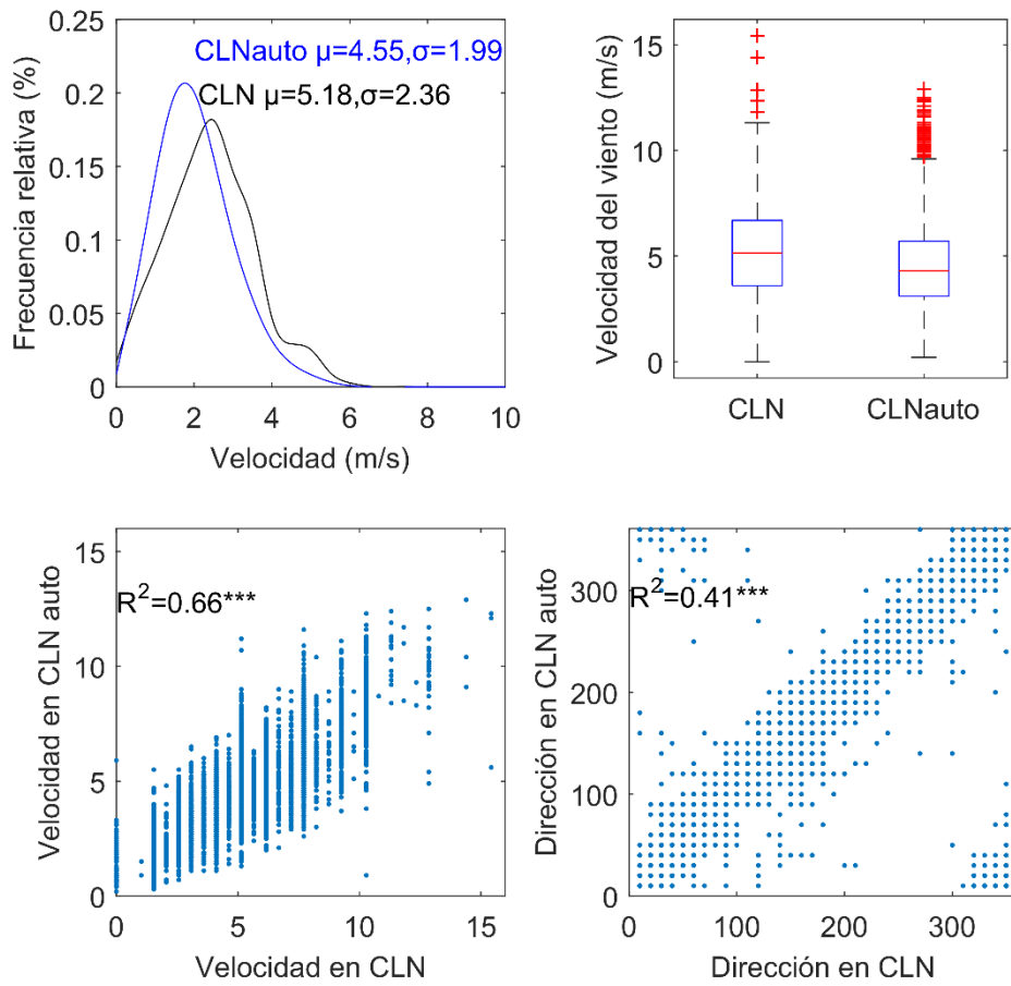
Figura 2.7. Comparación entre registros en Colonia (CLN) en el periodo de solapamiento entre la automática y la convencional. (***) p < 0,001 ; n para dirección=5729 y velocidad= 6197).
