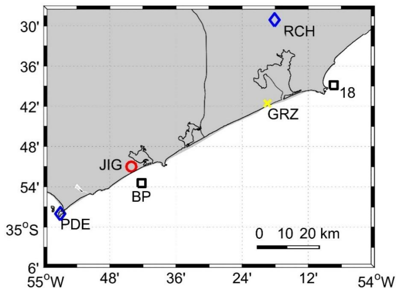
Figura 5.1. Región de la costa atlántica seleccionada para el estudio de brisa con alta resolución. El círculo rojo indica la posición de José Ignacio (JIG), estación de referencia. Se observan otras estaciones cercanas en
