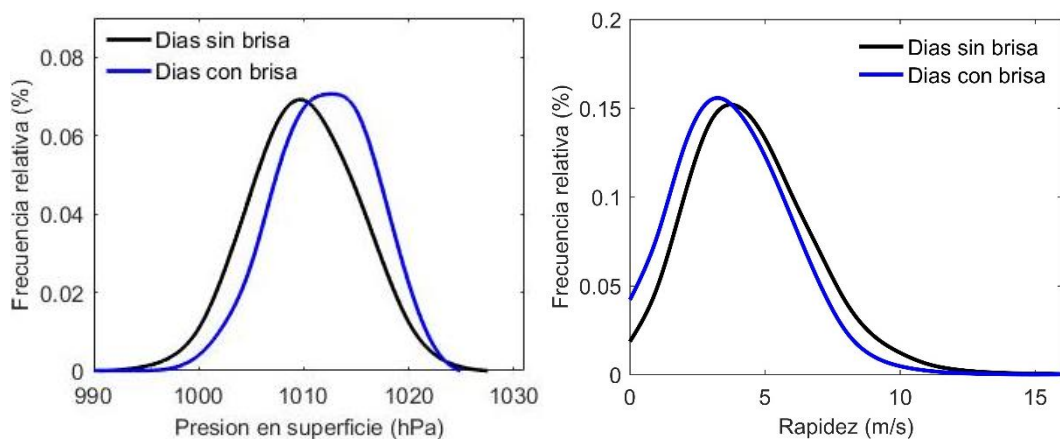
Figura 4.19. Distribución de frecuencias relativas de la presión en superficie (izquierda) y módulo de la velocidad (derecha) para los días de brisa generalizada y los de no brisa generalizada. Los datos corresponden a todas las estaciones seleccionadas con medición durante dic-mar 2011-2016.
