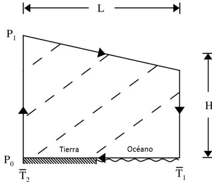
Figura 1.1. La brisa marina y el teorema de la circulación de Bjerknæs. La tierra está a la izquierda, el océano está a la derecha. Las flechas indican el sentido de la circulación. T_1 y T_2 indican la temperatura media a través de las columnas verticales sobre las superficies de la tierra o el mar. Las líneas punteadas son isopícnas, con un aire más denso en la parte inferior derecha. P_0 y P_1 son la presión en superficie y altura respectivamente. L y H son la extensión horizontal y vertical de la celda de circulación, respectivamente. Modificado de Miller et al. (2003).
