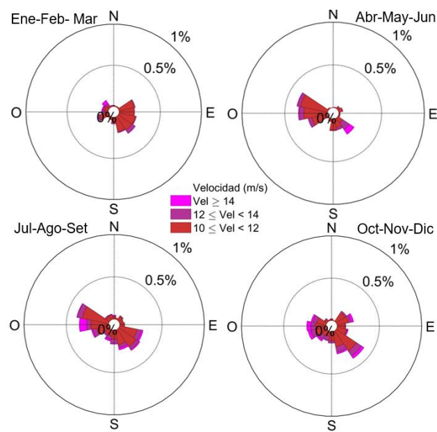
Figura 3.3. Rosa de vientos por trimestre en la estación de José Ignacio.
