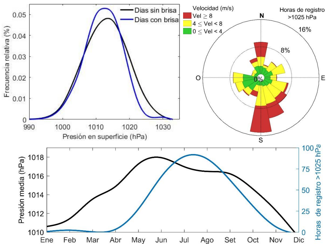
Figura 4.18. Arriba izquierda: Distribución de frecuencias relativas de la presión en superficie durante los días de brisa generalizada y los de no
