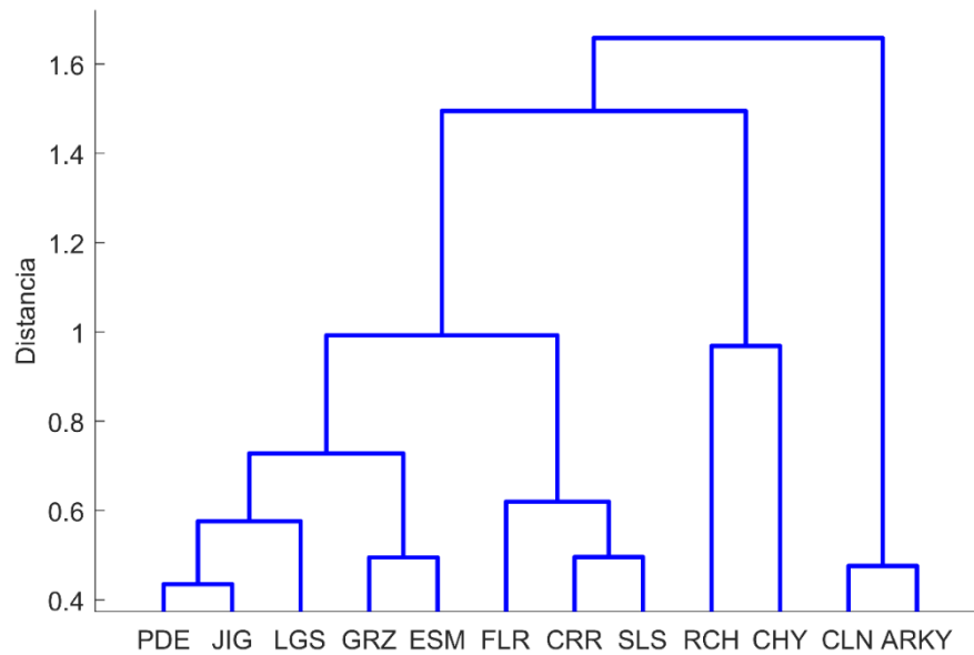
Figura 3.11. Análisis de cluster utilizando el método de Ward para la velocidad del viento. Se utilizaron 2527 datos en los que se contaba con registro simultáneo para las estaciones, fue necesario agrupar ART y KIY en ARKY ya que no coincidían en el tiempo. La medida de distancia es según la suma de varianzas de la correlación de Pearson.
