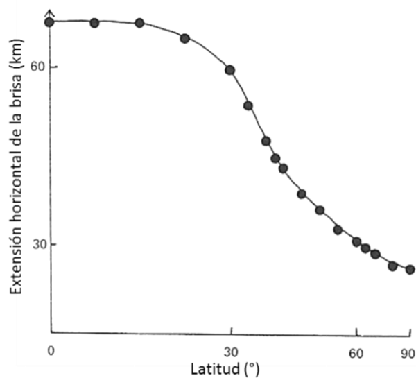
Figura 1.5. Máxima extensión horizontal que puede tomar la brisa según la latitud antes de ser torcida por Coriolis hasta una dirección paralela a la costa. Según Niino (1987).
