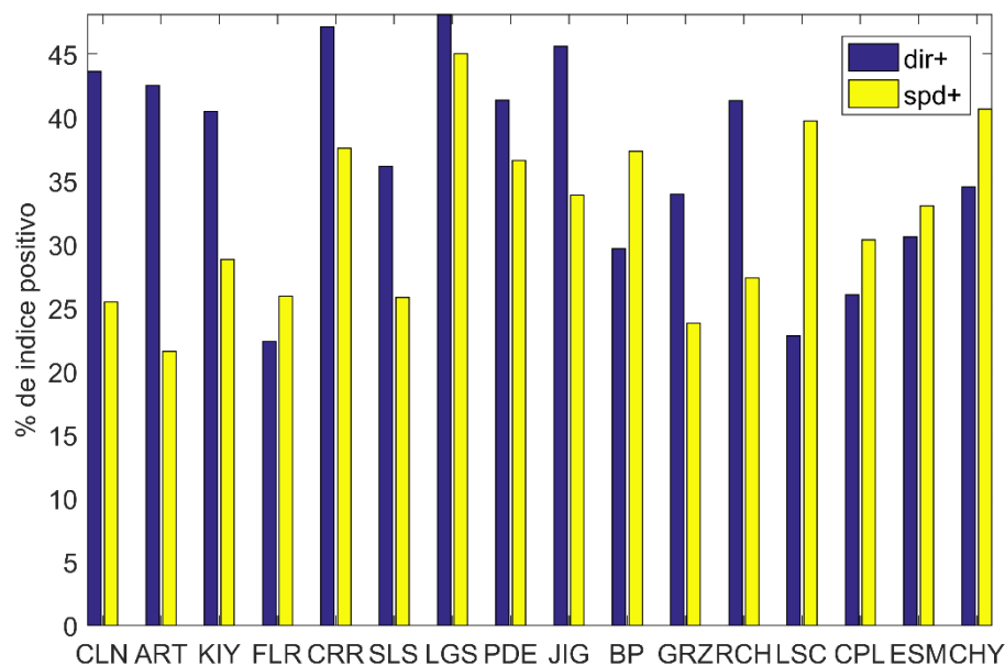
Figura 4.7. Porcentaje de casos positivos al índice con respecto a que rote el viento (azul) y se intensifique (amarillo).
