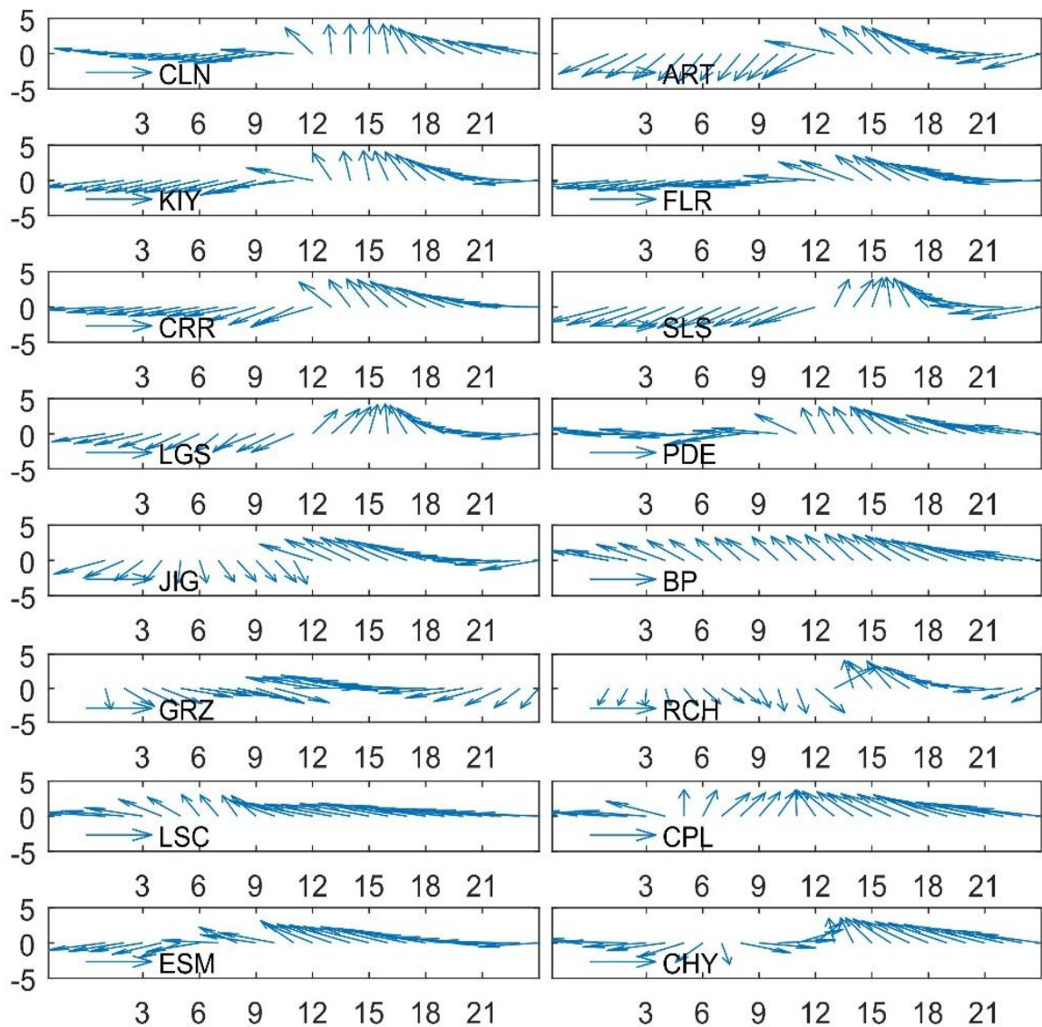
Figura 3.2. Ciclo diario de vientos ( \text{m}\cdot\text{s}^{-1} ) en todas las estaciones. Los vectores representan el promedio de u y v para cada hora con registro. El eje y representa el promedio de la velocidad (vectorial) y el x la hora del día.
