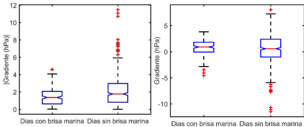
Figura 4.26. Diagrama de cajas del análisis de varianza (ANOVA) de una vía para el gradiente de presión en superficie del mar entre 36°S, 53°W y 33°S, 56°W y el factor día con (sin) brisa marina generalizada en Uruguay durante el periodo diciembre a marzo de los años 2011 al 2016 (n=728). A la izquierda se muestra el análisis utilizando el valor absoluto del gradiente de presión ( p < 0,05 ) mientras que a la derecha el valor ( p = 0,07 ). Datos de ERA-INTERIM, media diaria con resolución 0,25°.
