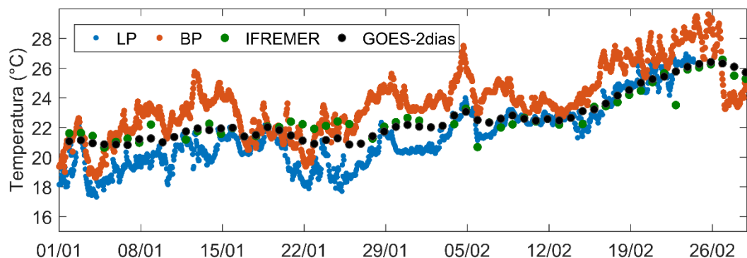
Figura 2.11. Temperatura de superficie del mar durante los meses enero y febrero de 2017 medida in situ en la Boya Petrolera (BP) de José Ignacio, La Paloma (LP) y remotamente por los productos satelitales de GOES-POES y el compilado de satélites de IFREMER en un punto intermedio entre BP y LP. Notar que LP y BP tienen resolución horaria y los GOES-POES e IFREMER diaria.
