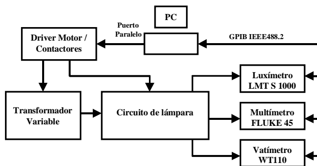
Fig. 1. Diagrama de bloques del SADE
