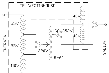
Fig. 4. Topología de conexión de los transformadores
