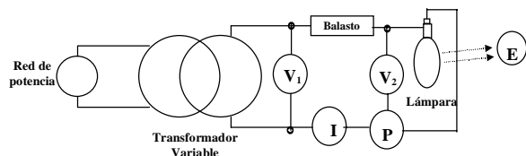
Fig. 2. Circuito de lámpara
