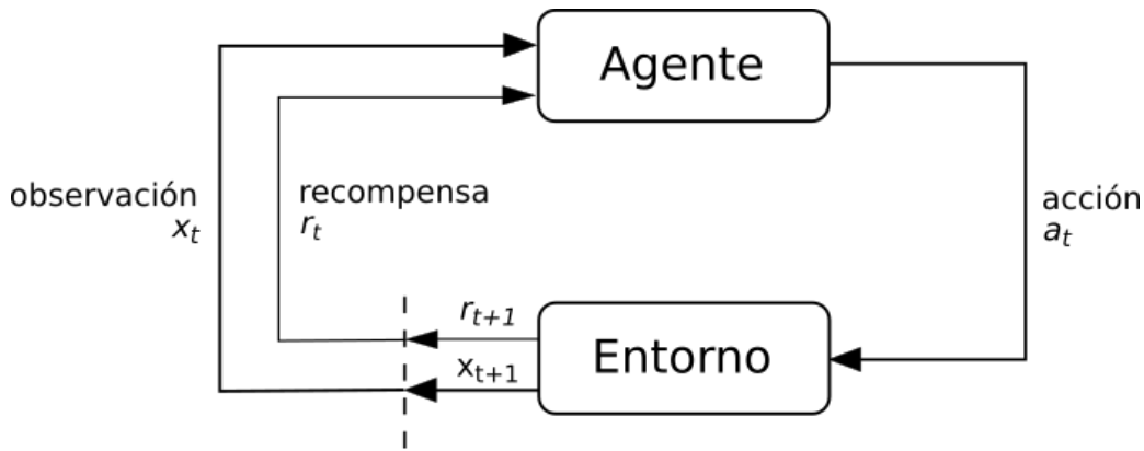
Figura 2.1: Modelo de interacción agente-entorno. Primero el agente selecciona una acción que se ejecuta en el entorno y luego como consecuencia de ella obtiene una nueva observación representativa del mismo junto a la recompensa. Imagen tomada del libro de Richard S. Sutton [38]
