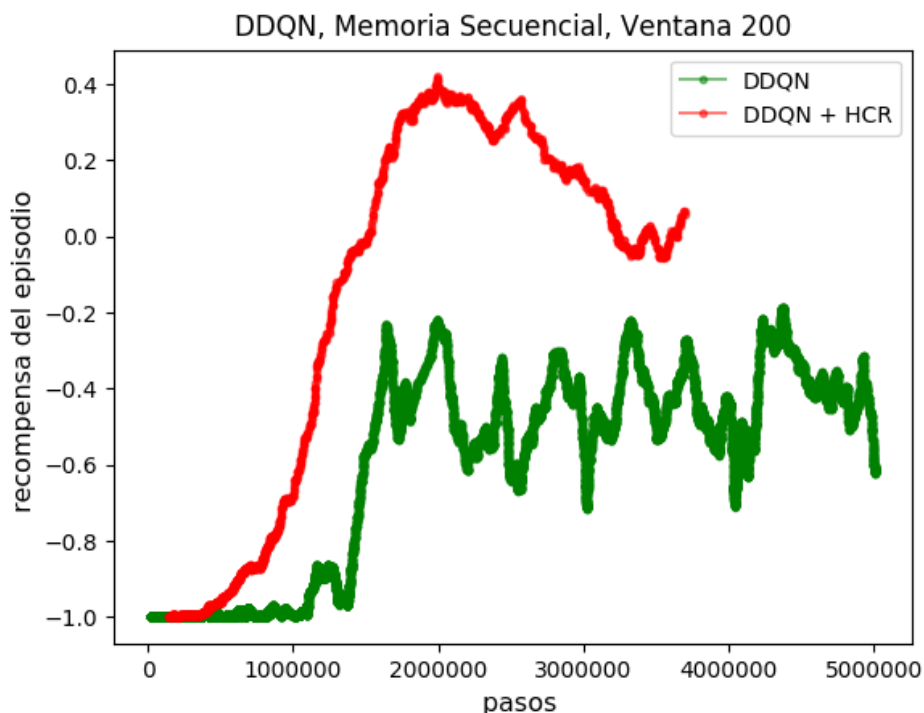
Figura 3.17: Recompensa con y sin HCR . Se muestran únicamente los episodios que empiezan en el checkpoint inicial para hacer ambos registros comparables.
