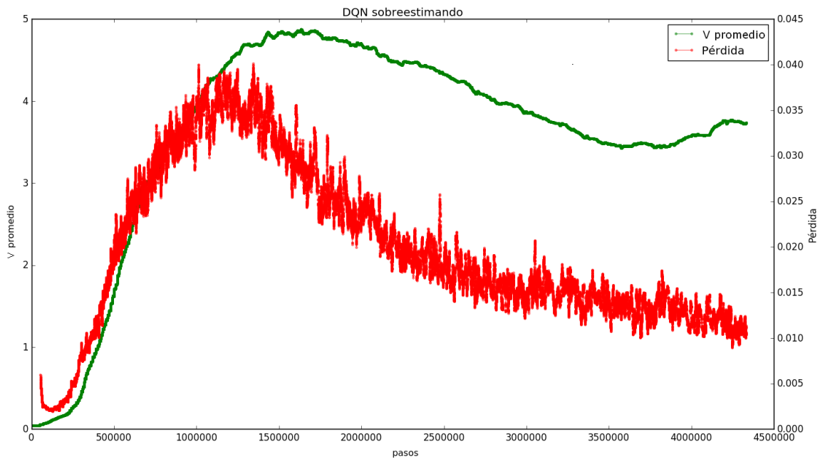
Figura 3.13: V promedio y pérdida para DQN. Puede notarse que a medida que la red se ajusta, el error disminuye y también desciende V promedio. Se muestra la media móvil con ventana 50.
