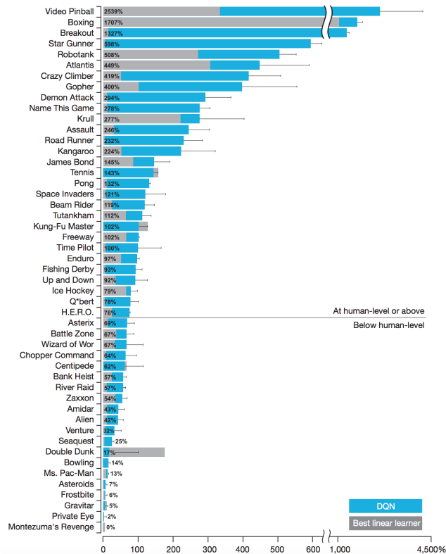
Figura 2.10: Resultados de la arquitectura DQN sobre 49 juegos testeados, presentados por Mnih et al. [29]. Se observa que para juegos con recompensa dispersa no se obtienen buenos resultados.
