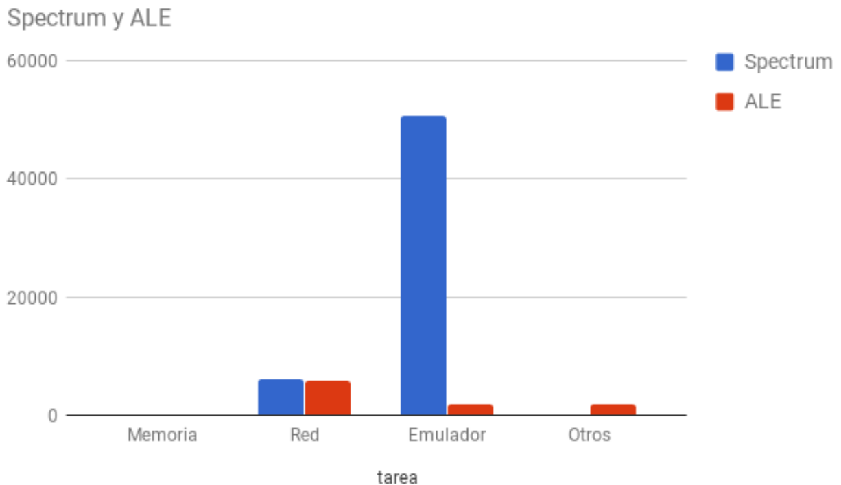
Figura 4.3: Para cada tarea se muestran los tiempos netos comparándolos entre ALE, en rojo, y Spectrum, en azul
