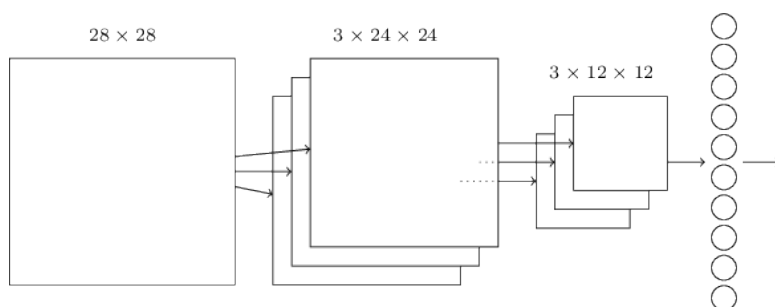
Figura 2.8: Esquema de la arquitectura convolutiva completa. Tomada del libro de Michael A. Nielsen [31].
