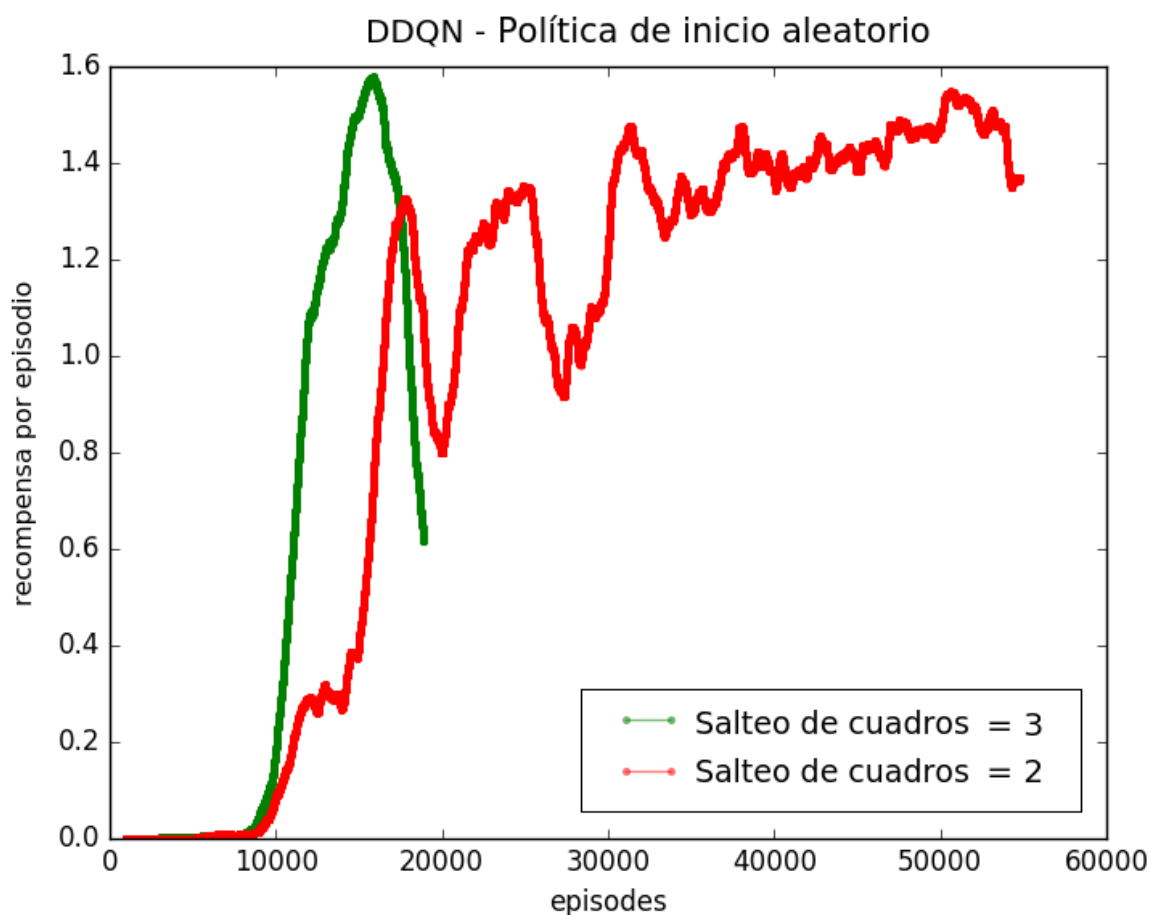
Figura 3.7: Recompensa en función de los episodios, con una media móvil de ventana tamaño 1000. Se corta la ejecución del agente con 3 cuadros de salteo debido a la abrupta caída en el desempeño. Para el salto de 2 cuadros, se observa la misma caída, sin embargo, como comienza a crecer se continúa su ejecución.
