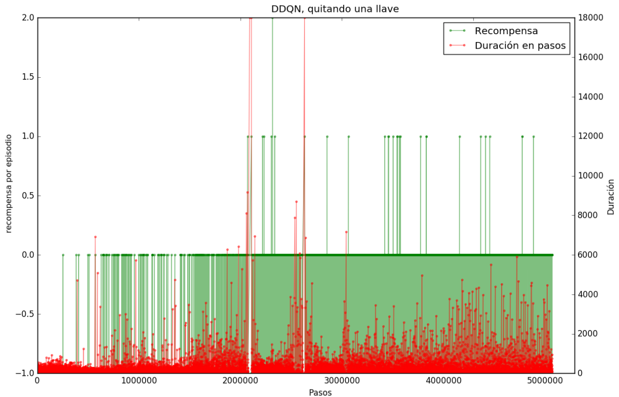
Figura 3.8: Recompensa obtenida y duración del episodio en pasos.
