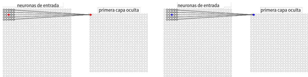
Figura 2.5: Estas figuras representan cómo se desplazan horizontalmente los campos receptivos locales. Análogamente se desplazan de forma vertical cubriendo así la totalidad de la imagen. Se puede interpretar la capa oculta como una nueva imagen donde cada uno de sus píxeles se corresponde con un píxel en la imagen original. Imágenes tomadas del libro de Michael A. Nielsen [31].
