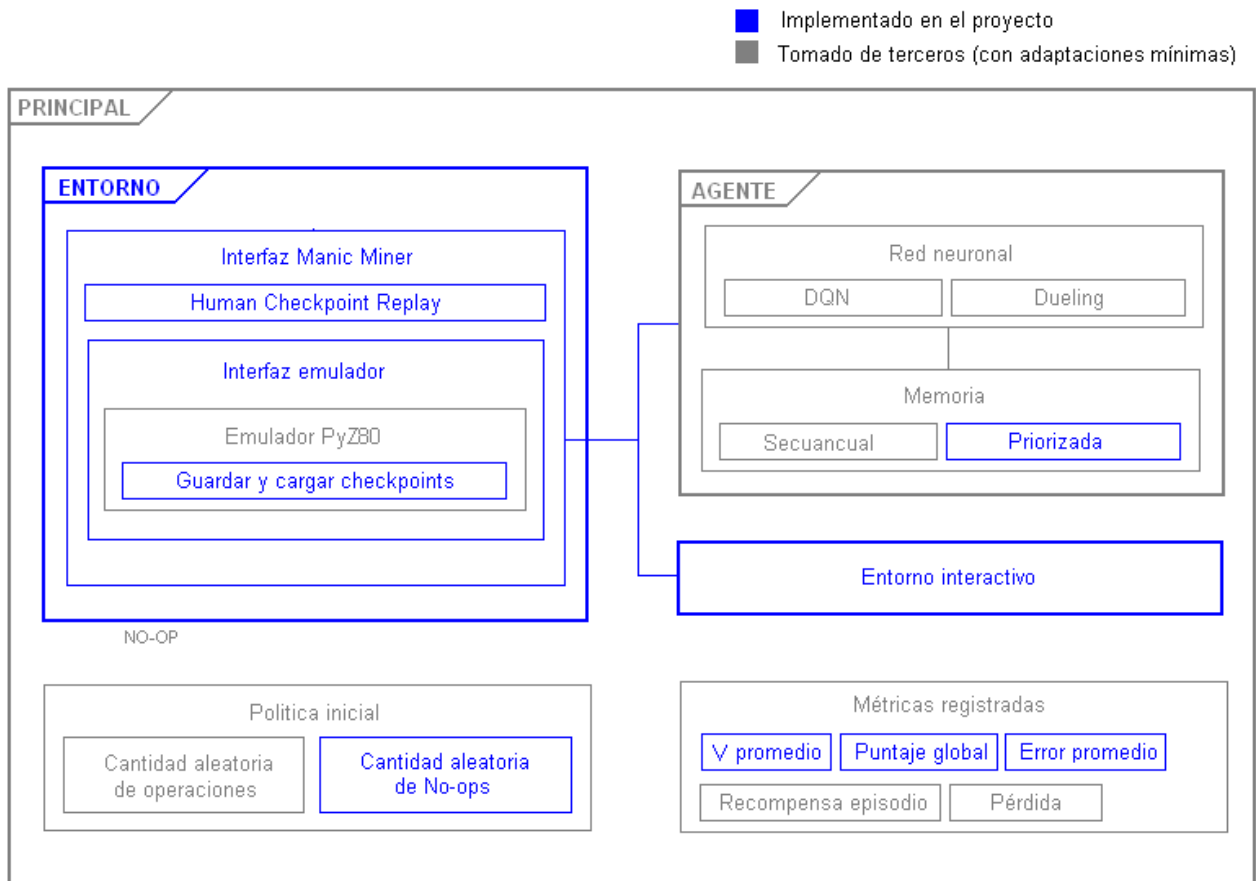
Figura 4.1: Estructura modularizada del entorno y agente. Cada componente está coloreado indicando si es desarrollado en el contexto de este proyecto o si es tomado de terceros.
