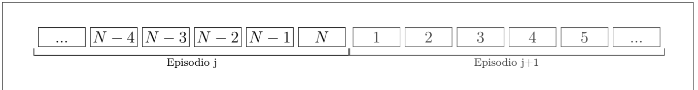
Cuadro 4.5: Segmento de memoria en la que se almacenan cuadros para dos episodios consecutivos, donde i contiene al último cuadro del i -ésimo episodio
