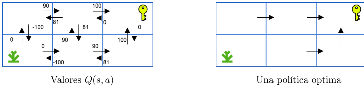
Figura 2.3: Se muestra la tabla de la función \hat{Q} luego de converger y una política óptima, correspondiente a las acciones con máximo valor \hat{Q} .
