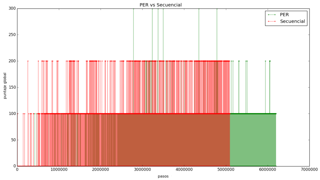
Figura 3.15: Puntaje para Dueling implementado con y sin PER
