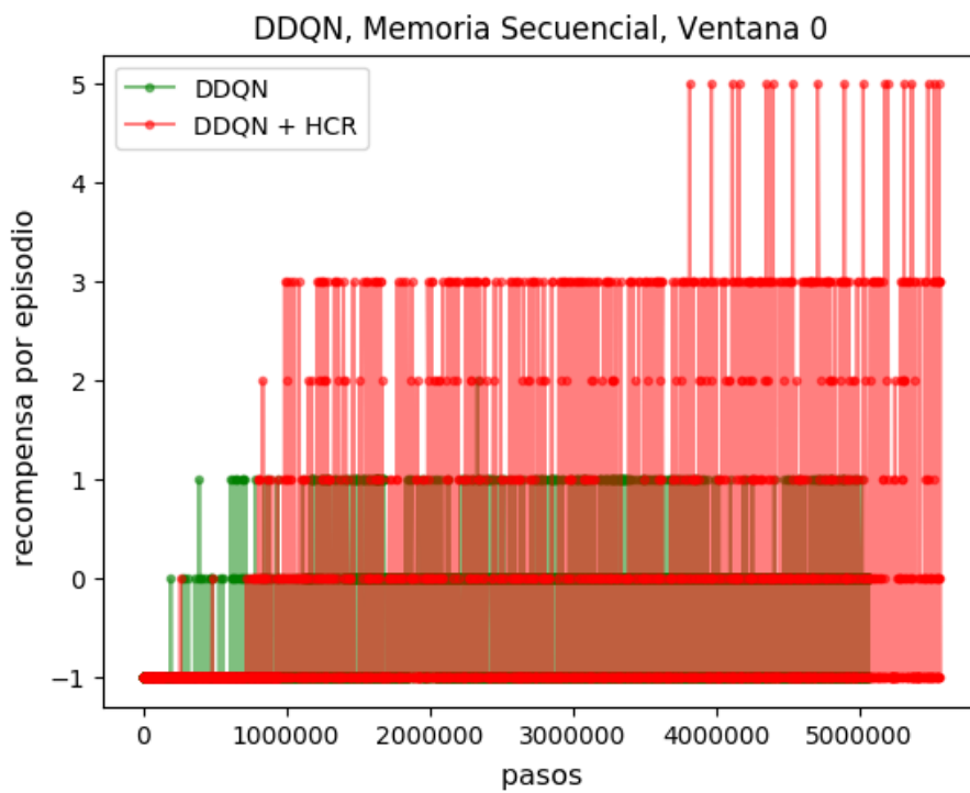
Figura 3.20: Recompensa con y sin HCR.
