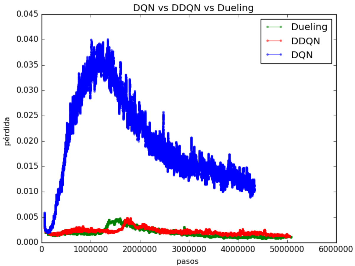
Figura 3.10: Función de pérdida para cada una de las tres arquitecturas consideradas. Se muestra la media móvil con ventana 50.
