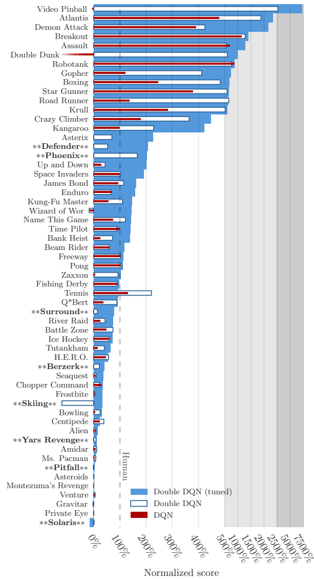
Figura 2.11: Resultados de la arquitectura DDQN presentado por Hasselt et al. [42]
