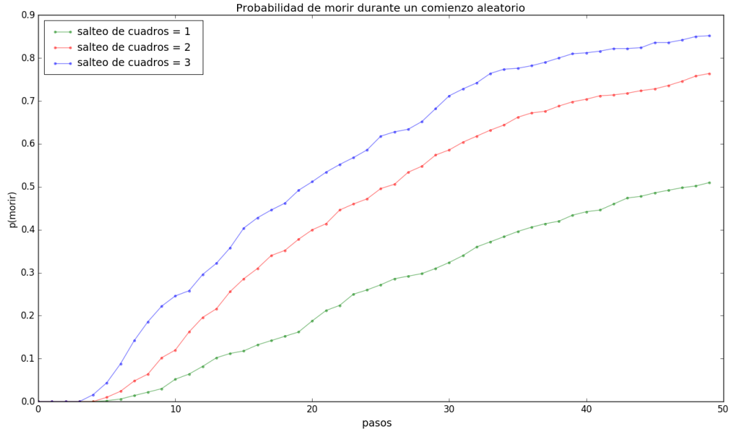
Figura 3.3: Probabilidad de morir en función de la cantidad máxima de movimientos aleatorios iniciales, M .
