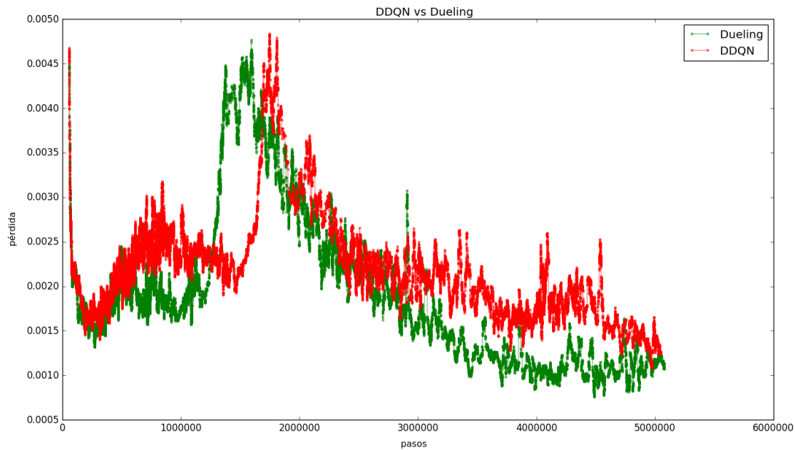
Figura 3.11: Función de pérdida para DDQN y Dueling. Se muestra la media móvil con ventana 50.
