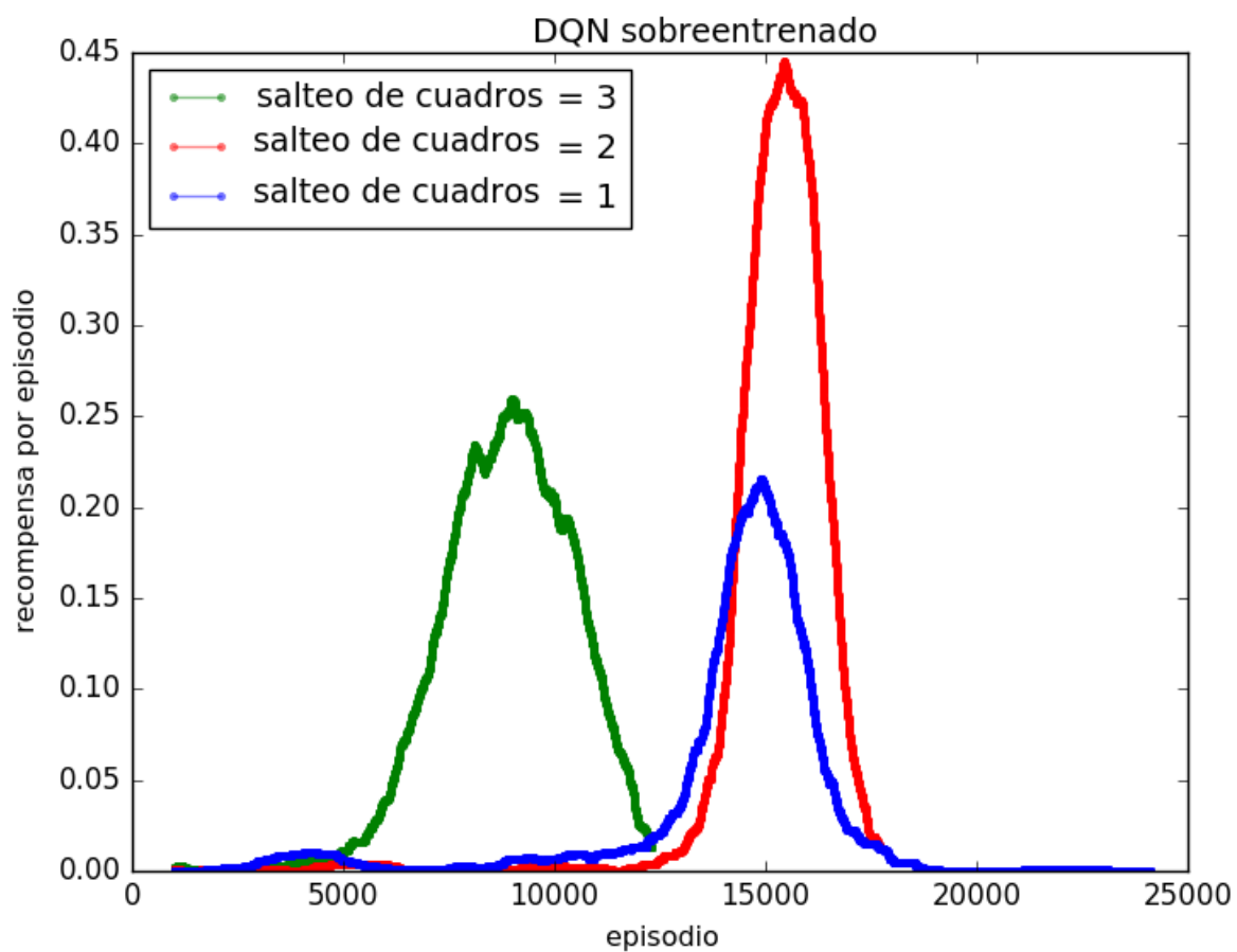
Figura 3.6: Recompensa en función de los episodios, con una media móvil de ventana 1000. Se observa que saltando de a 3 cuadros el aprendizaje comienza antes, mientras que saltando de a 2 se alcanza el mayor valor.
