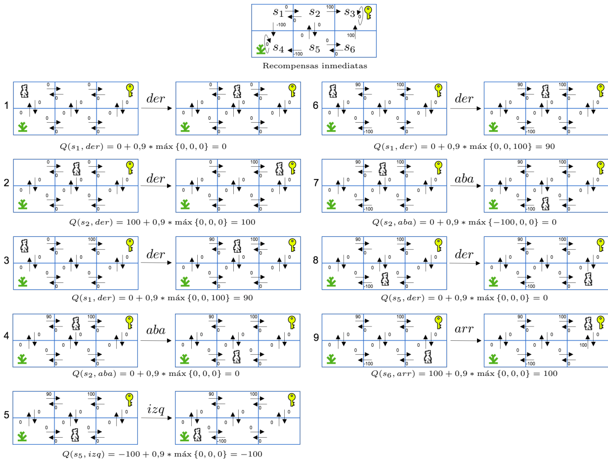
Figura 2.2: Ejemplo simple para ilustrar los conceptos básicos de aprendizaje por refuerzos. Cada entrada de la tabla representa un estado distinto y cada flecha una acción. Se muestra la función de recompensa inmediata y los cambios en la tabla \hat{Q} producidos por cada una de las acciones usando un factor de descuento de 0,9.
