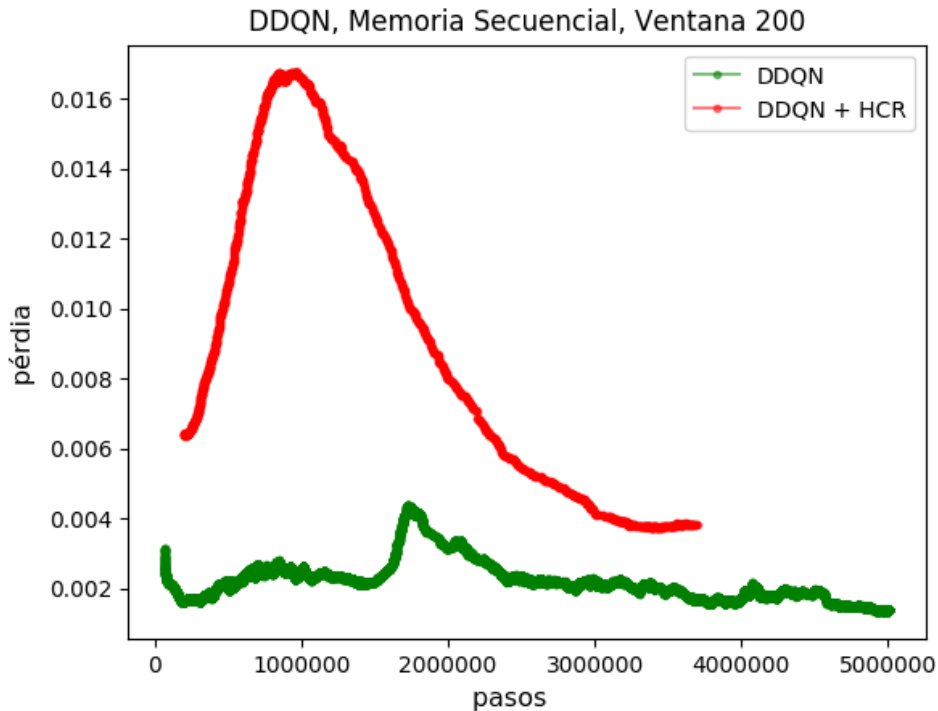
Figura 3.18: Pérdida con y sin HCR.
