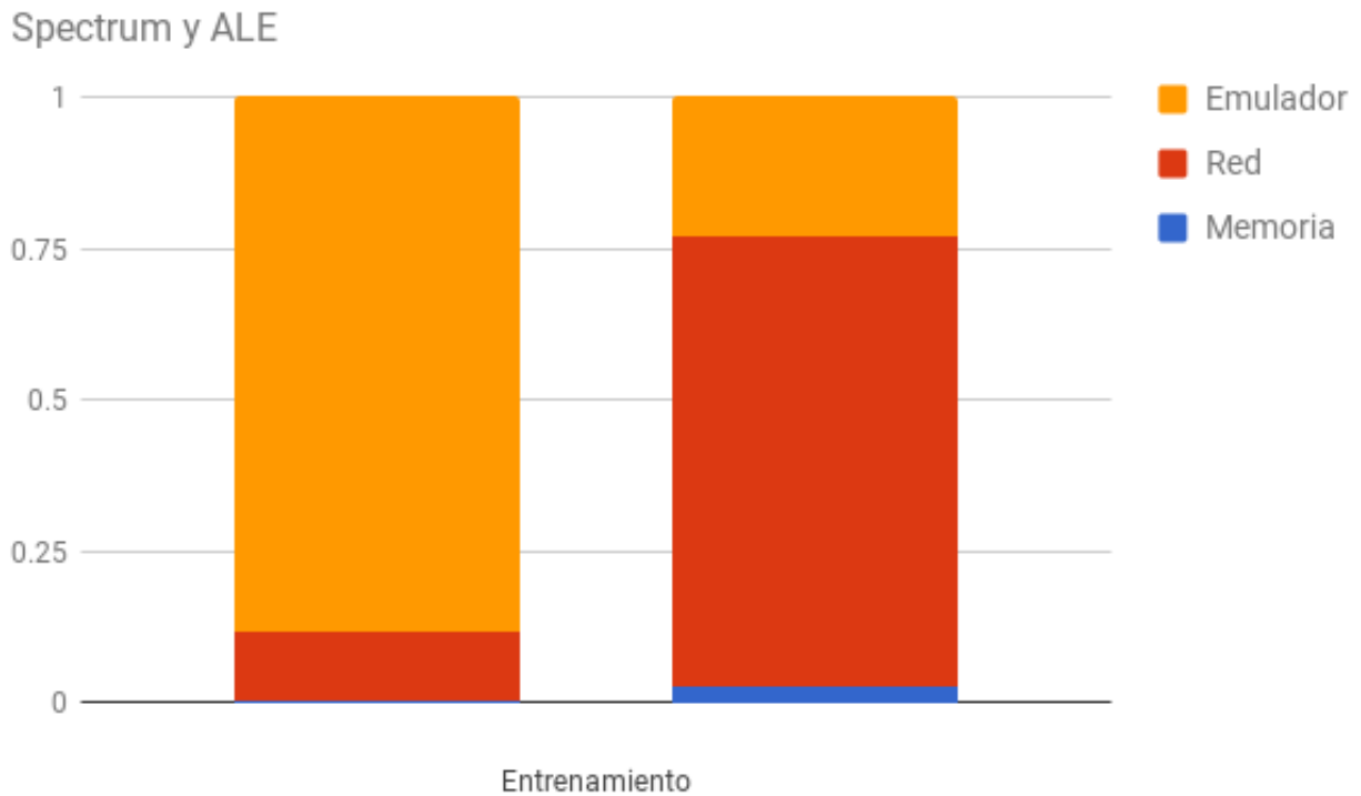
Figura 4.2: Se muestran los tiempos para cada emulador durante el entrenamiento. Los tiempos totales se encuentran discriminados proporcionalmente por tareas. La barra de la izquierda corresponde a ZX Spectrum mientras la de la derecha, a ALE.
