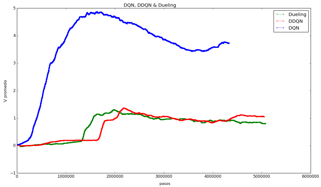
Figura 3.12: V promedio para cada una de las arquitecturas. Se muestra la media móvil con ventana 50.
