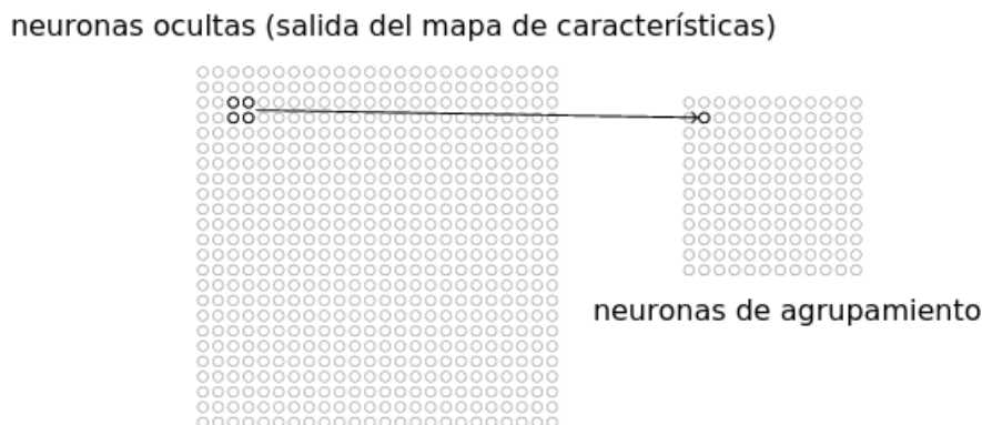
Figura 2.6: Capa de agrupamiento: la información de cuatro neuronas se condensa en una sola. Tomada del libro de Michael A. Nielsen [31].
