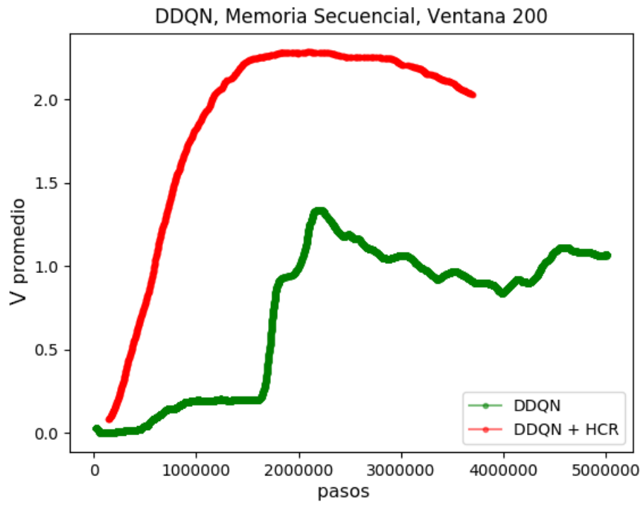
Figura 3.19: Recompensa con y sin HCR.
