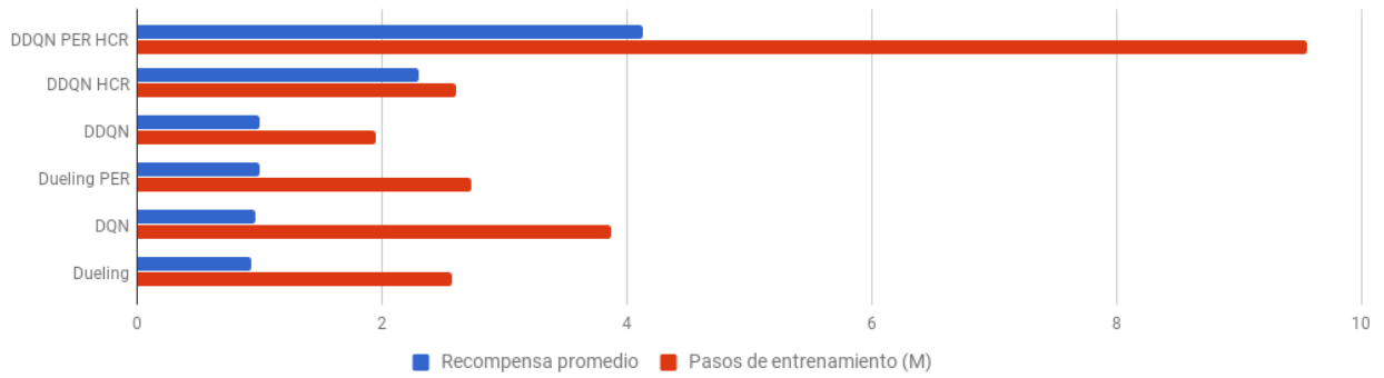
Figura 3.22: Recompensa promedio y pasos de entrenamiento.
