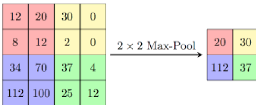
Figura 2.7: Unidad max pooling aplicada con 2 de stride a regiones de 2 \times 2 . Se reducen los parámetros en un 75% pasando de 16 a 4.
