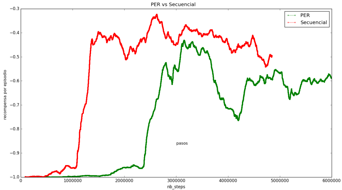
Figura 3.14: Recompensa para Dueling implementado con y sin PER, con media móvil tamaño 1000
