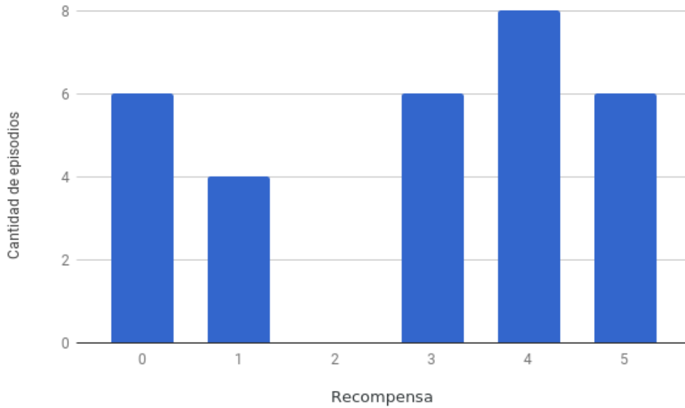
Figura 3.21: Histograma con HCR . Cantidad de episodios agregados según recompensa obtenida. No hay ocurrencias con recompensa en -1 debido a que todas las ejecuciones toman al menos una llave.
