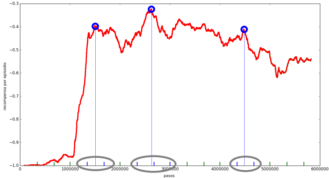
Figura 3.4: Para elegir los pesos prometedores se consideran aquellos que fueron almacenados en momentos cercanos a donde se alcanzan máximos locales durante el entrenamiento. Este ejemplo ilustrativo muestra la función de recompensa por episodio, los círculos azules señalan los máximos locales escogidos. Las marcas en el eje x, separados por cada 250 mil pasos, representan los puntos del entrenamiento en donde se realiza un respaldo de los pesos de la red. La cantidad de máximos locales elegidos y el tamaño de la ventana son aleatorios y dependen de la cantidad de puntos del entrenamientos que se desean evaluar.
