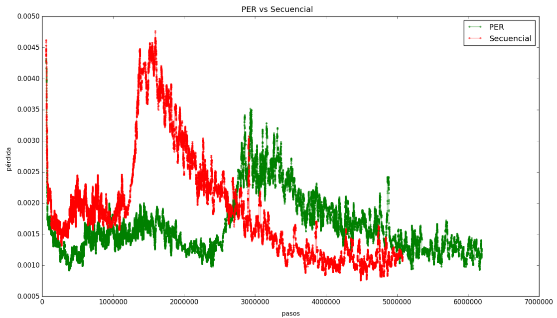
Figura 3.16: Pérdida para Dueling implementado con y sin PER.
