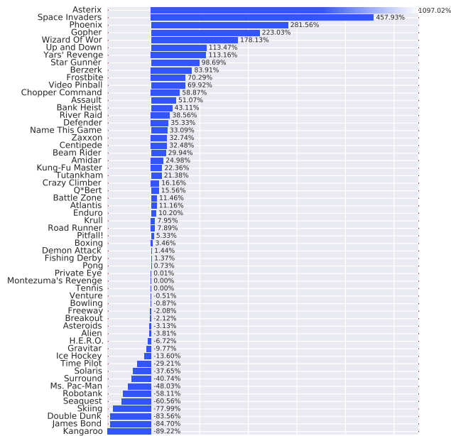
Figura 2.13: Resultados de la arquitectura Dueling reportados por van Hasselt [43]
