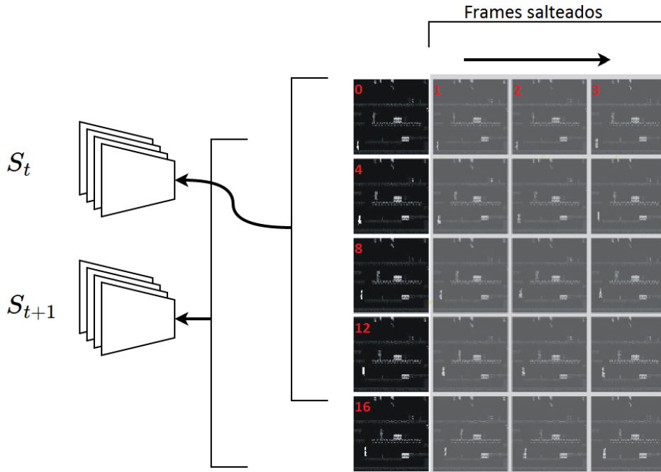
Figura 2.4: Los cuadros opacos no forman parte de la entrada para el agente. Se ejemplifican dos estados consecutivos; se observa que entre un estado y el siguiente hay una superposición de m - 1 cuadros.
