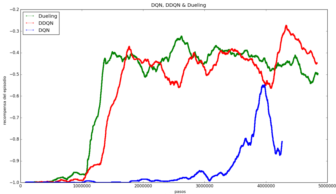
Figura 3.9: Recompensas por episodio para cada una de las tres arquitecturas consideradas. Se utiliza una ventana de tamaño 1000.
