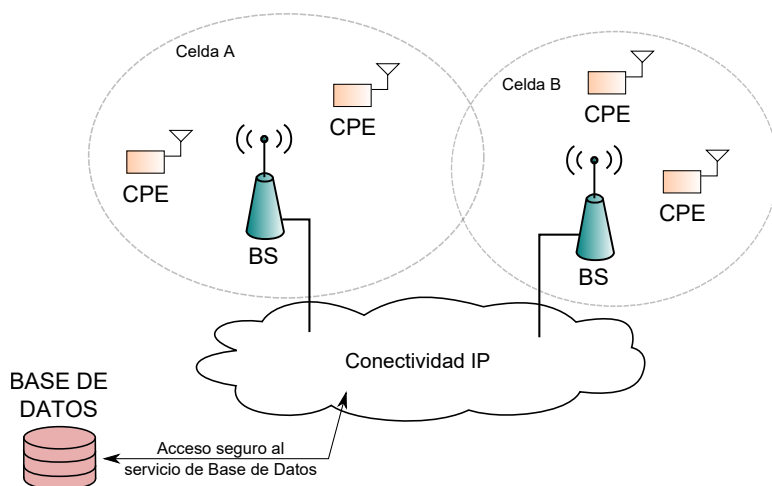
Figura 5.6: Topología de red IEEE 802.22 10 .
