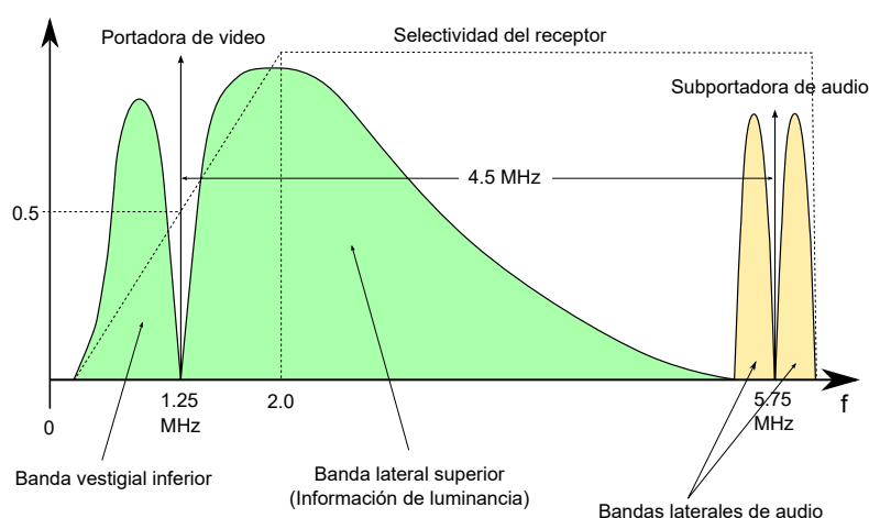
Figura H.1: Uso del espectro para un canal de televisión analógica 6 .
