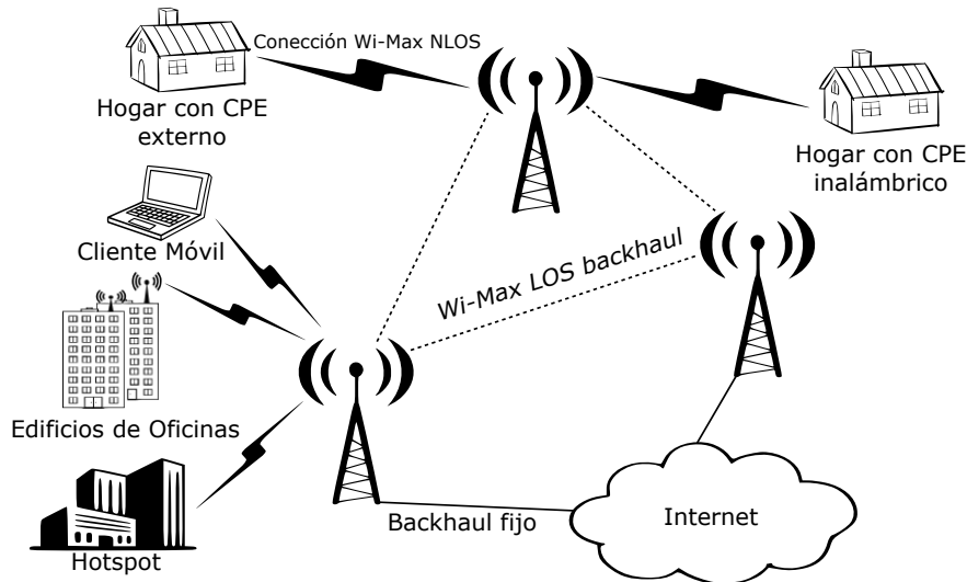
Figura 5.12: Topología de red IEEE 802.16 [35].
