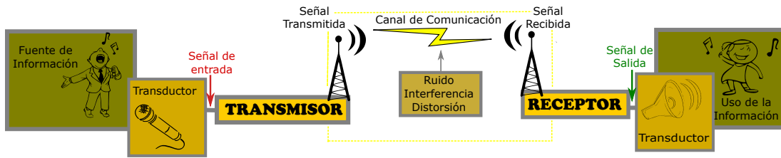
Figura A.12: Esquema de un sistema de comunicación simplificado 17 .
