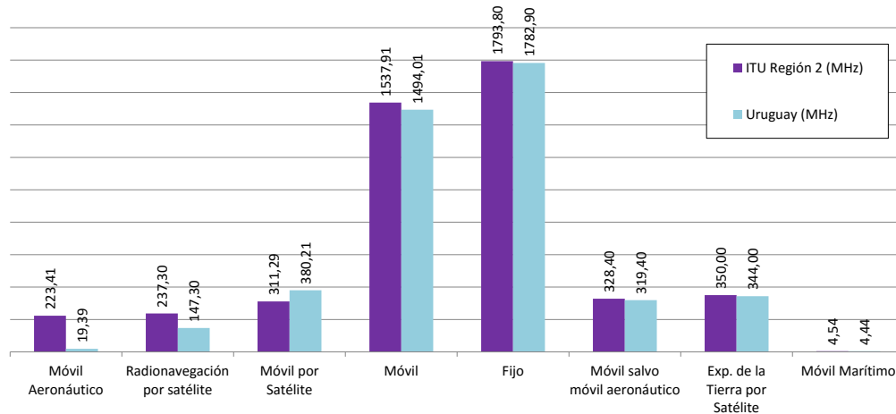
Figura 3.3: Cuadro comparativo entre atribución por servicio de UIT y URSEC.
