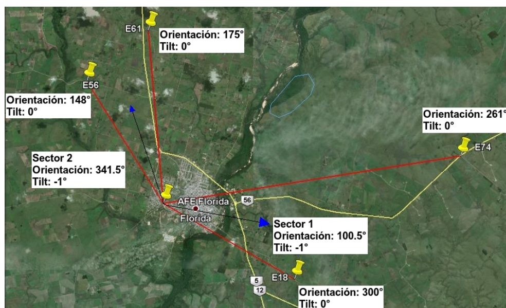
Figura 5.18: Ubicación geográfica de los puntos a comunicar en Florida (Uruguay), en el piloto TVWS de Ceibal 26 .
