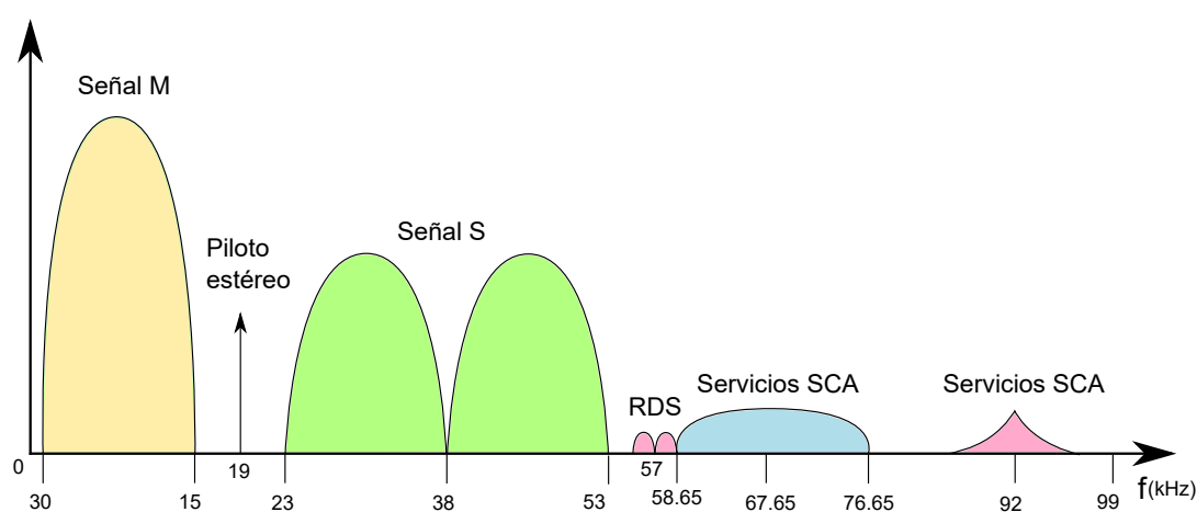
Figura H.2: Uso del espectro para un canal de FM.
