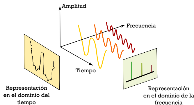
Figura A.7: Representación de una señal en el tiempo y en la frecuencia 5 .
