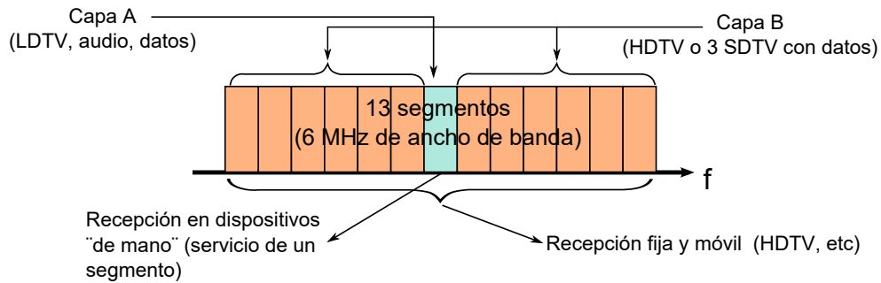
Figura H.3: Canal segmentado ISDB-T 12 .
