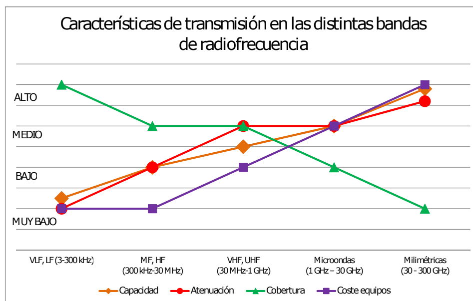
Figura 2.2: Características bandas de radiofrecuencia 6 .
