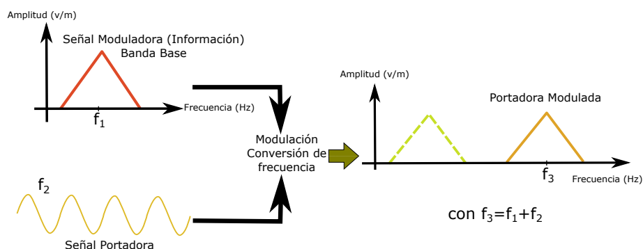
Figura A.14: Esquema de modulación por conversión de frecuencia 20 .
