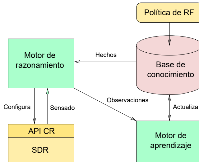
Figura 5.3: Diagrama funcional de un CR, representando sus capacidades de razonamiento y aprendizaje [68].
