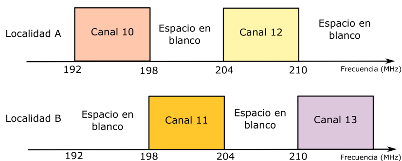
Figura 5.2: Espacios en blanco entre canales de TV 3 .
