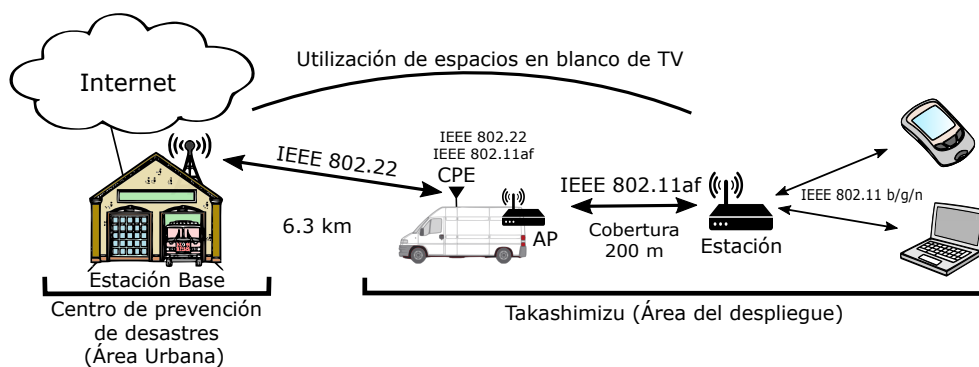
Figura 5.17: Esquema de red multi-salto implementada con estándares IEEE [39].
