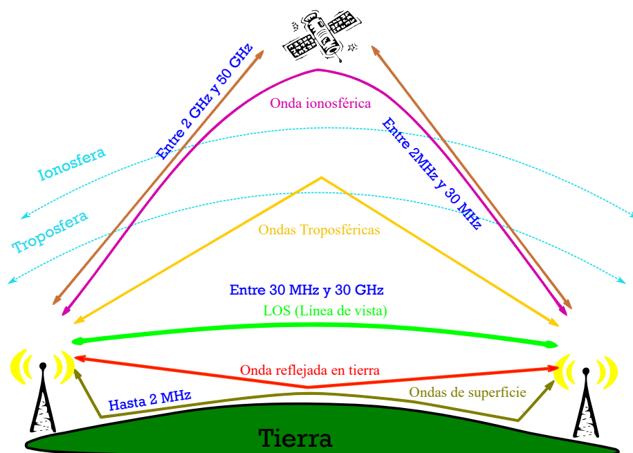
Figura A.11: Mecanismos de propagación de una onda 14 .
