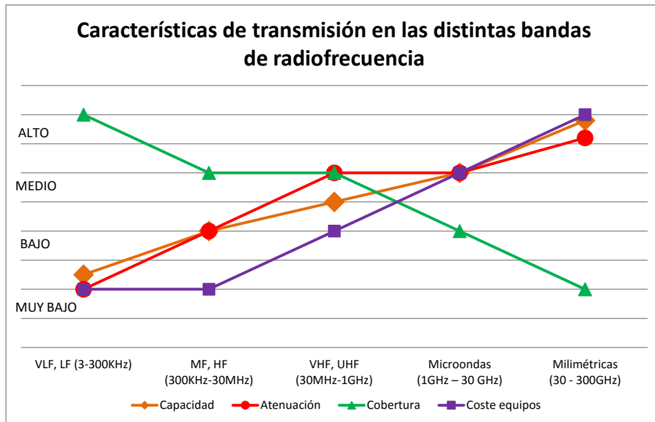
Figura A.10: Características bandas de radiofrecuencia.
