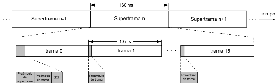
Figura 5.10: Estructura general de supertrama [29].
