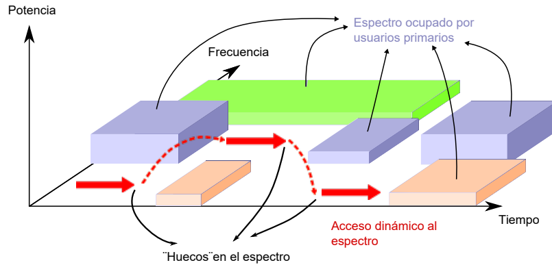
Figura 5.1: Representación del DSA en los espacios en blanco del ERE 2 .
