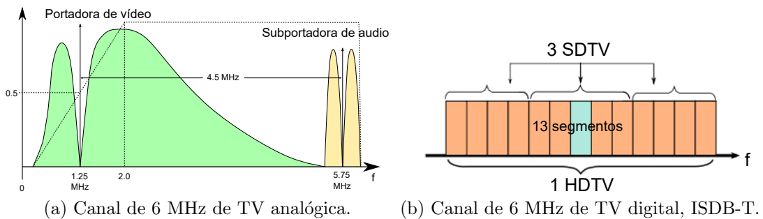
Figura 3.4: Comparación de uso del ERE para diferentes sistemas de TV.
