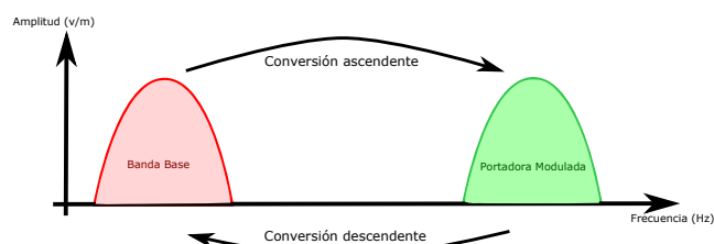
Figura A.13: Conversión de frecuencia.
