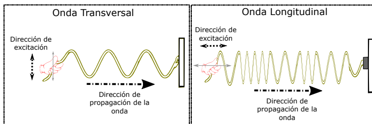
Figura A.2: Onda longitudinal y onda transversal 3 .
