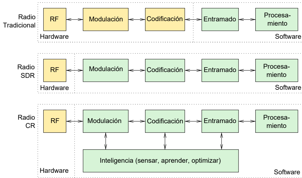
Figura 5.4: Comparación funcional de los distintos tipos de equipos de RF [68].
