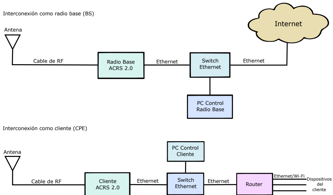
Figura 5.20: Interconexiones.
