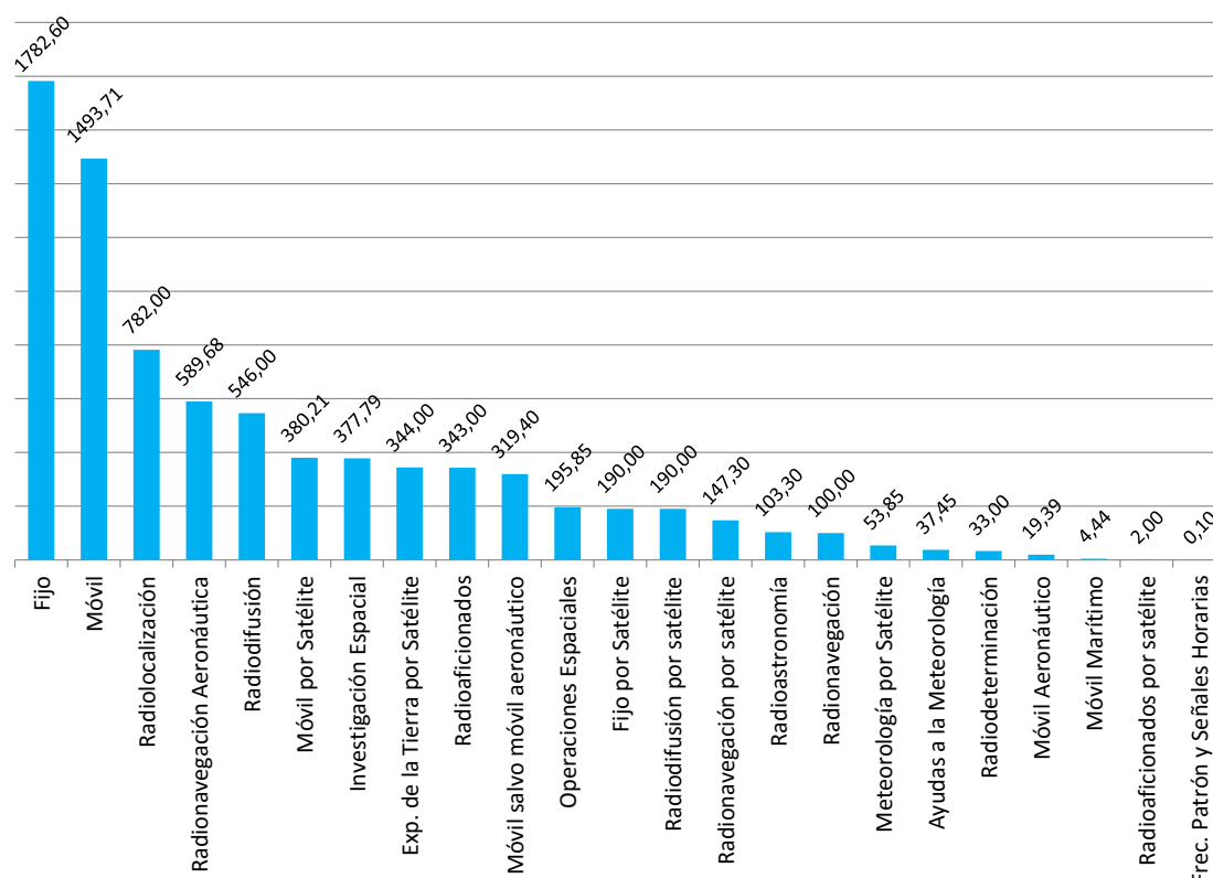
Figura 3.2: Cantidad de espectro atribuido por servicio en Uruguay (MHz).
