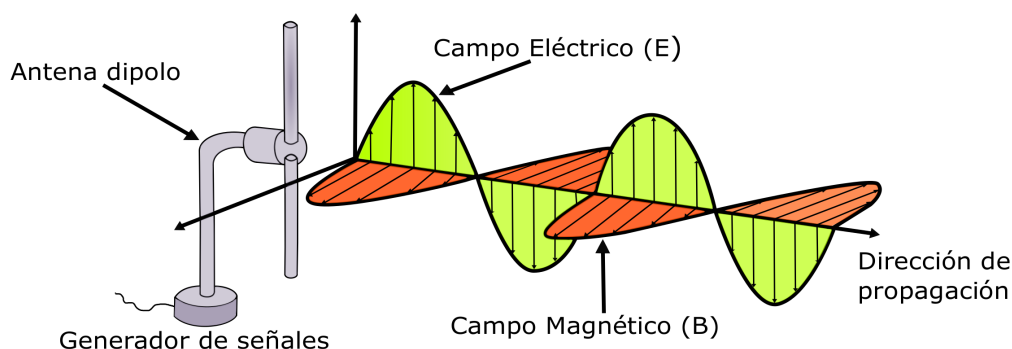
Figura A.8: Onda electromagnética 6 .
