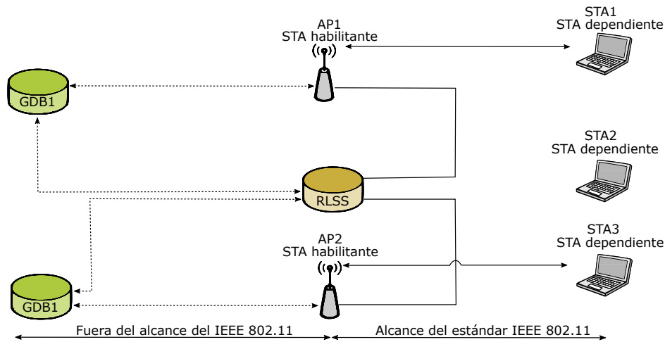
Figura 5.11: Topología de red IEEE 802.11af [32].
