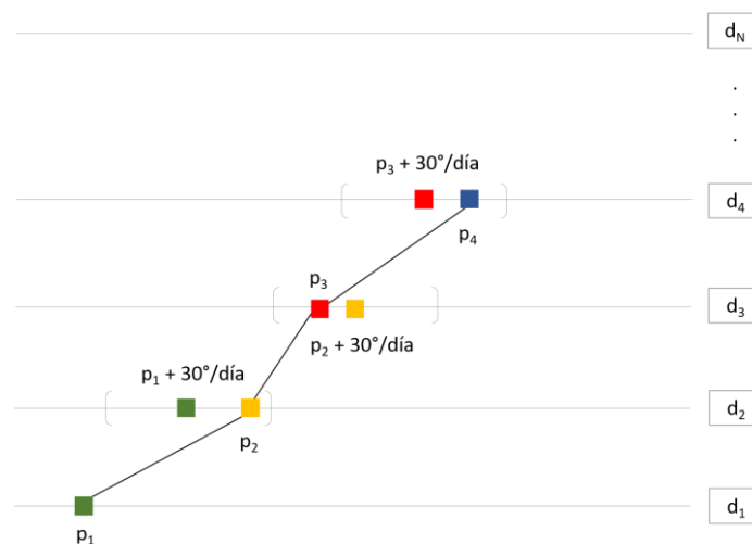
Figura 4: Esquema del funcionamiento del algoritmo de rastreo. p_1 , p_2 , p_3 y p_4 son las posiciones de los máximos en los niveles 1,2,3 y 4 respectivamente. Cada nivel representa un día de la temporada considerada para el rastreo.
